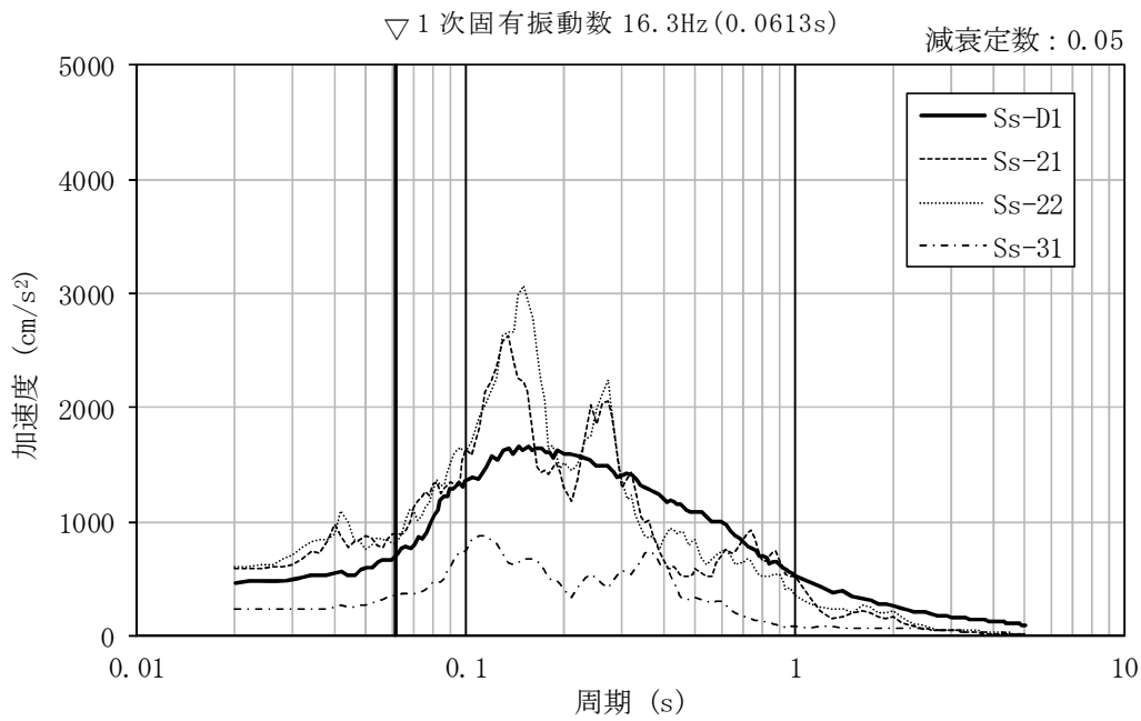
図 4-2 評価対象が位置する質点での床応答スペクトル (質点番号 7, S_s , +\sigma ケース, 鉛直方向)
