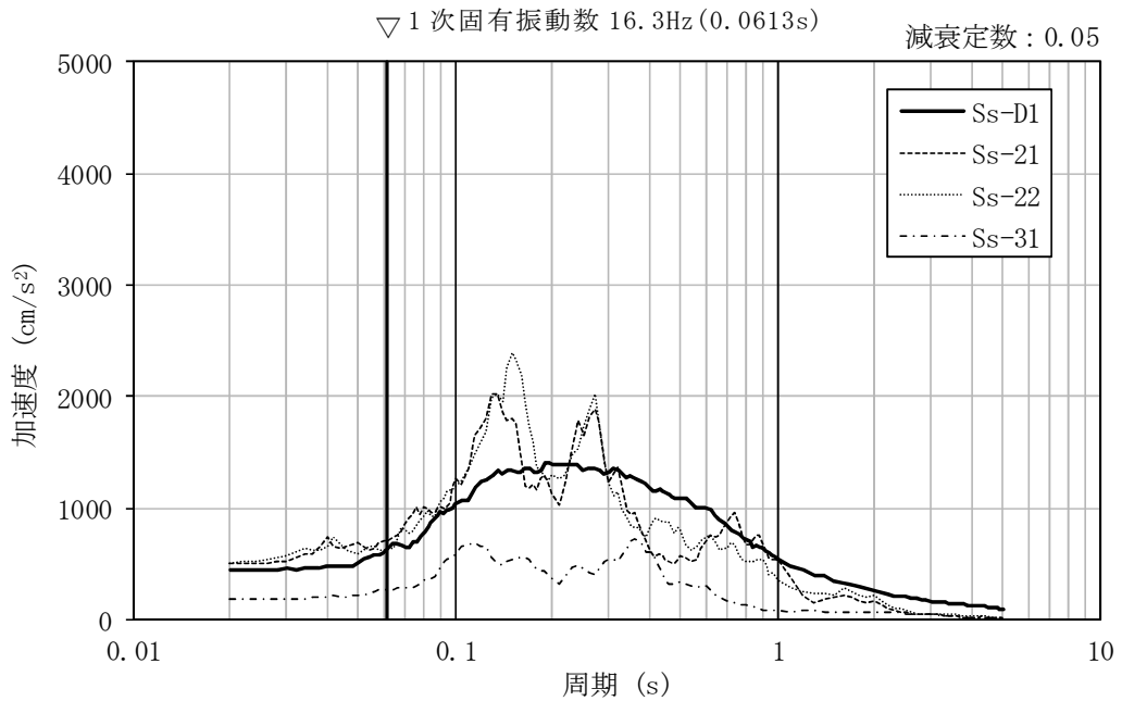
図 4-3 評価対象が位置する質点での床応答スペクトル (質点番号 7, S_s , -\sigma ケース, 鉛直方向)
