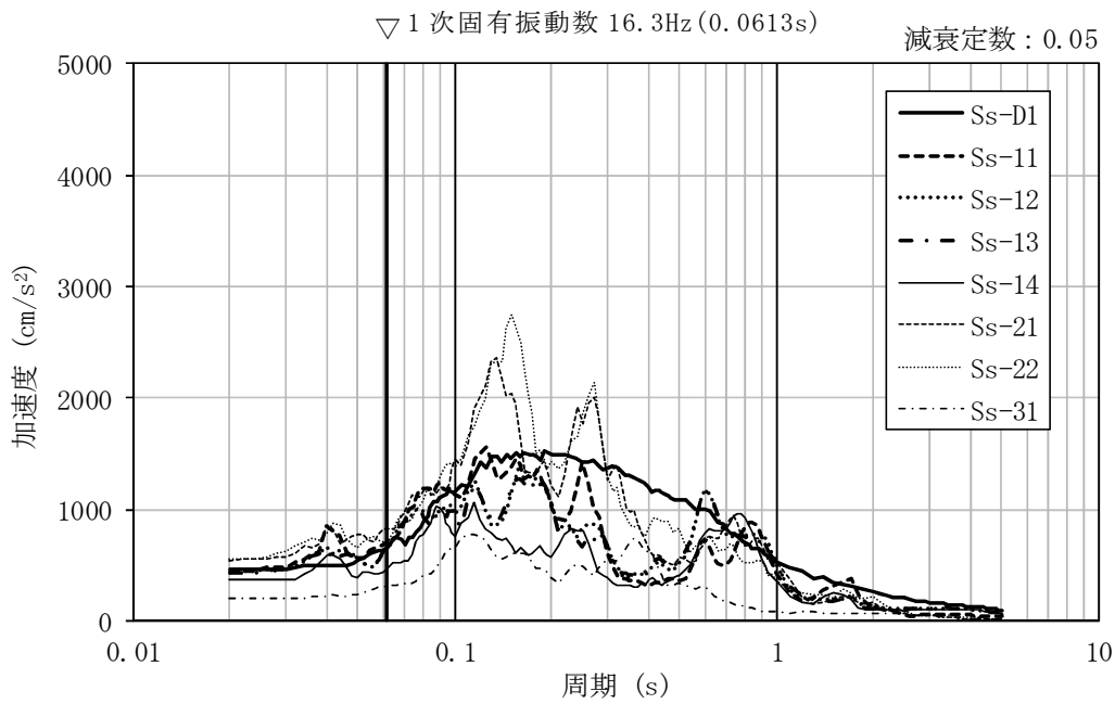
図 4-1 評価対象が位置する質点での床応答スペクトル (質点番号 7, S_s , 基本ケース, 鉛直方向)
