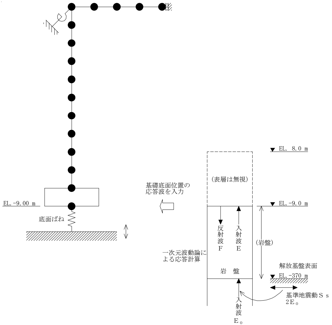
図 3-20 地震応答解析モデルに入力する地震動の概念図 (UD 方向)
