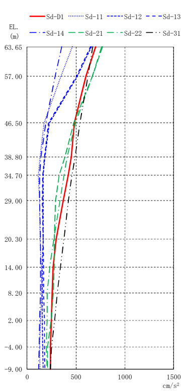
圖 4-18 最大応答加速度 (S d , NS 方向)
