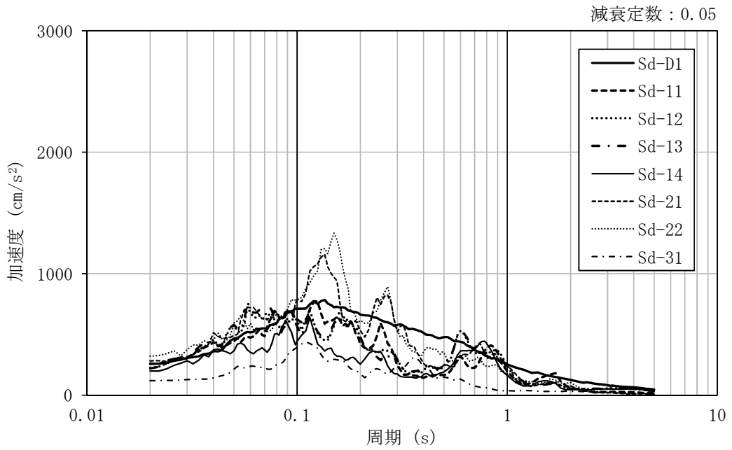
図 3-22 入力地震動の加速度応答スペクトル ( S_d , UD 方向, EL. -9.0 m)
