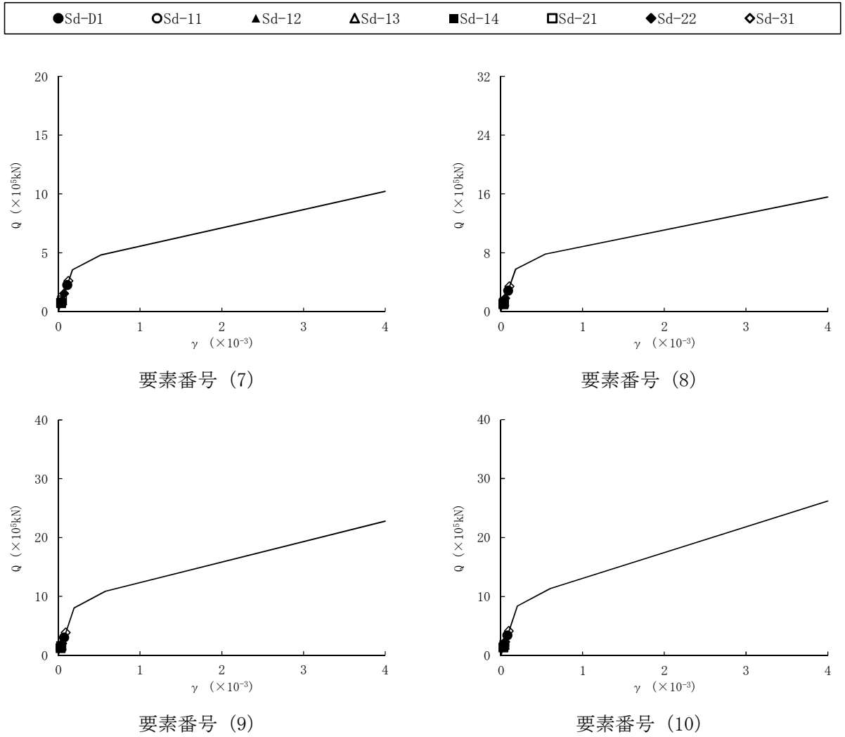
図 4-30 (2/2) せん断スケルトンカーブ上の最大応答値 (S d , EW 方向)
