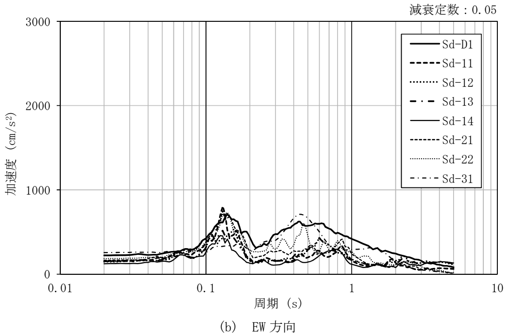
図 3-19 入力地震動の加速度応答スペクトル ( S_d , EL. -9.0 m)
