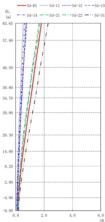
圖 4-19 最大応答変位 (S d , NS 方向)
