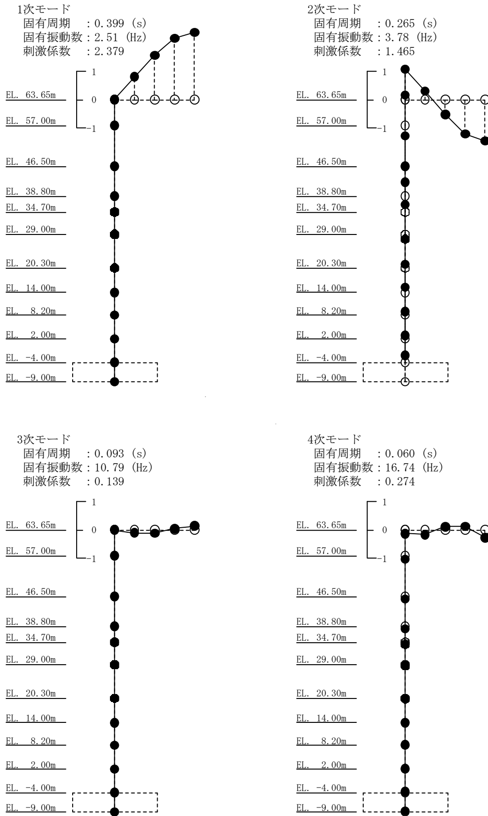
図 4-2 (3/3) 刺激関数図 (S d -D 1, UD 方向)
