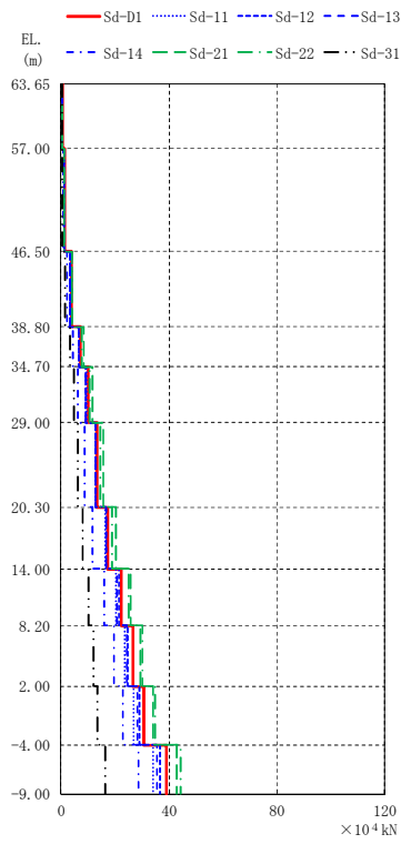
图 4-28 最大応答軸力 (S d , UD 方向)
