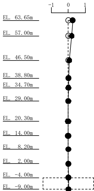
図 4-2 (2/3) 刺激関数図 (S d -D 1, EW 方向)
