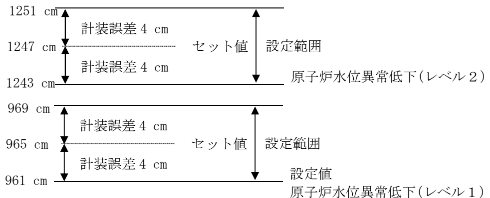
原子炉水位異常低下（レベル1）設定値の概要図
