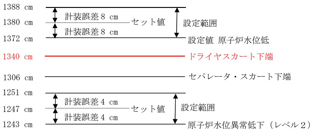
原子炉水位低設定値の概要図
