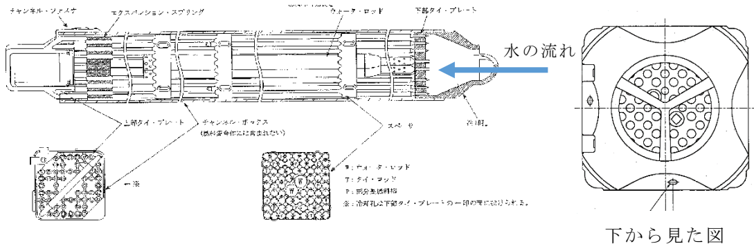
図2 燃料集合体下部タイプレート（9×9燃料（A型）の例）
