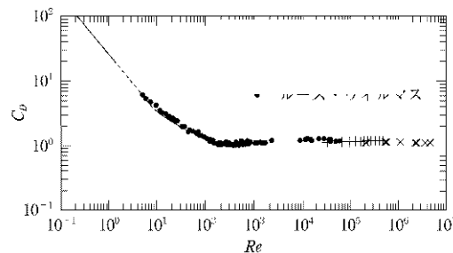
図 5 円板の抗力係数
