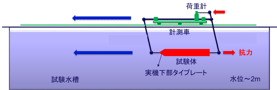
図8 抵抗力係数測定試験イメージ
