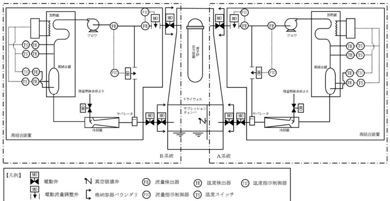
第 2-1 図 可燃性ガス濃度制御系の系統概略図
