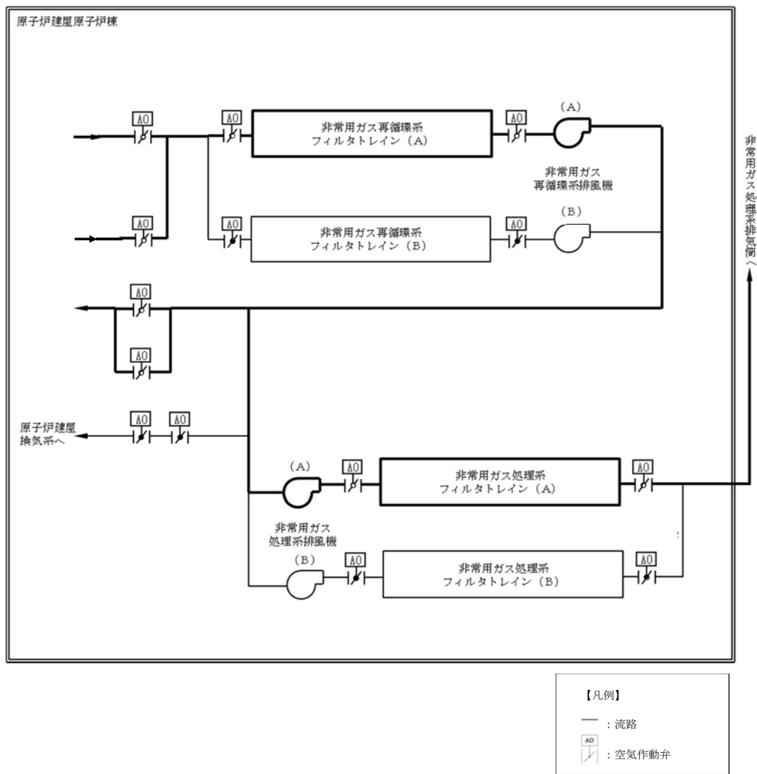
第2-5図 原子炉建屋ガス処理系 系統概略図
