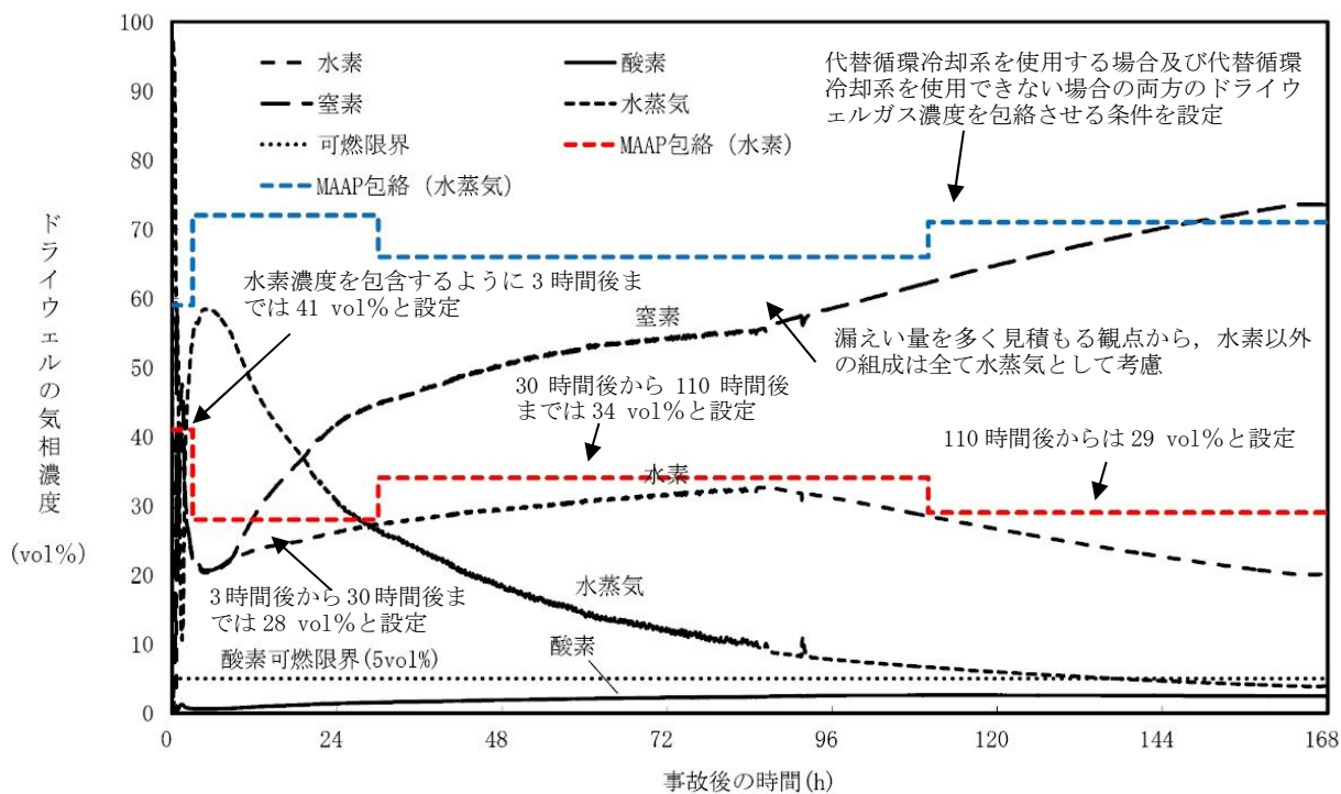
第 2.3.1-6 図 ドライウエルガス濃度 (有効性評価シナリオ包絡条件) (代替循環冷却系を使用する場合)
