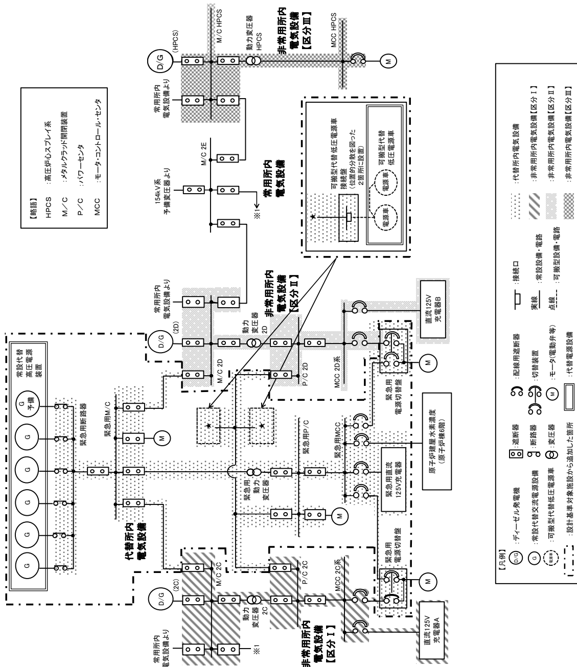
第2.4-5図 単線結線図 (交流電源設備)
