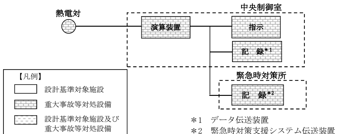
第4図 PAR動作監視装置の概略構成図
