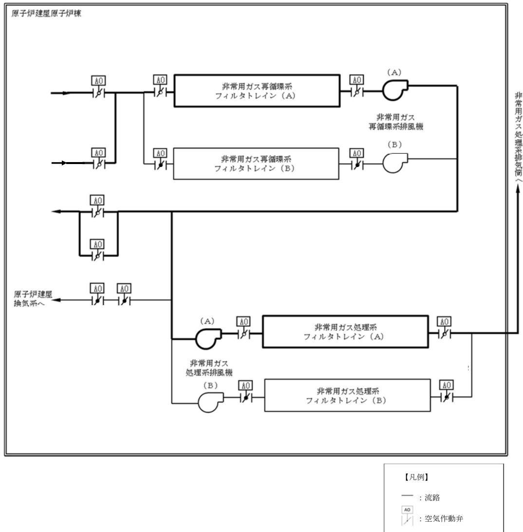
第2.2.1-1図 原子炉建屋ガス処理系 系統概略図
