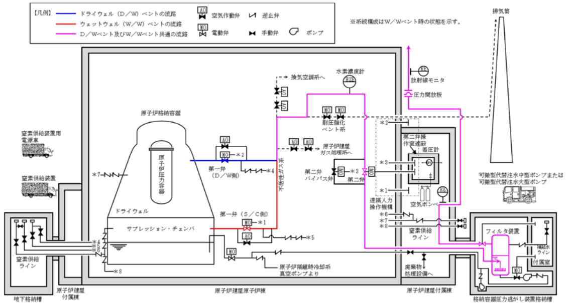
第 2-3 図 格納容器圧力逃がし装置の系統概略図
