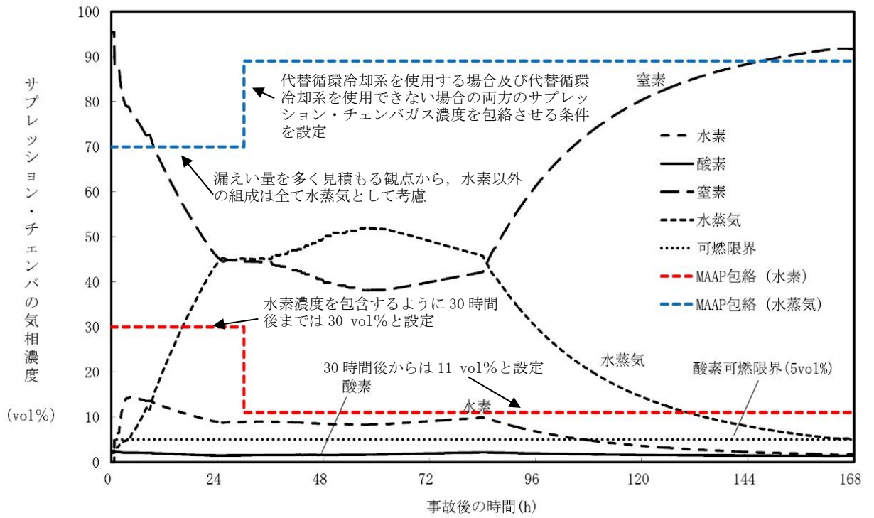
第 2. 3. 1-8 図 サプレッション・チェンバガス濃度 (有効性評価シナリオ包絡条件) (代替循環冷却系を使用する場合)
