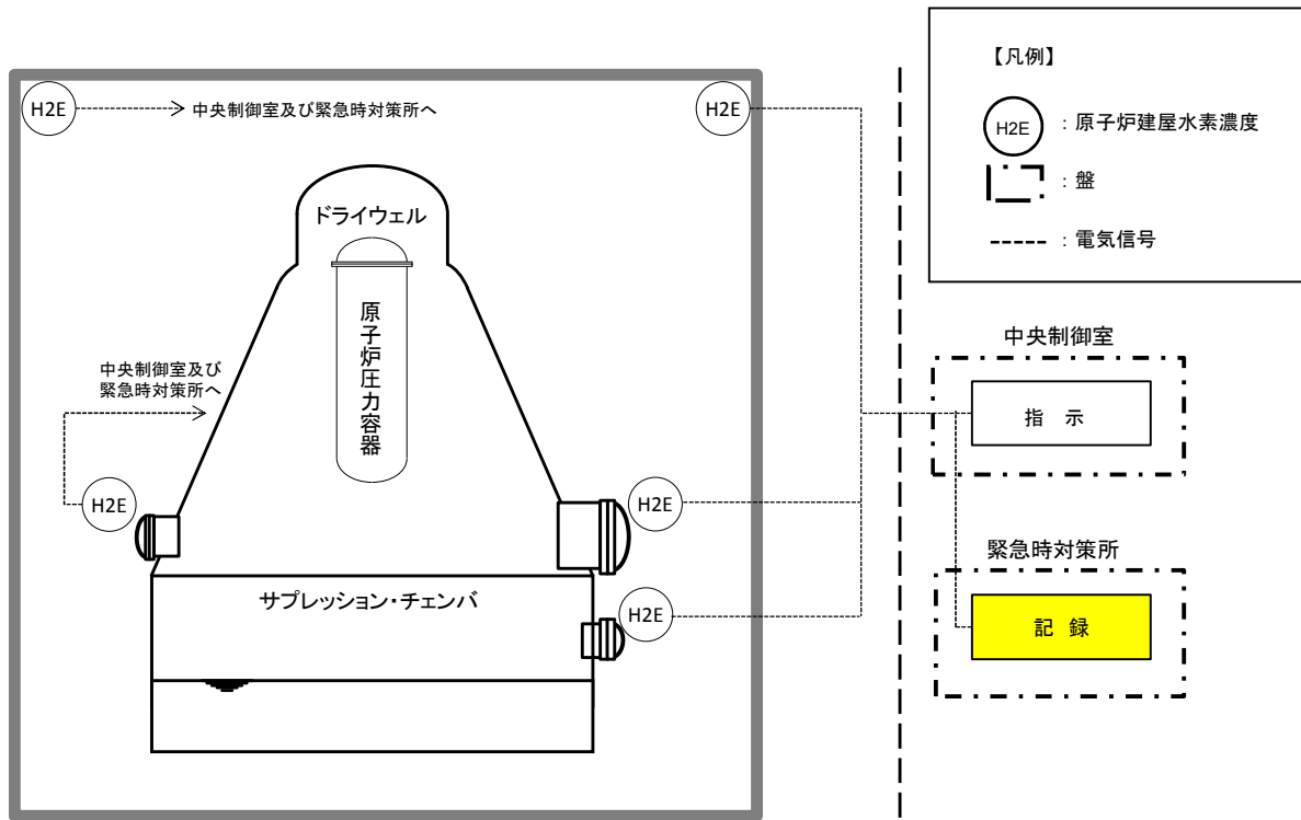
第 2-7 図 原子炉建屋水素濃度の系統概要図
