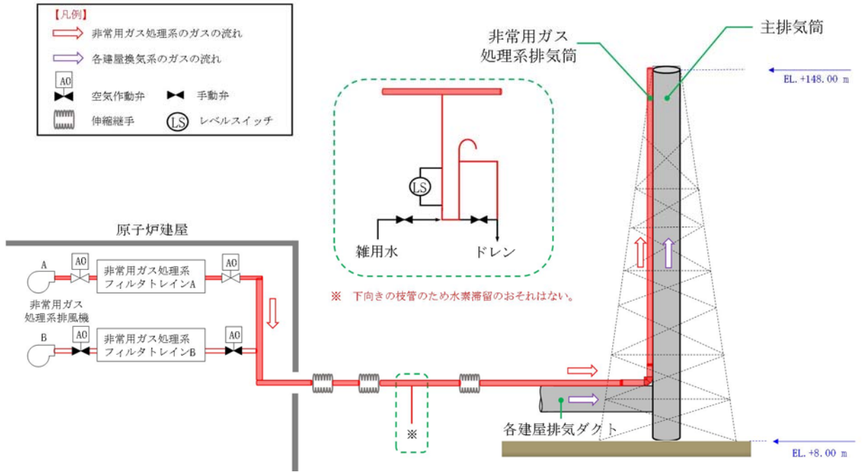
第 2. 2. 1-2 図 排気筒及び非常用ガス処理系排気筒の位置関係
