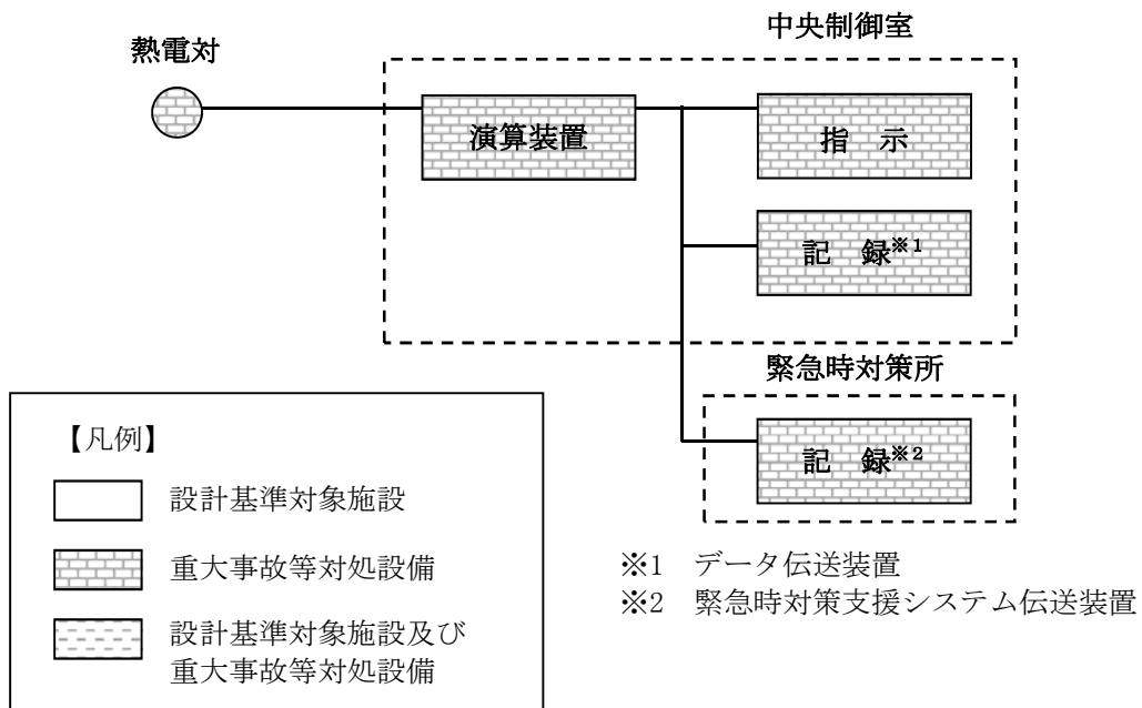
第4-5図 静的触媒式水素再結合器動作監視装置の概略構成図
