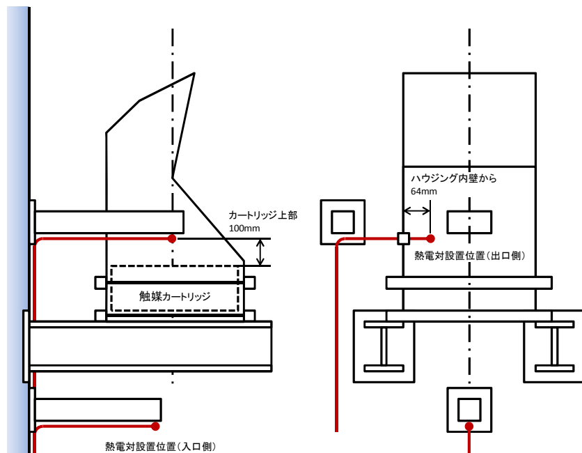
第4-6図 静的触媒式水素再結合器への熱電対取付位置概要図
