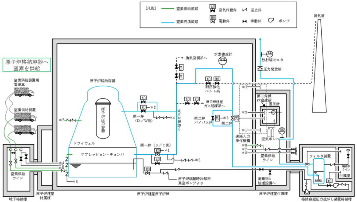
第 2-2 図 窒素供給装置の系統概略図
