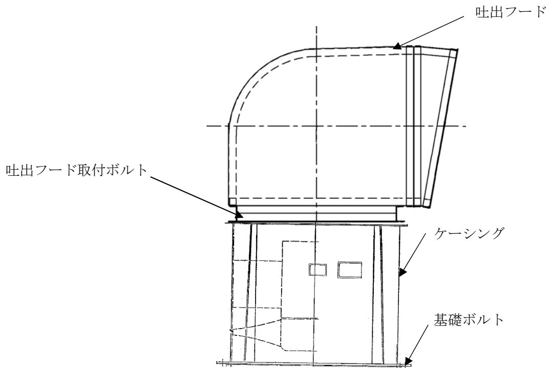
図 2-2 ディーゼル発電機室ルーフトファンの概要図
