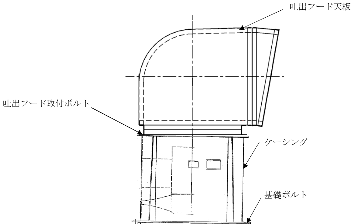
図 3-1 ディーゼル発電機室ルーフベントファンの評価対象部位
