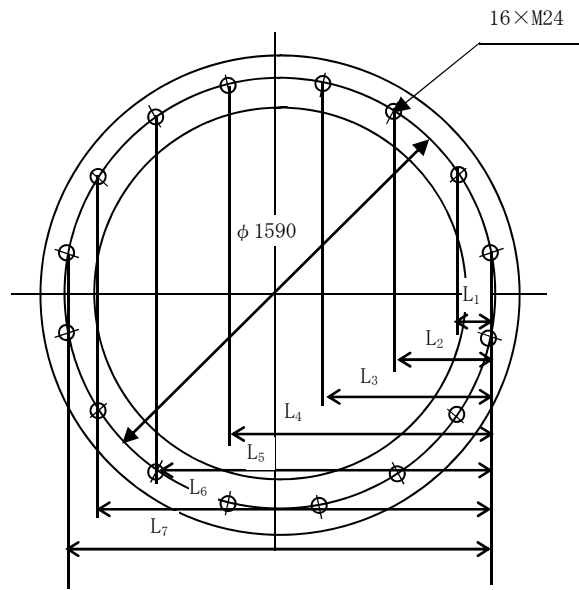
図 3-4 基礎ボルト配置図
