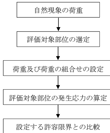
図2-2 ディーゼル発電機室ルーフベントファンの強度評価フロー
