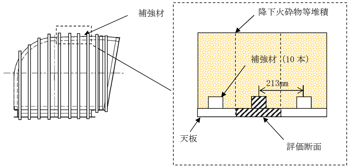
図 3-6 吐出フード天板部評価断面概要
