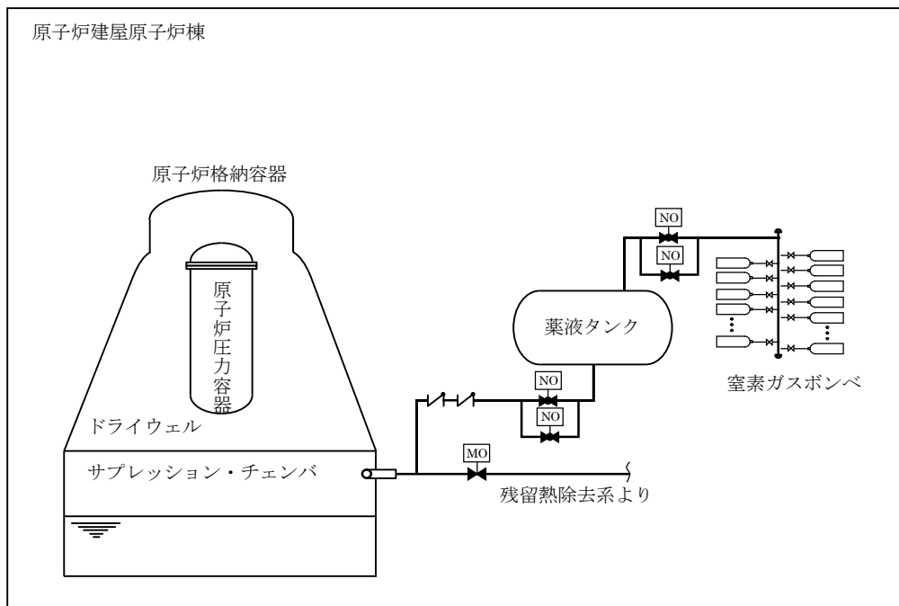
第 1 図 原子炉格納容器 pH 制御のための設備 系統概要図
