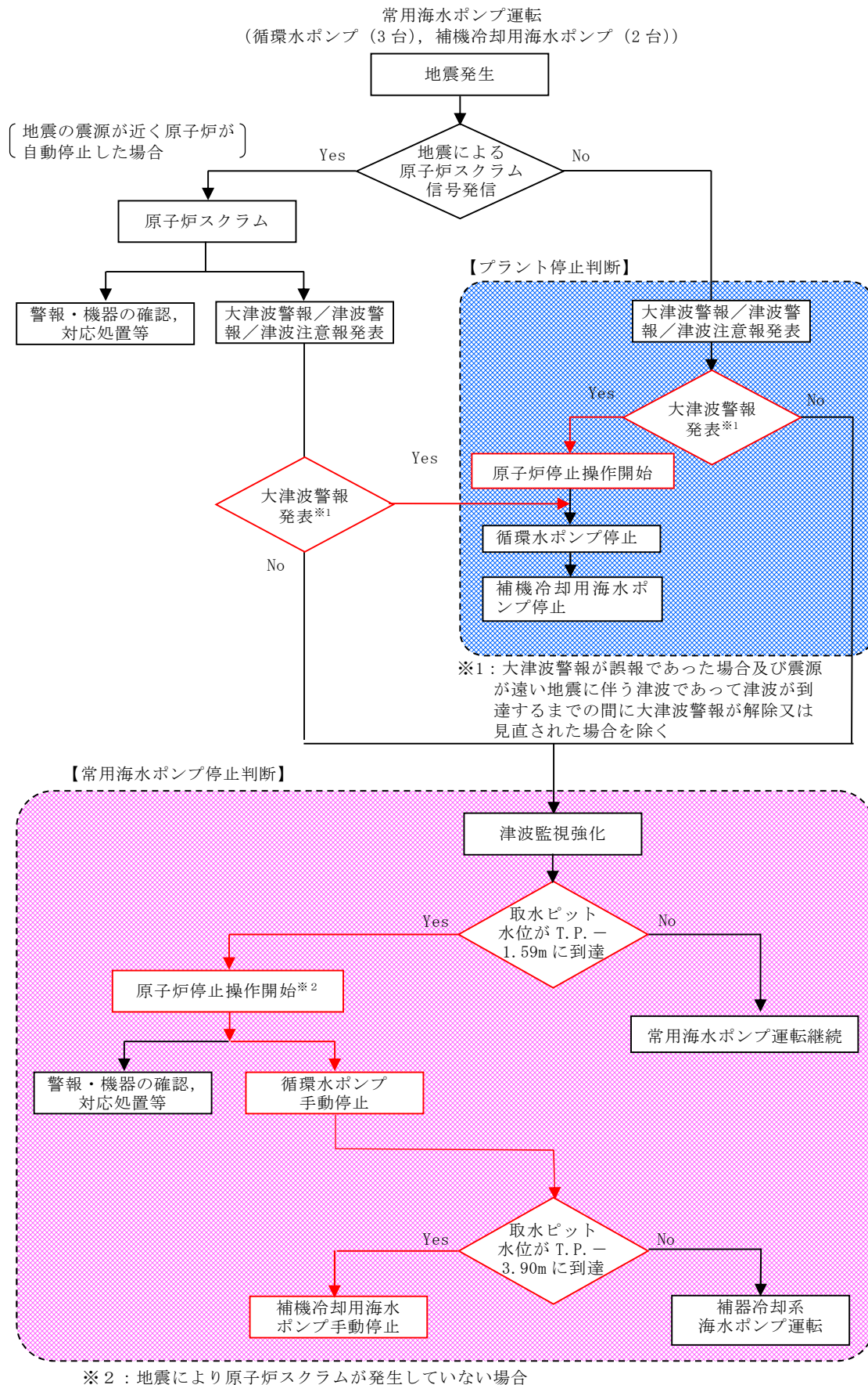
第1図 常用海水ポンプ停止フロー 5条 添付10-3
