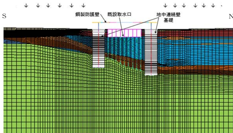
D 断面
