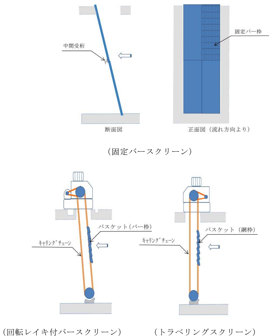
図 2.5-33 除塵装置概略構造
