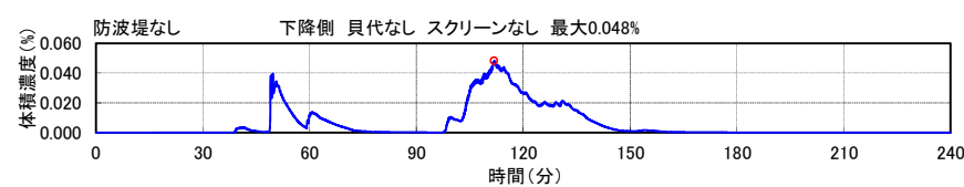
第5図 浮遊砂濃度時刻歴グラフ
