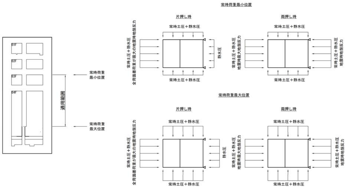
図 5-2 水平断面解析モデル概念図（開口部がない構造部）
