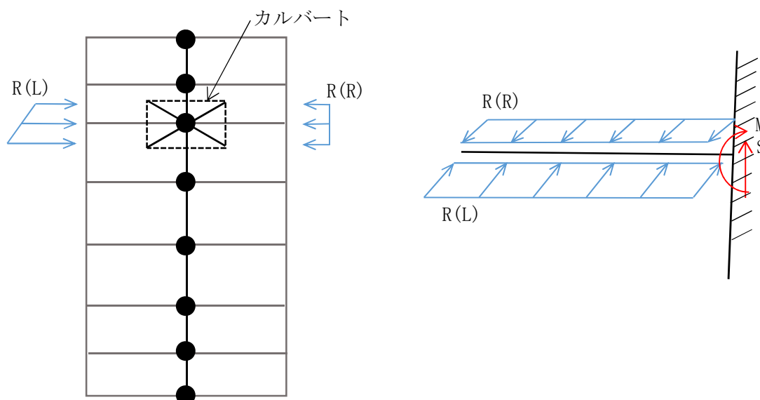
図 10-3 カルバート延長方向水平曲げに対する設計モデル概念図
