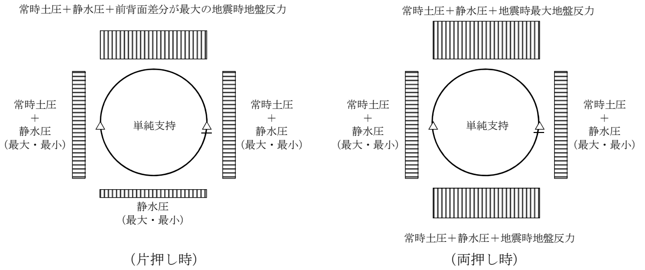
図 5-1 円形立坑の水平断面解析モデル概念図
