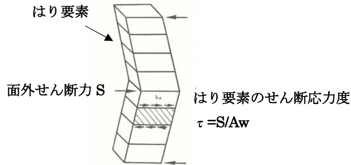
図 4-1 はり要素のせん断変形概念図
