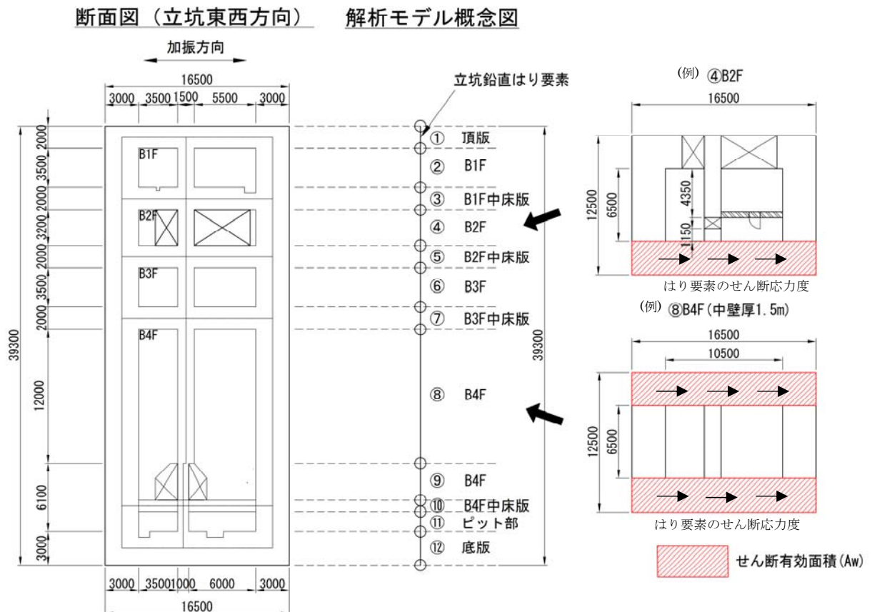
図 4-3 立坑を線形はり要素でモデル化した場合の概念図
