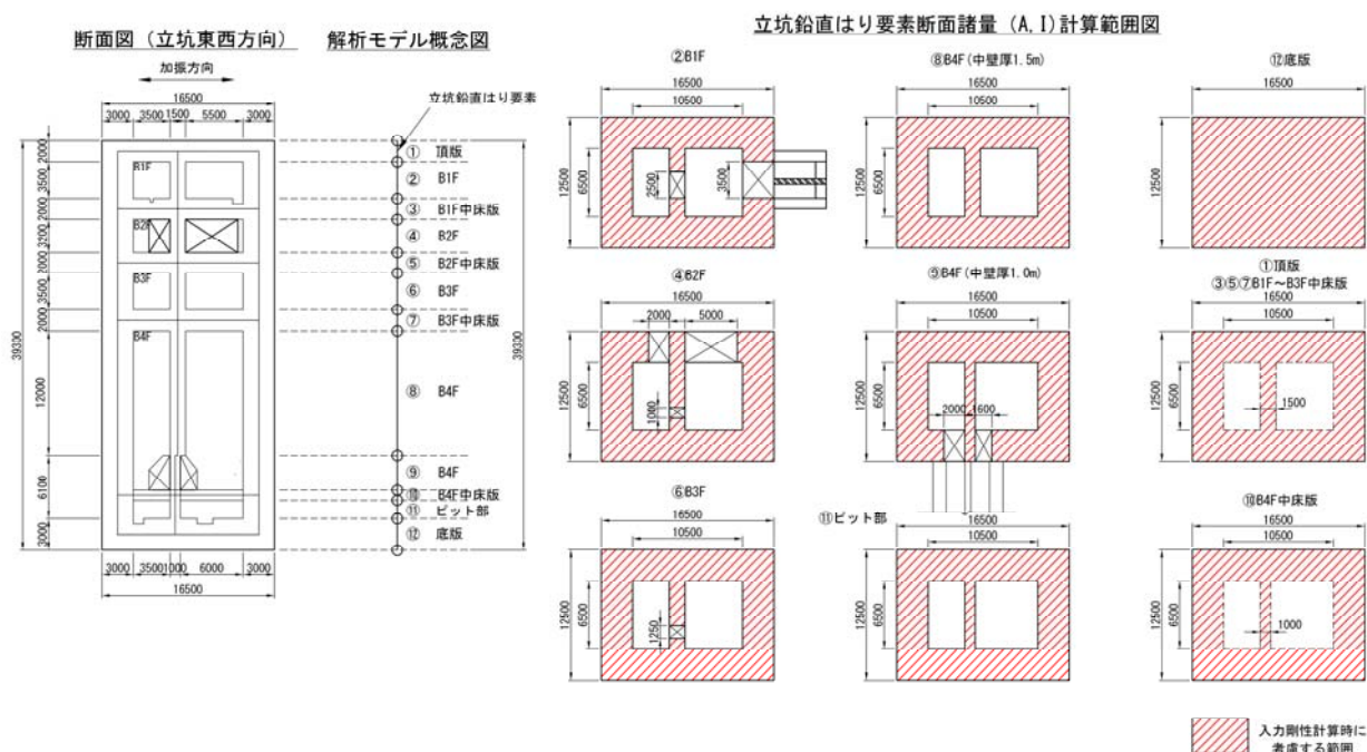
図 3-4 立坑構造物（線形はり要素）の入力剛性設定例（矩形立坑）
