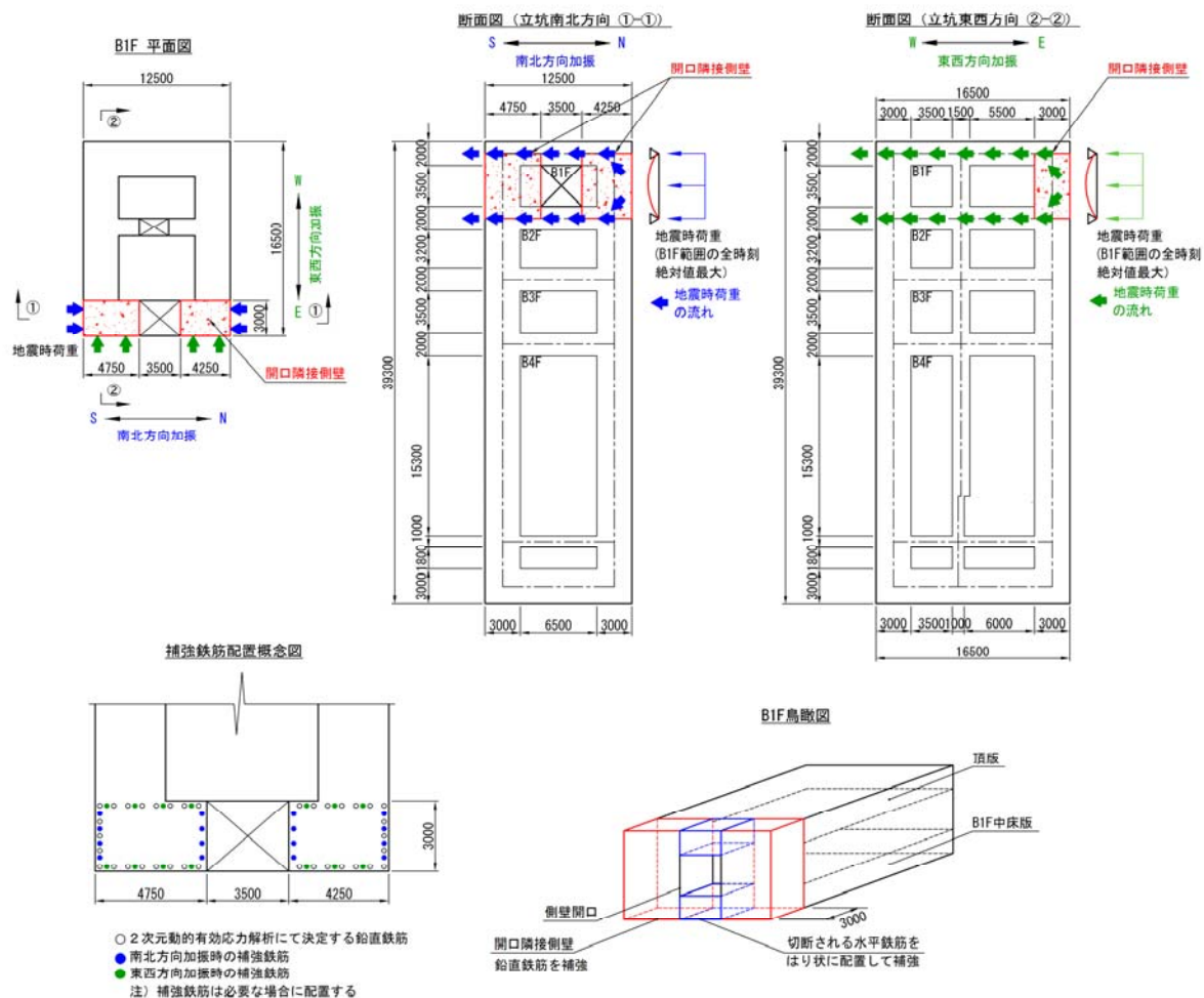
図 7-1 側壁開口部概念図
