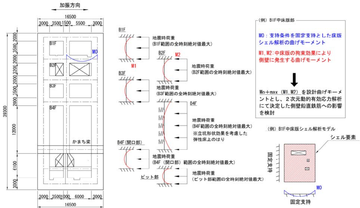
図 9-1 版部材から側壁に廻り込む曲げモーメント算定概念図
