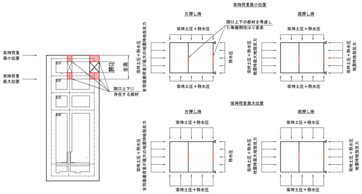
図 5-4 水平断面解析モデル概念図（開口部を含む構造部）
