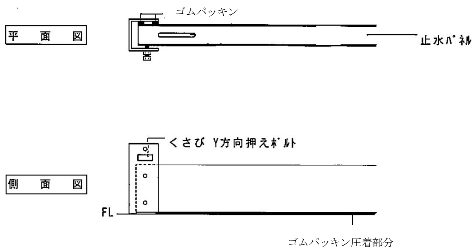
第4-5図 止水板の概要図
