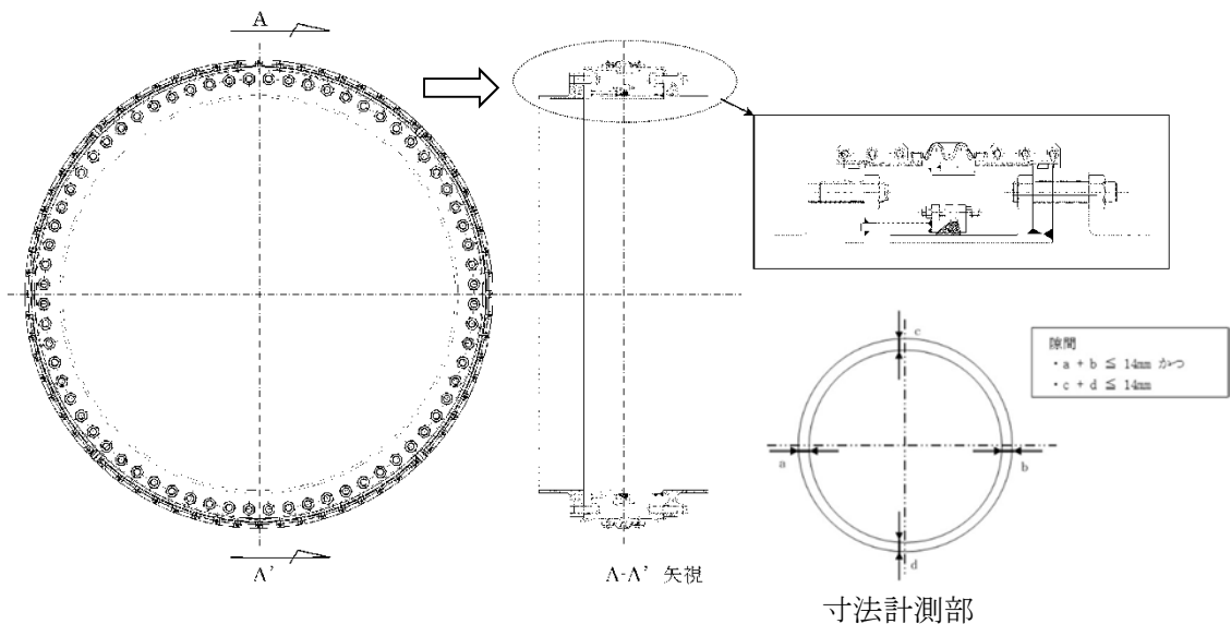
第4-15図 循環水管可撓継手設置時のすき間管理について
