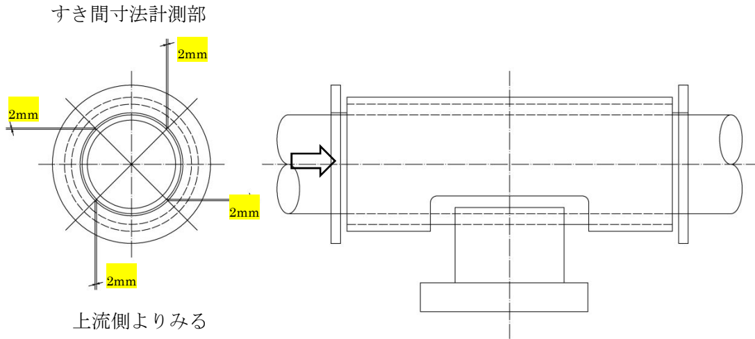
第4-16図 防護カバーと配管のすき間設定
