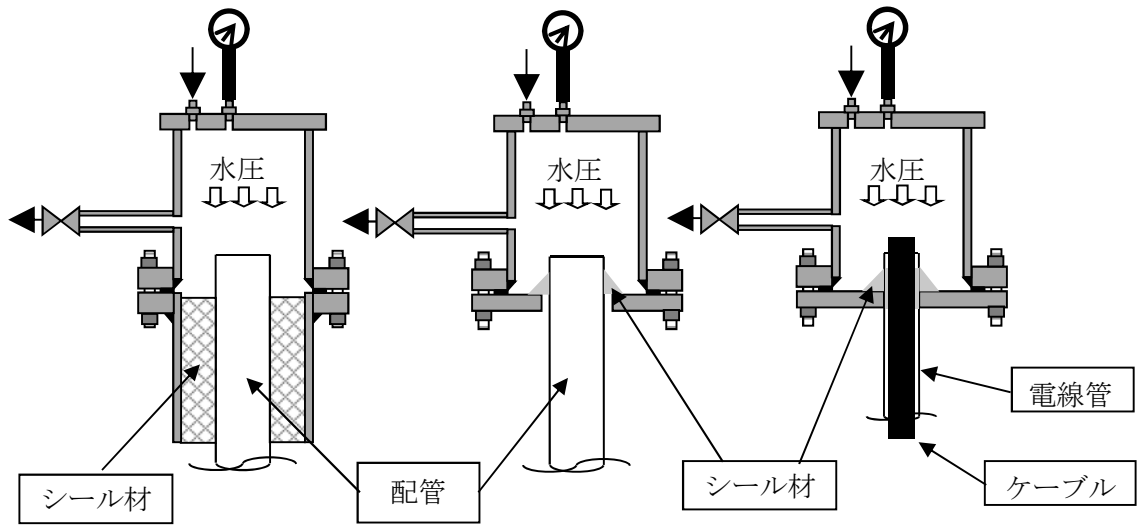
第4-10図 シール材の耐圧漏えい試験の概要
