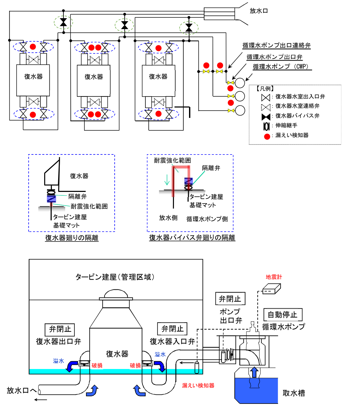
第4-13図 設備概要
