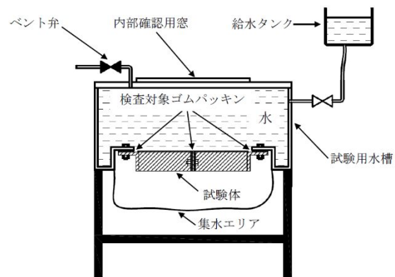
第4-7図 ゴムパッキンの漏えい試験の概要
