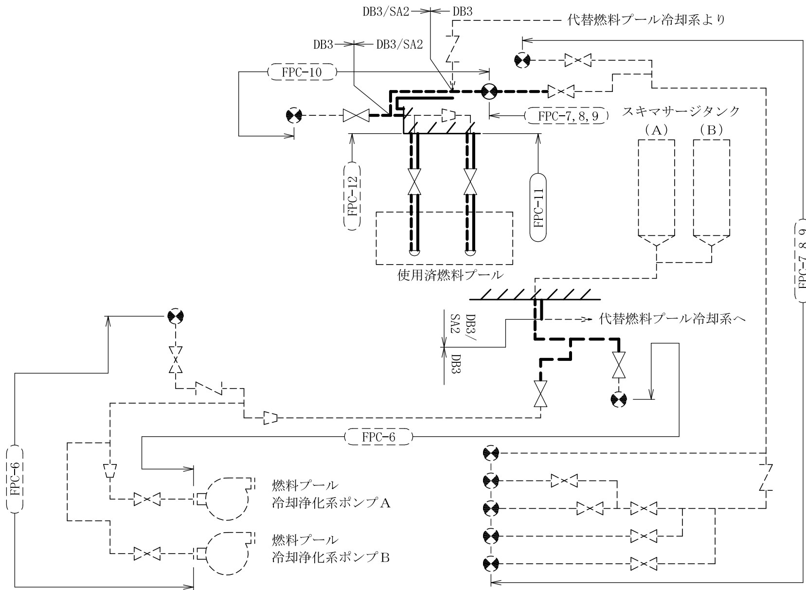
燃料プール冷却浄化系概略系統図
