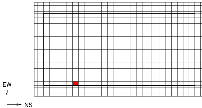
(b) NS 方向、部材厚 2.5m (要素番号 50308、ケース 108)
