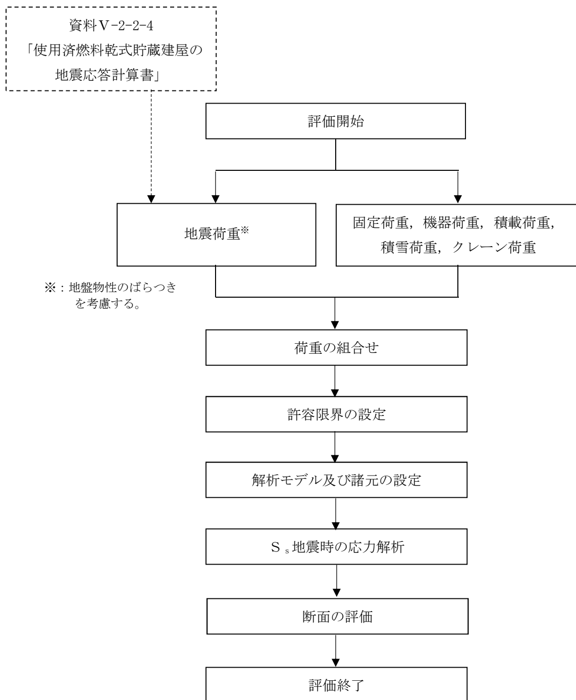
図 3-1 応力解析による評価フロー（基礎）
