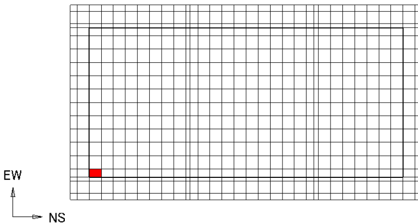
(d) EW 方向、部材厚 2.5m (要素番号 50303、ケース 104)
