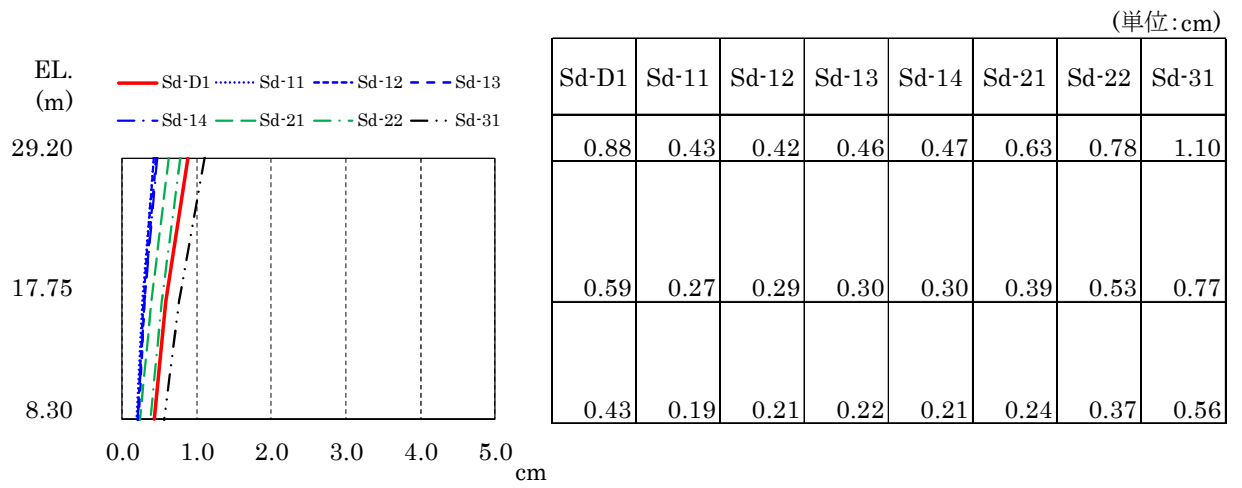
(a) 壁部
