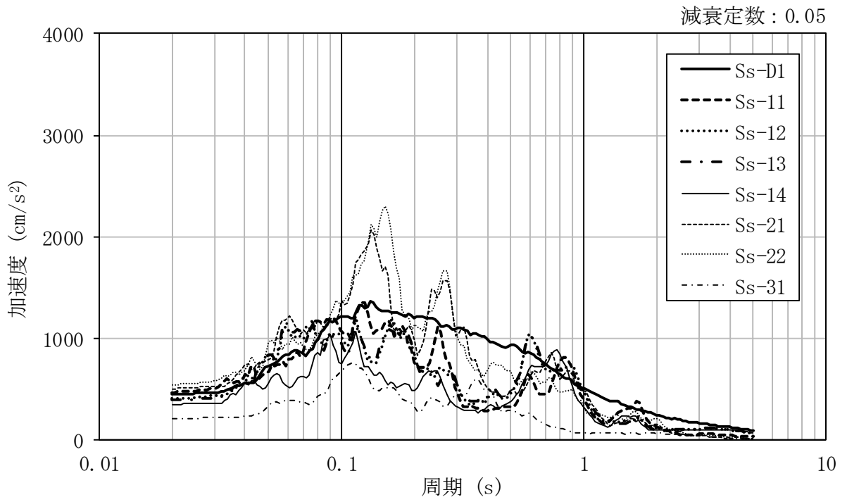
図 3-13 (1/2) 入力地震動の加速度応答スペクトル ( S_s , UD 方向, EL. 5.8 m)
