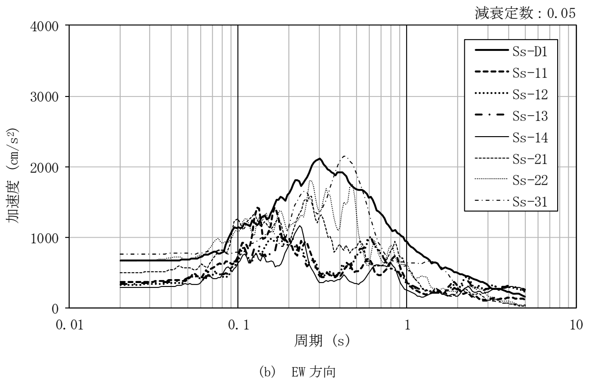
図 3-11 (1/2) 入力地震動の加速度応答スペクトル ( S_s , EL. 5.8 m)
