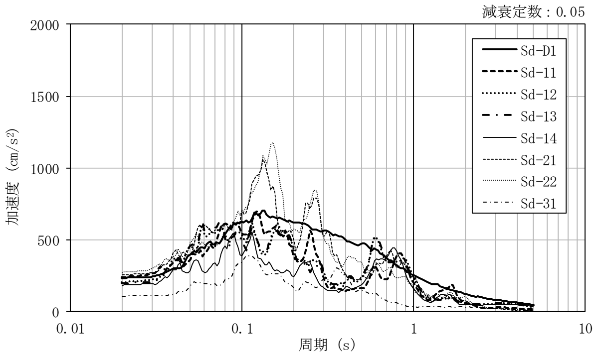
図 3-13 (2/2) 入力地震動の加速度応答スペクトル ( S_a , UD 方向, EL. 5.8 m)
