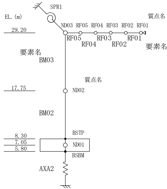
図 3-9 地震応答解析モデル (UD 方向)
