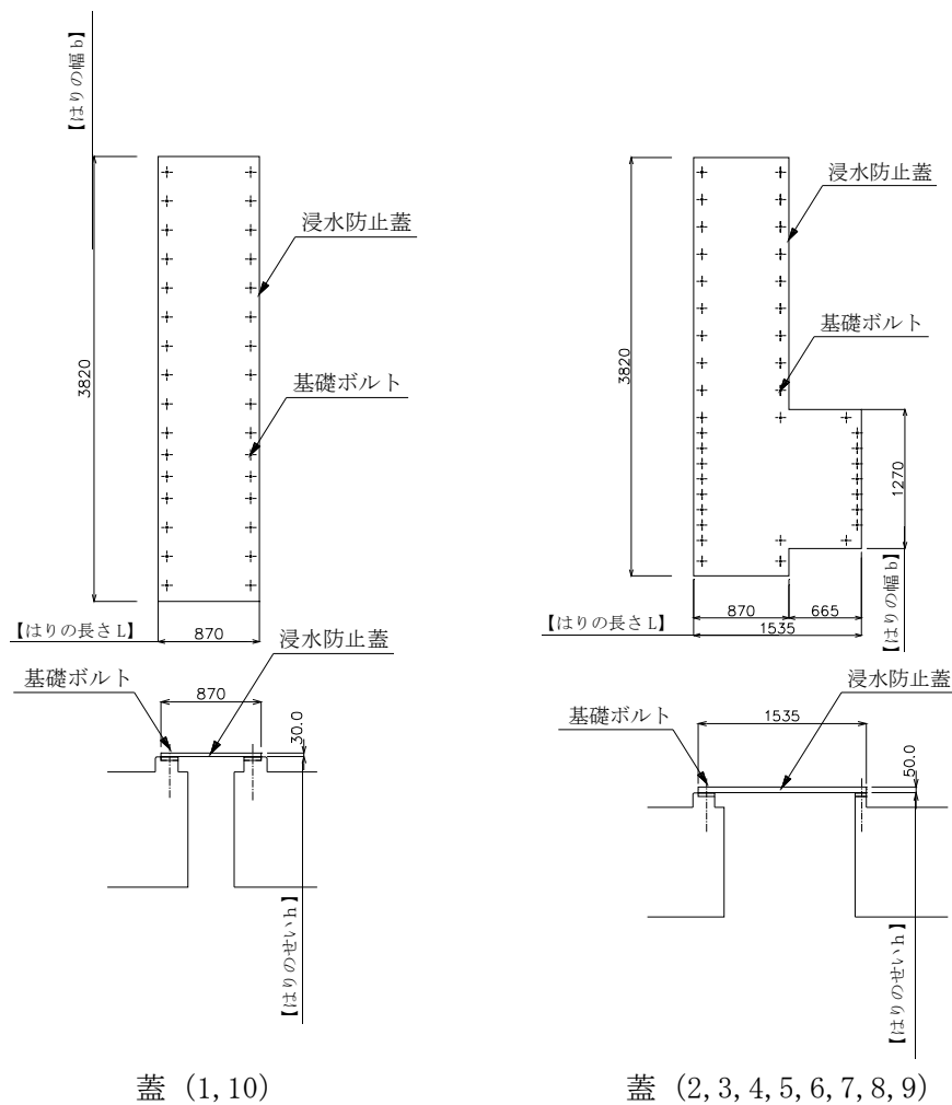
図 6.9.1-2 取水路点検用開口部浸水防止蓋の構造図
