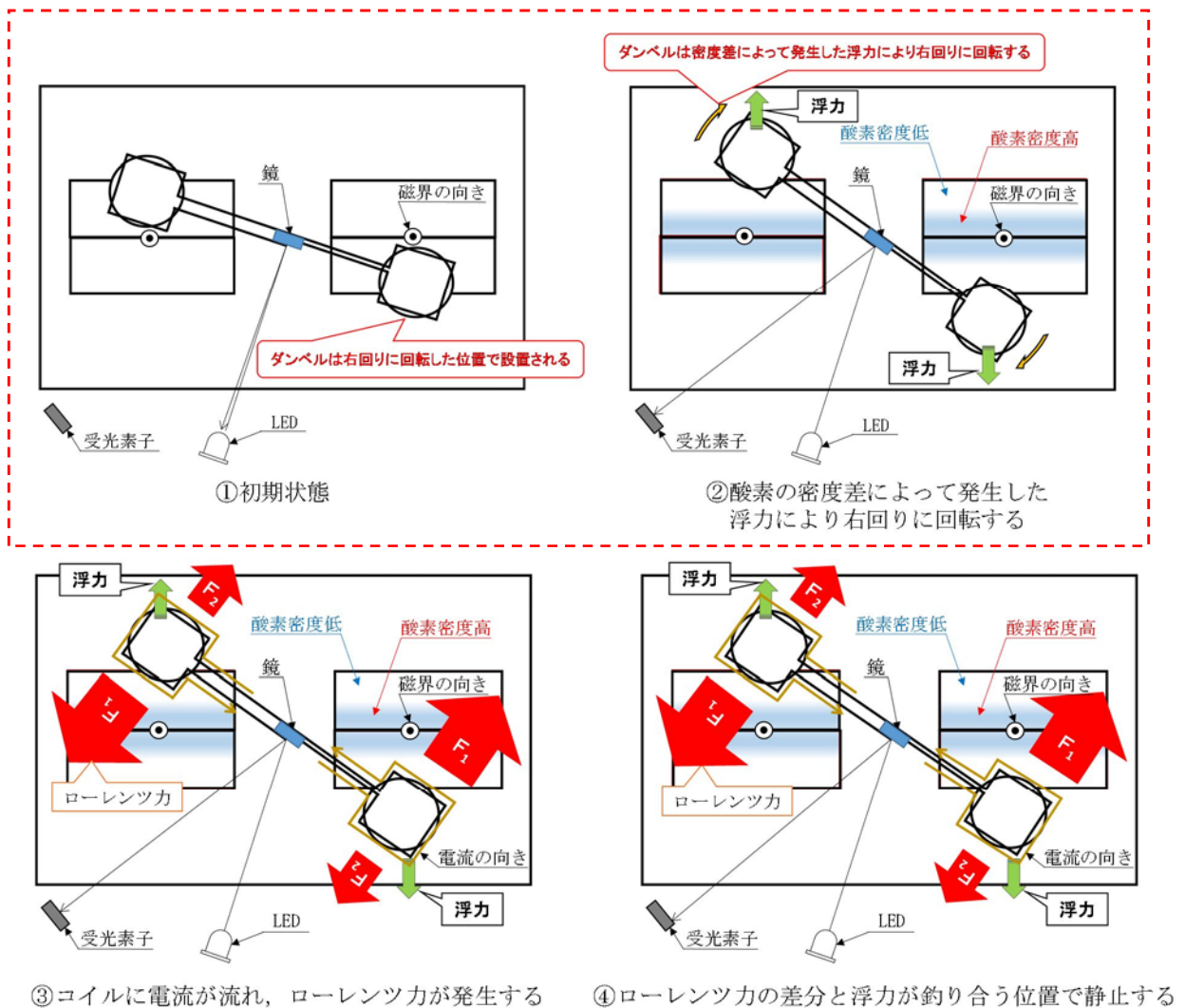
図 1-2-2-3 格納容器内酸素濃度（SA）の動作原理イメージ
