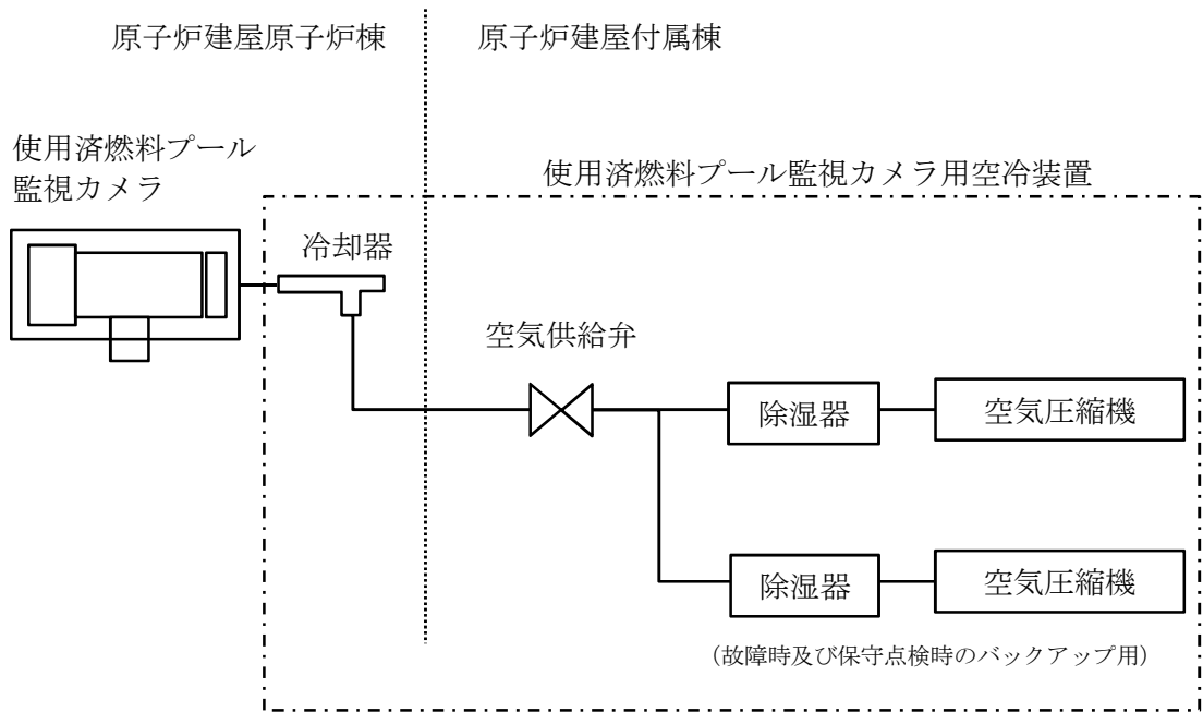
図2 使用済燃料プール監視カメラ用空冷装置の空気供給概略図
