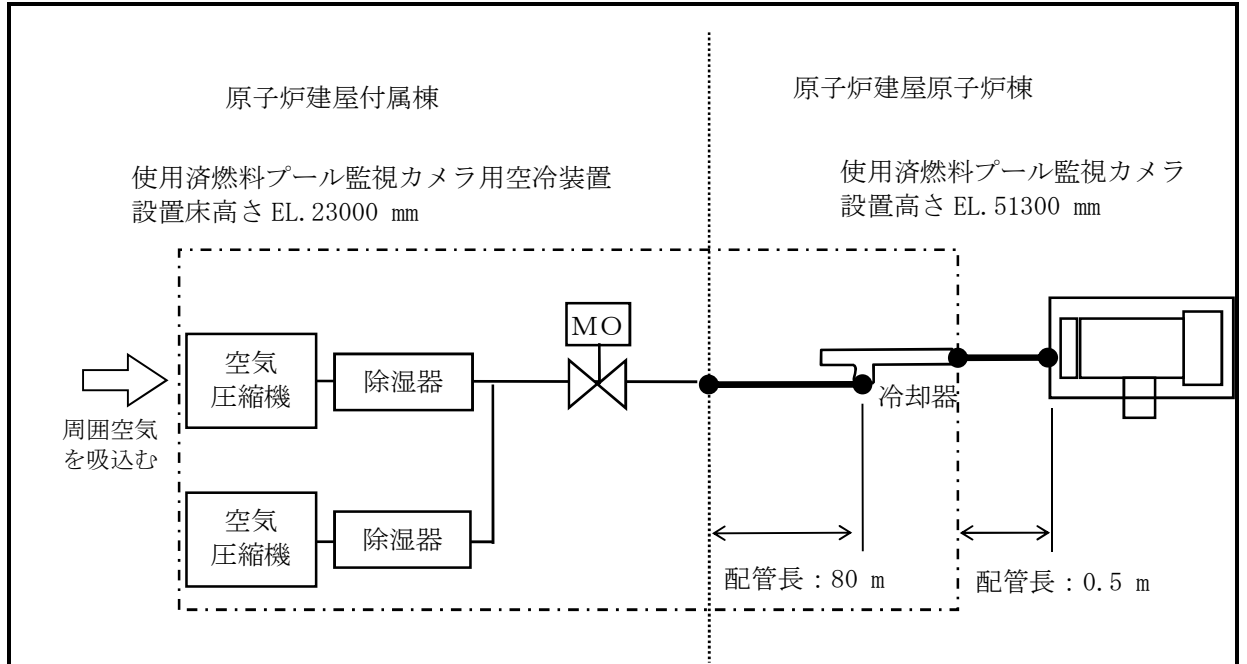
図1 使用済燃料プール監視カメラ用空冷装置の空気供給概略図
