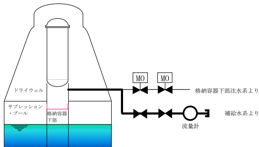
第7-2図 格納容器床ドレンサンプ水張系統概略図
