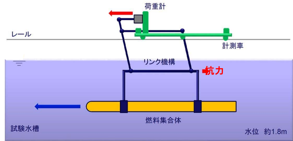
図2 試験体系
