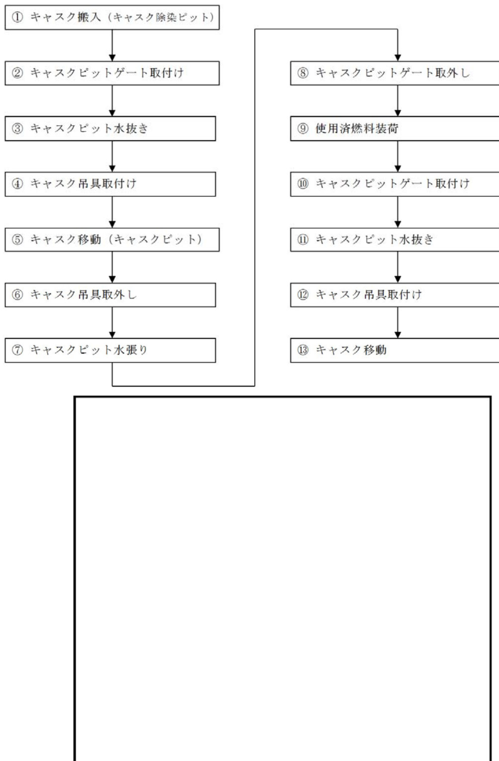
第5-1図 キャスク取扱い作業フロー（例）
