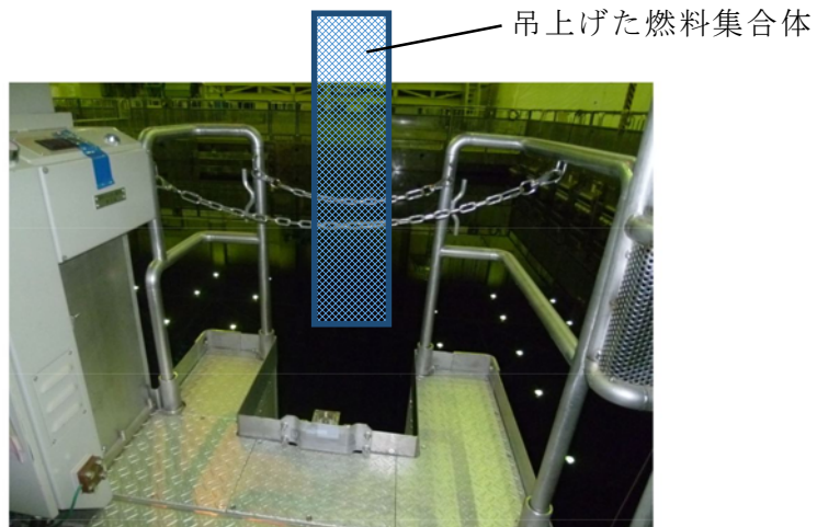
図 1 0 チャンネル着脱機のカートへ吊下ろす直前の状況（イメージ）
