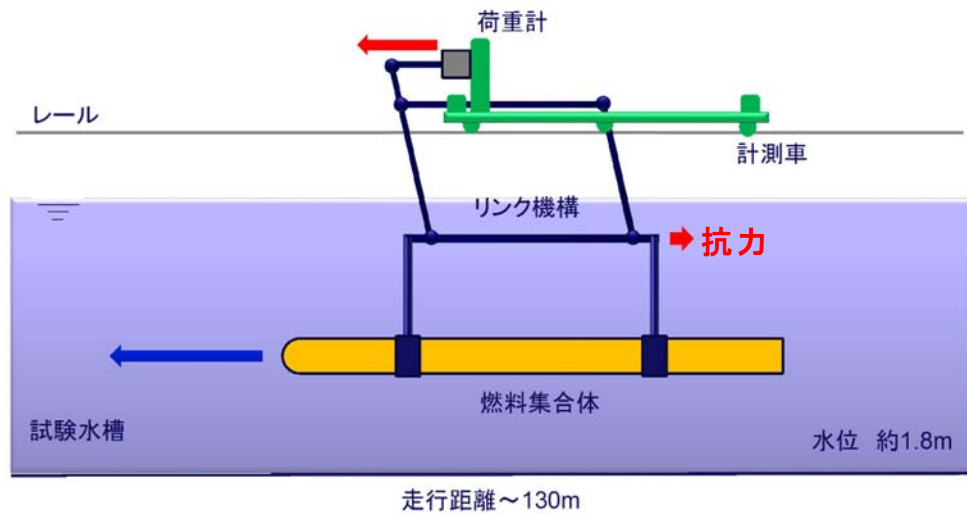
図8 抗力係数測定試験イメージ
