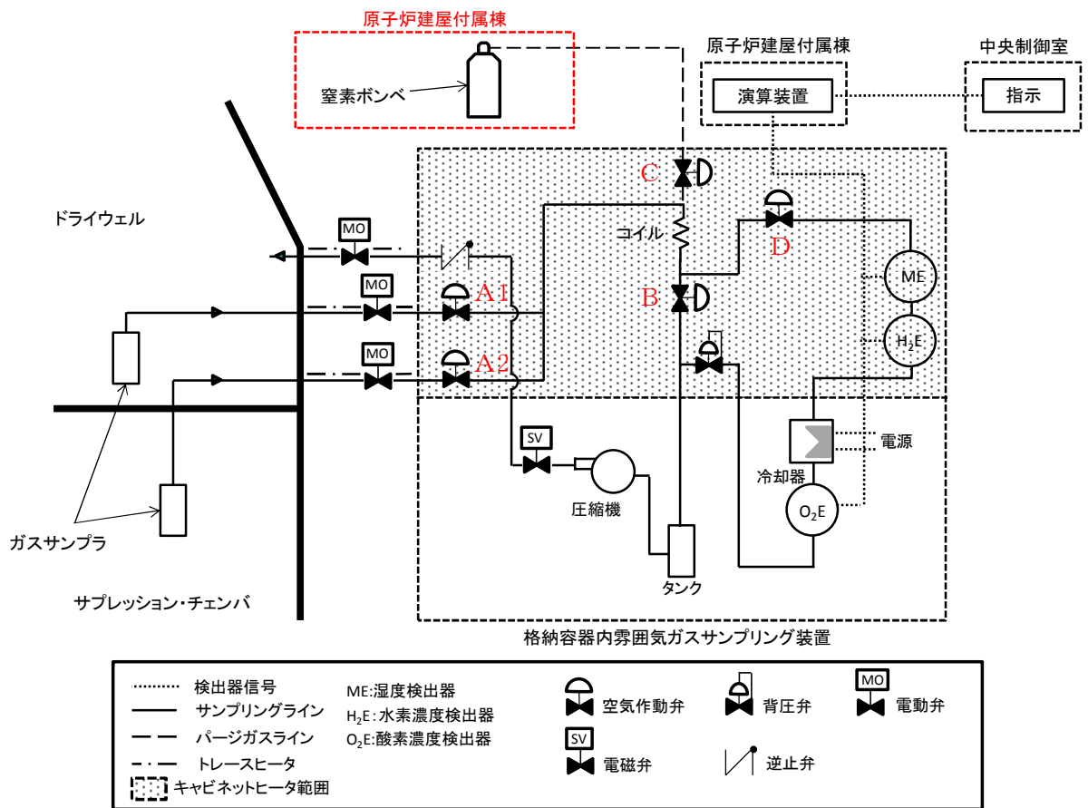
図 1-3-1 格納容器内雰囲気ガスサンプリング装置の構成
