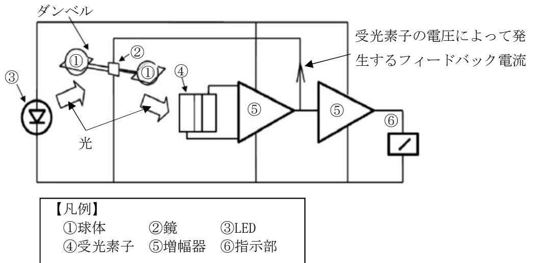
図 1-2-2-2 格納容器内酸素濃度 (S A) 検出回路図
