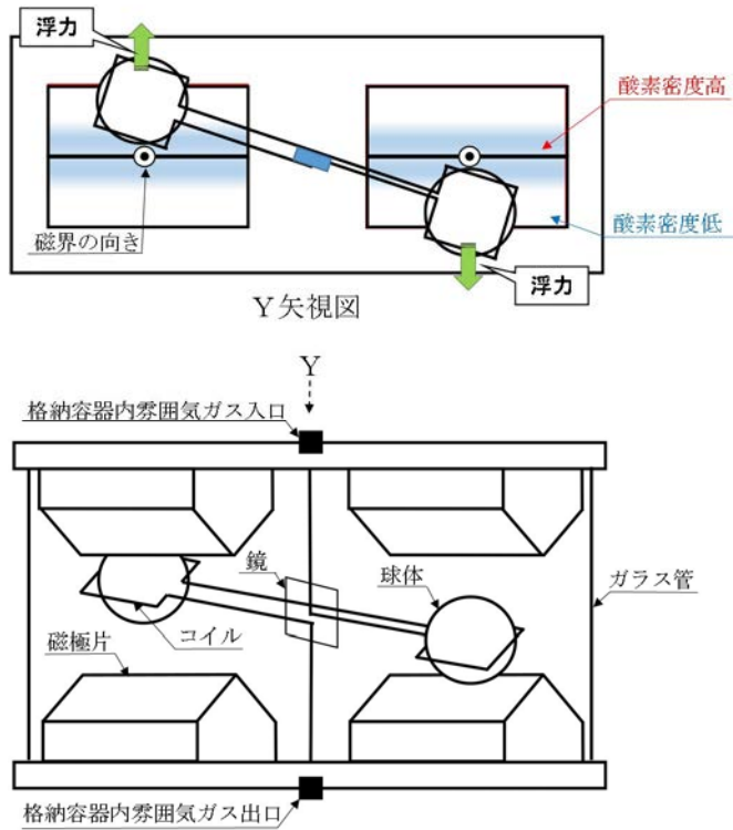
図 1-2-2-1 格納容器内酸素濃度 (S A) の概要図
