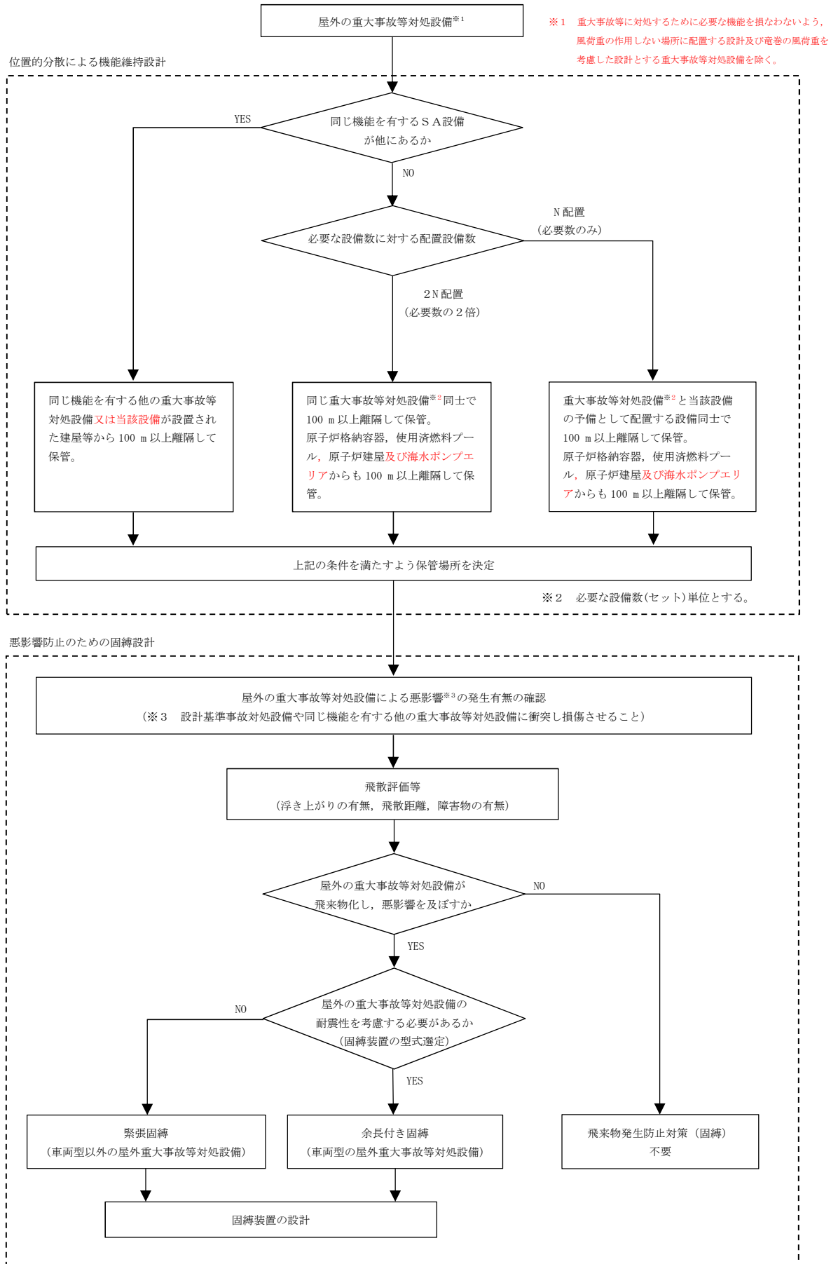
図 2-1 屋外重大事故等対処設備の竜巻防護に関する設計方針のフロー
