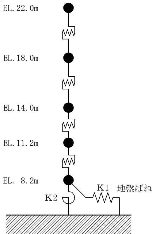
図 3-3 地震応答解析モデル
