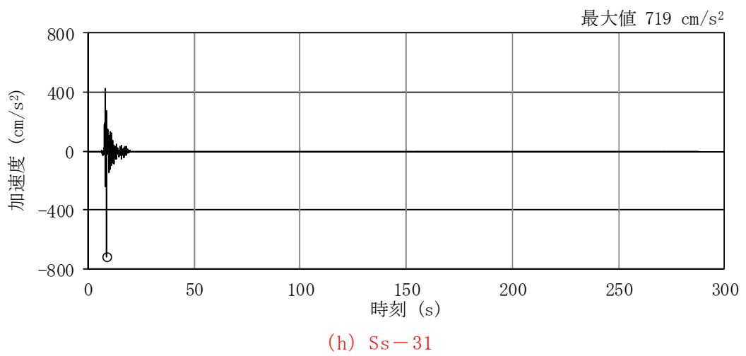
図 3-1 (3/3) 加速度時刻歴波形 (Ss)
