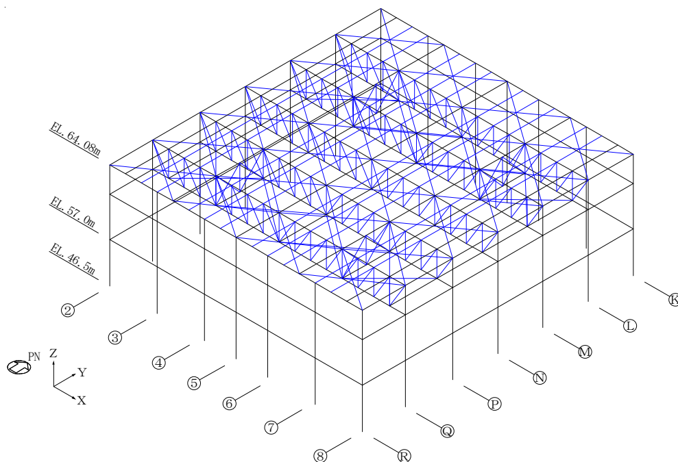
図4-67 解析モデル（屋根トラス）
