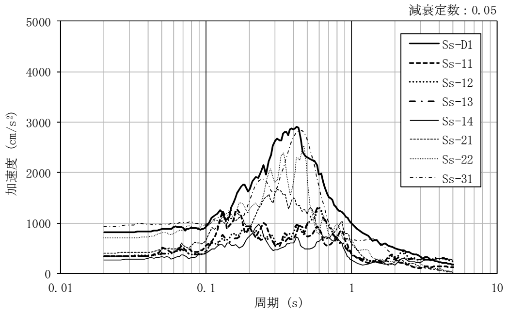
図 4-39 加速度応答スペクトル (基準地震動 S_s , EW 方向並進成分, 基本ケース)
