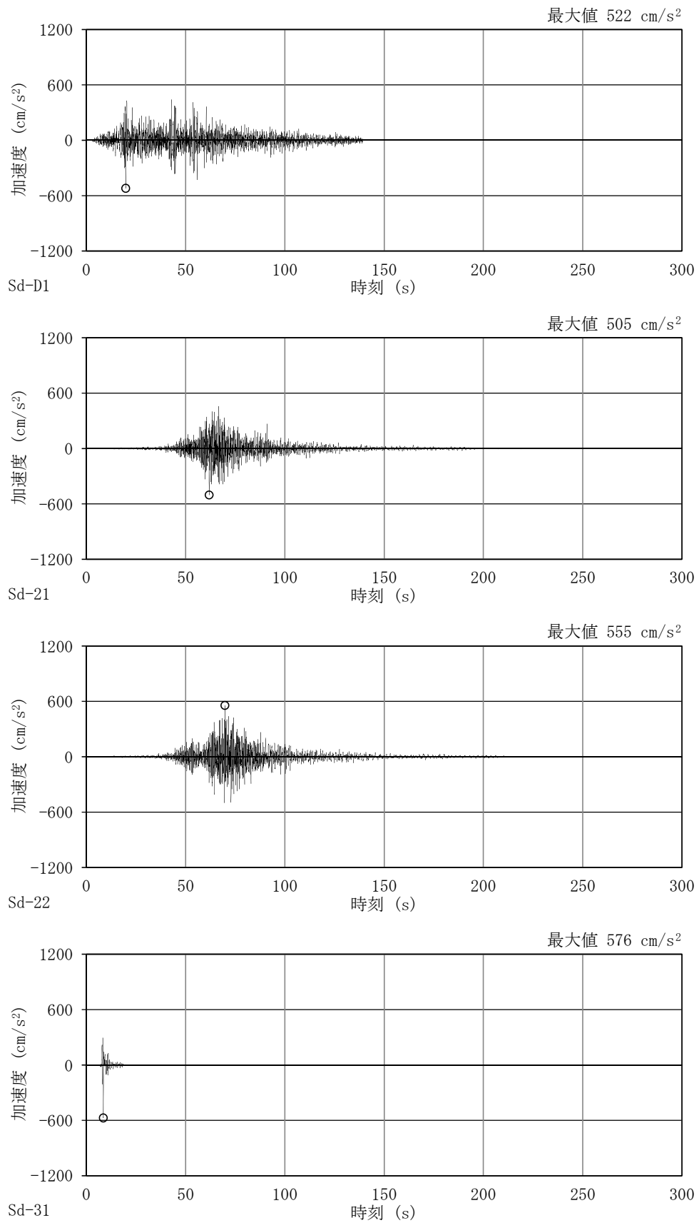
図 4-16 加速度時刻歴波形
