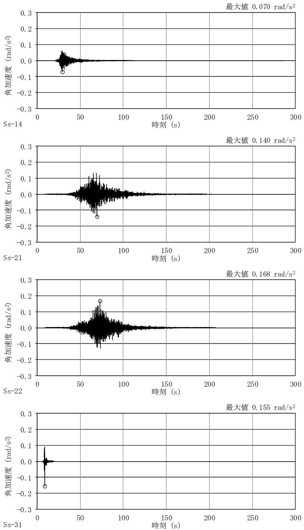
図 4-42 (2/2) 加速度時刻歴波形 (基準地震動 S_s , EW 方向回転成分, 基本ケース)
