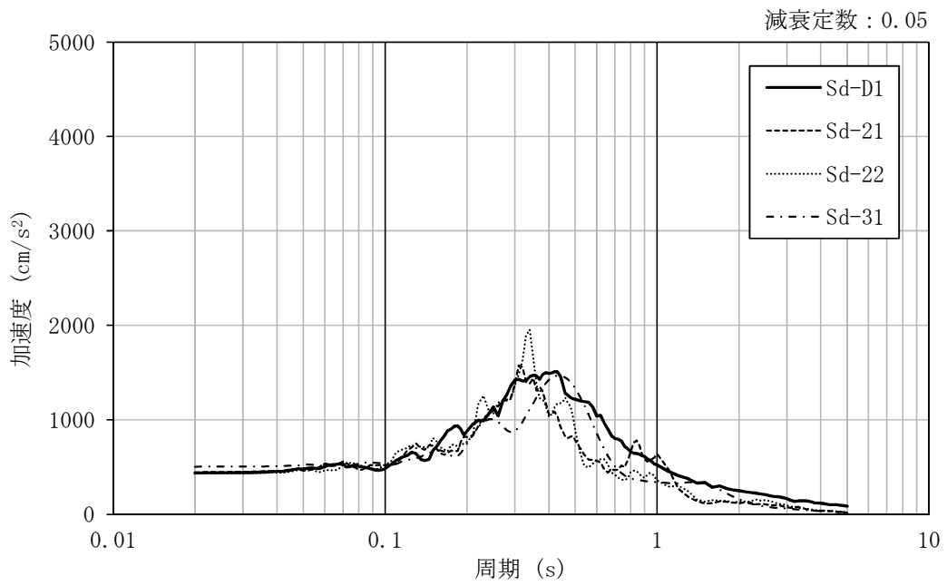
図 4-25 加速度応答スペクトル (弾性設計用地震動 S_a , NS 方向並進成分, 地盤物性のばらつきを考慮 ( -\sigma ))
