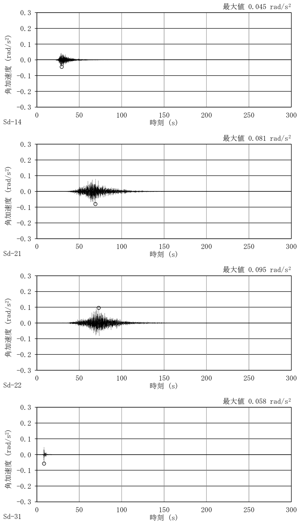
図 4-12 (2/2) 加速度時刻歴波形 (弾性設計用地震動 S_d , EW 方向回転成分, 基本ケース)
