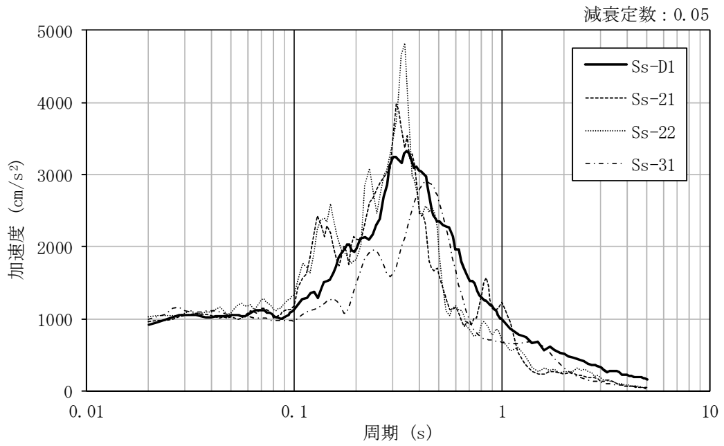
図 4-45 加速度応答スペクトル (基準地震動 S_s , NS 方向並進成分, 地盤物性のばらつきを考慮 (+ \sigma ))
