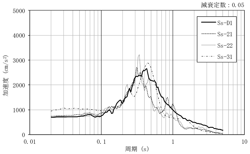
図 4-55 加速度応答スペクトル (基準地震動 S_s , NS 方向並進成分, 地盤物性のばらつきを考慮 ( -\sigma ))
