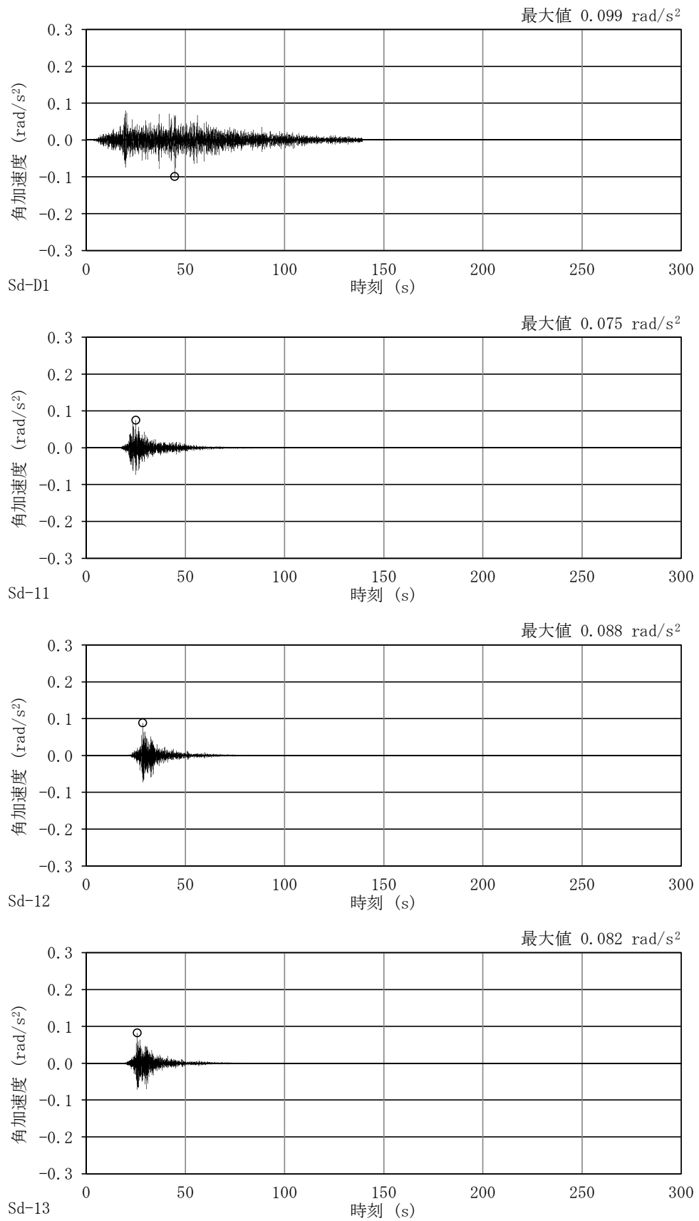
図 4-8 (1/2) 加速度時刻歴波形 (弾性設計用地震動 S_a , NS 方向回転成分, 基本ケース)
