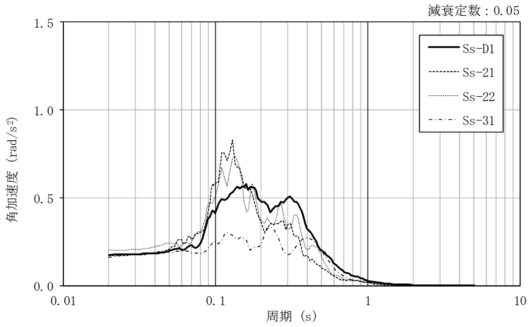
図 4-51 加速度応答スペクトル (基準地震動 S_s , EW 方向回転成分, 地盤物性のばらつきを考慮 (+ \sigma ))
