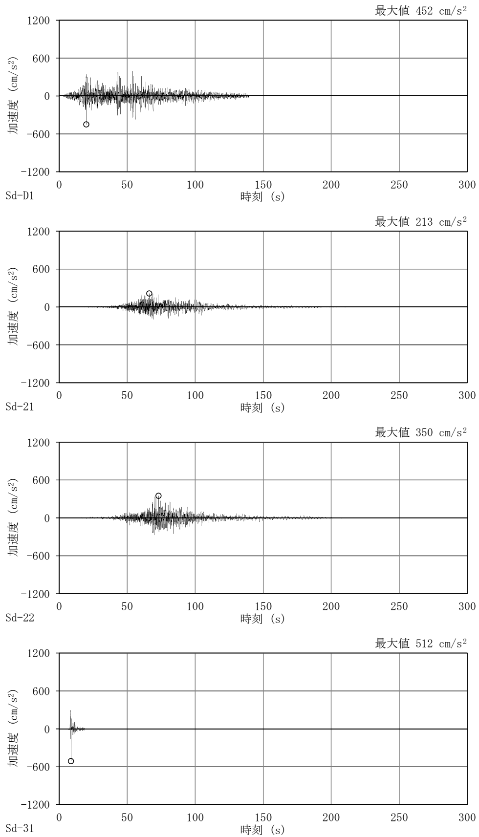
図 4-30 加速度時刻歴波形
