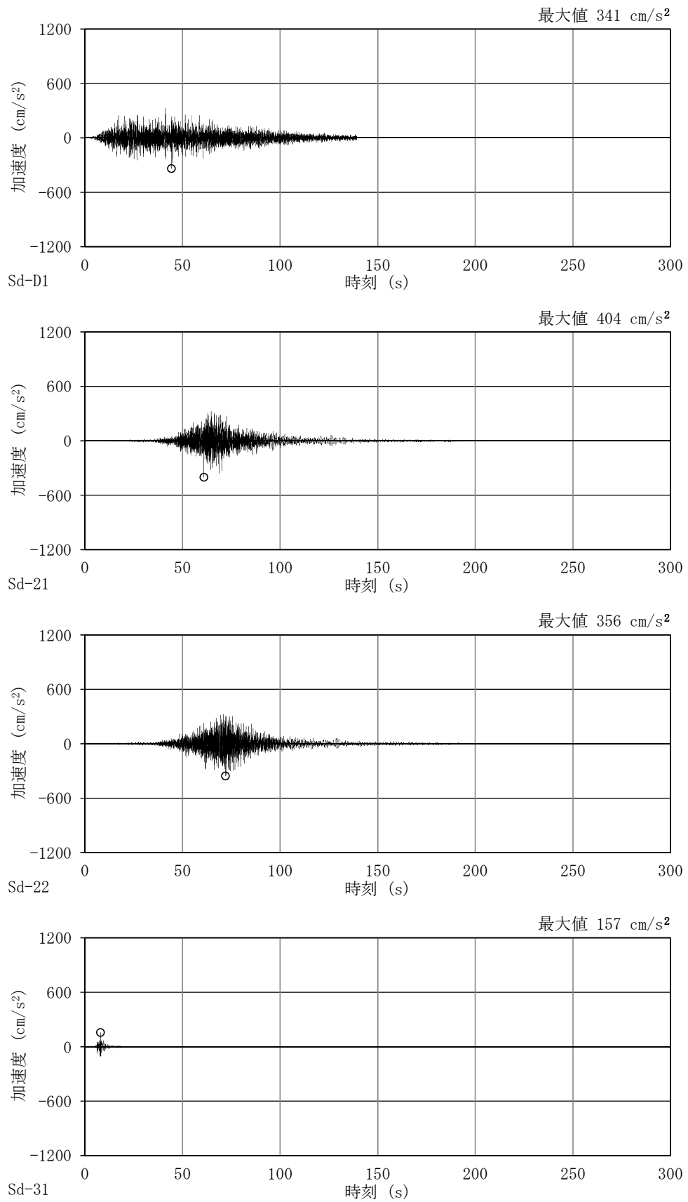
図 4-34 加速度時刻歴波形 (弾性設計用地震動 S_d , UD 方向, 地盤物性のばらつきを考慮 ( -\sigma ))
