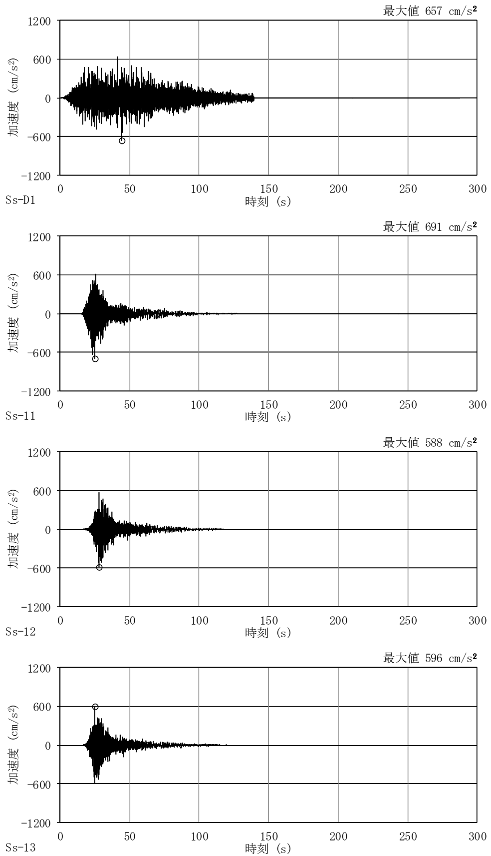
図 4-44 (1/2) 加速度時刻歴波形 (基準地震動 S s , UD 方向, 基本ケース)
