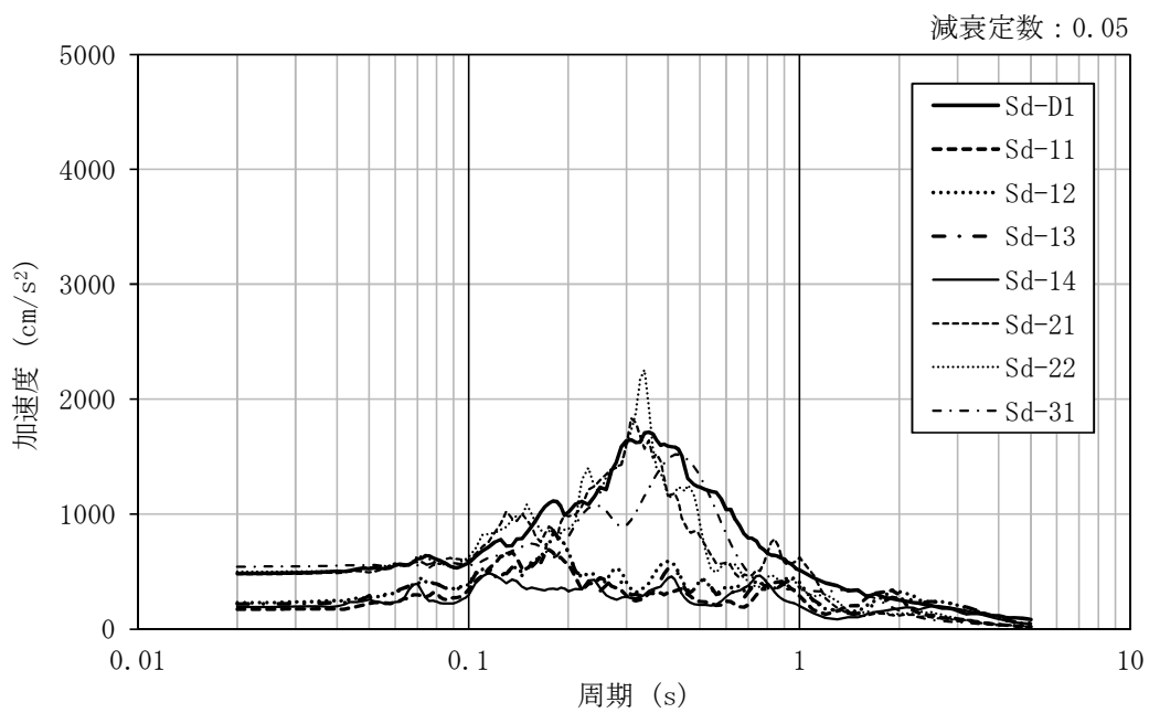
図 4-5 加速度応答スペクトル (弾性設計用地震動 S_d , NS 方向並進成分, 基本ケース)
