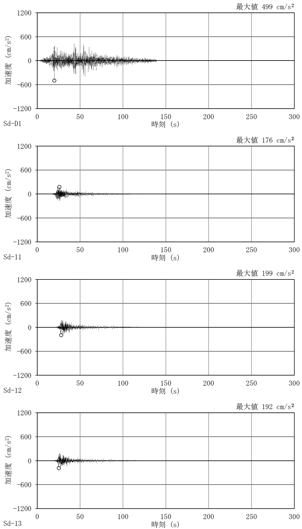
図 4-10 (1/2) 加速度時刻歴波形 (弾性設計用地震動 S_d , EW 方向並進成分, 基本ケース)
