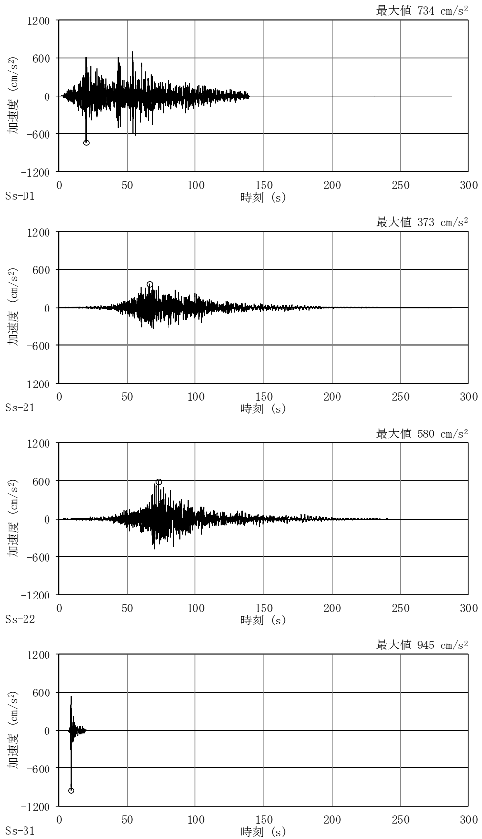
図 4-60 加速度時刻歴波形
