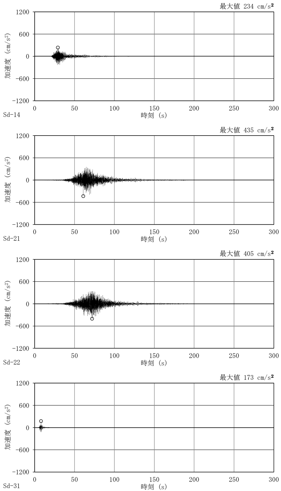
図 4-14 (2/2) 加速度時刻歴波形 (弾性設計用地震動 S a , UD 方向, 基本ケース)
