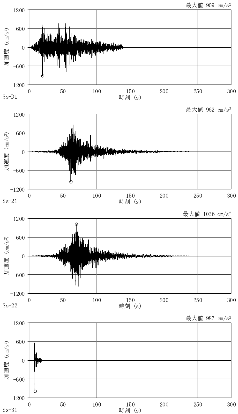
図 4-46 加速度時刻歴波形
