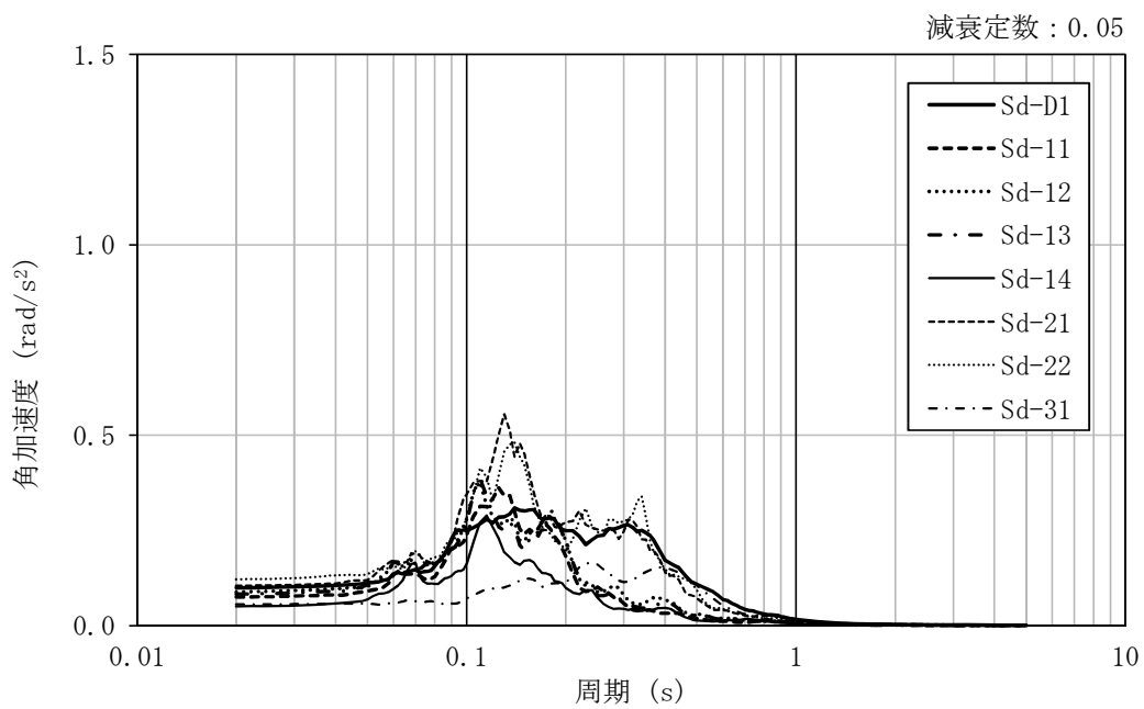
図 4-7 加速度応答スペクトル (弾性設計用地震動 S_d , NS 方向回転成分, 基本ケース)
