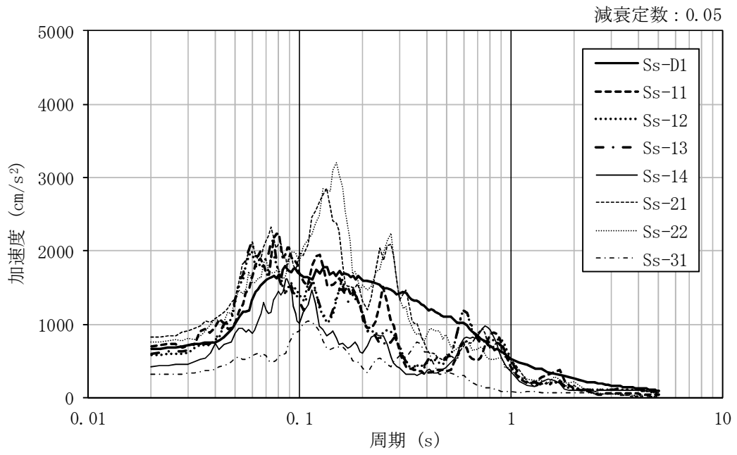
図 4-43 加速度応答スペクトル (基準地震動 S s , UD 方向, 基本ケース)
