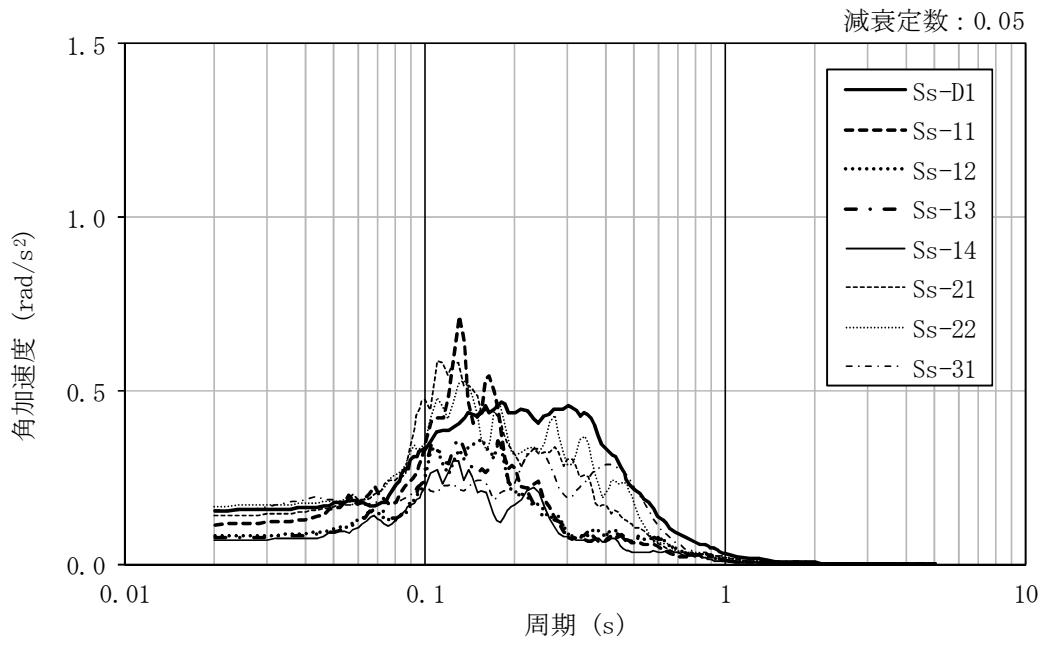
図 4-41 加速度応答スペクトル (基準地震動 S_s , EW 方向回転成分, 基本ケース)
