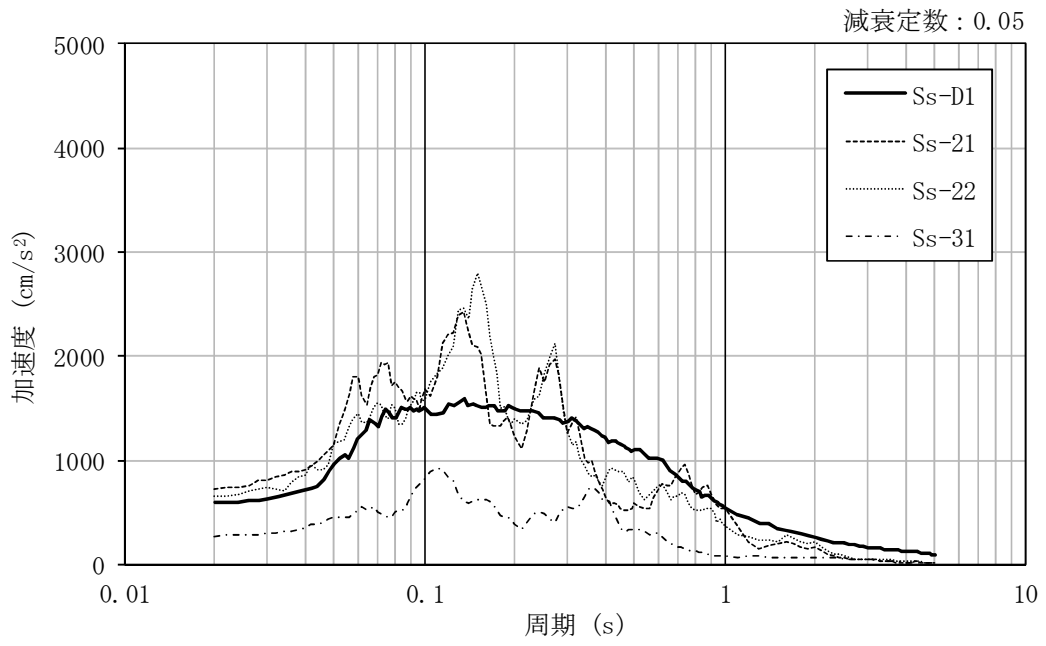
図 4-63 加速度応答スペクトル (基準地震動 S_s , UD 方向, 地盤物性のばらつきを考慮 ( -\sigma ))
