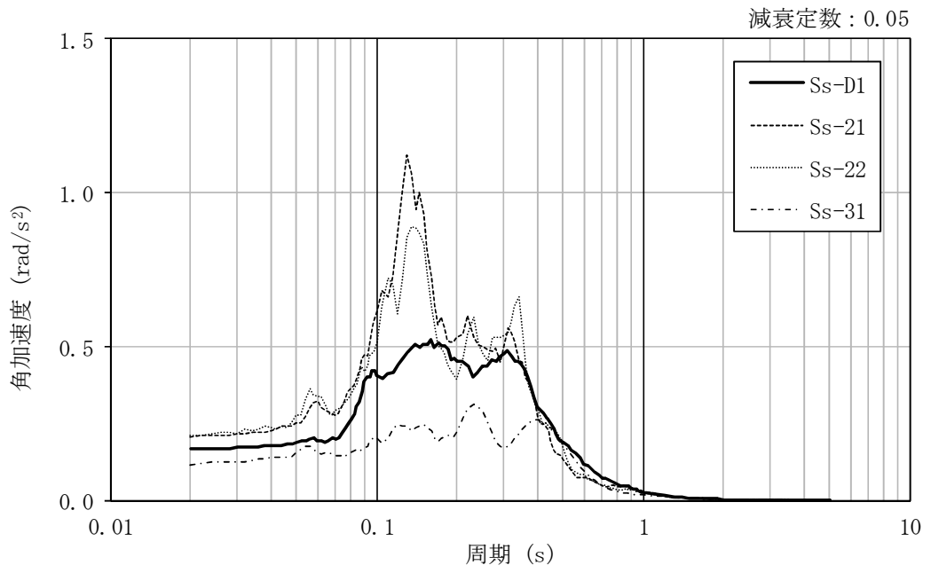
図 4-47 加速度応答スペクトル (基準地震動 S_s , NS 方向回転成分, 地盤物性のばらつきを考慮 (+ \sigma ))
