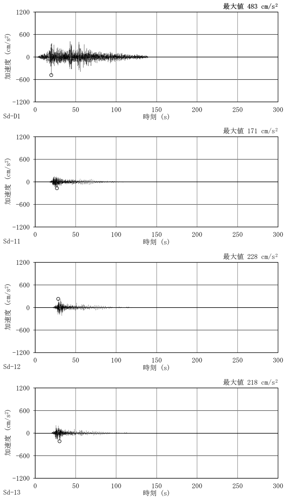
図 4-6 (1/2) 加速度時刻歴波形 (弾性設計用地震動 S_a , NS 方向並進成分, 基本ケース)
