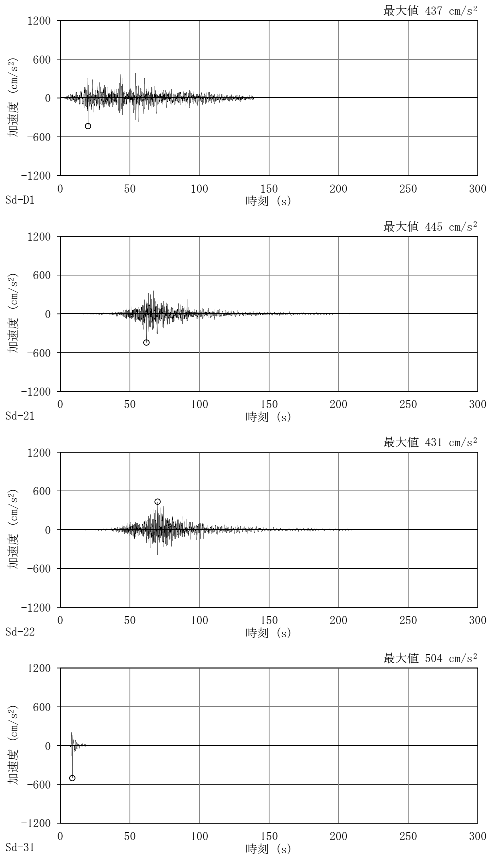
図 4-26 加速度時刻歴波形
