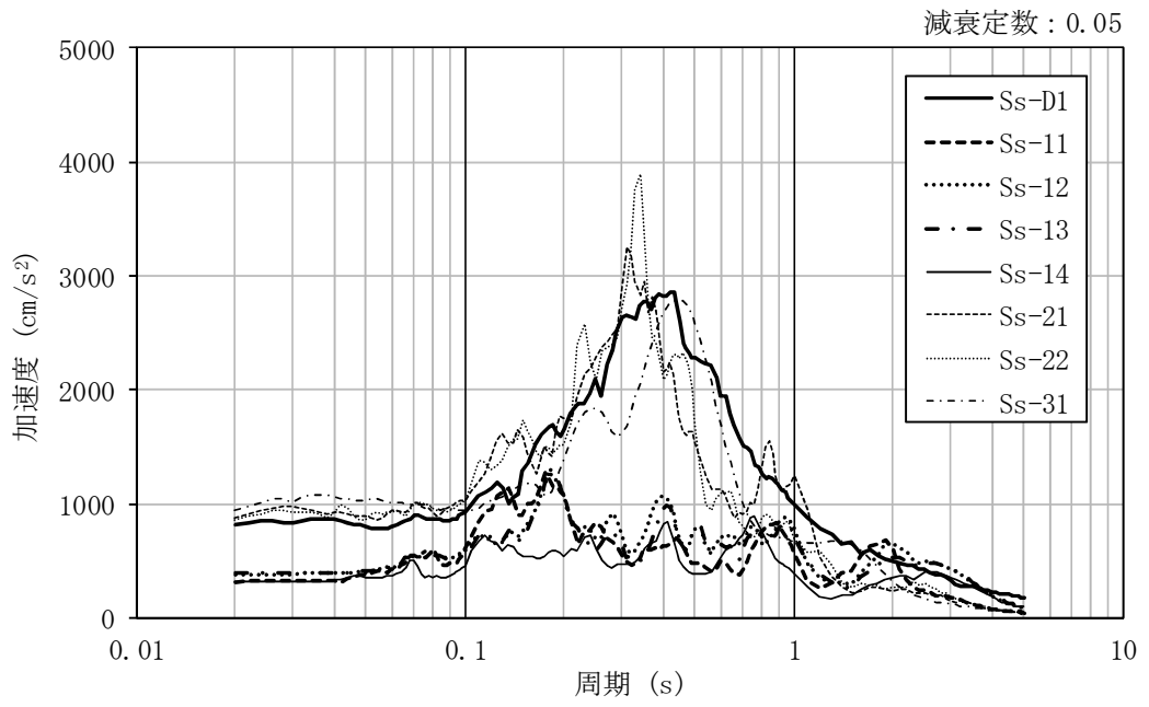
図 4-35 加速度応答スペクトル (基準地震動 S_s , NS 方向並進成分, 基本ケース)
