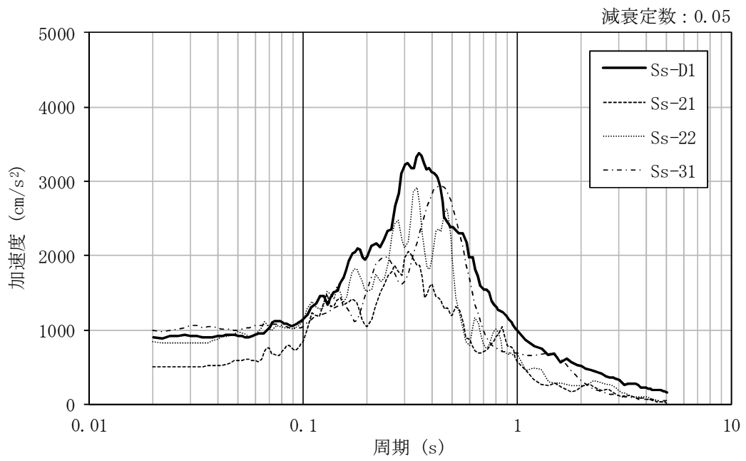
図 4-49 加速度応答スペクトル (基準地震動 S_s , EW 方向並進成分, 地盤物性のばらつきを考慮 (+ \sigma ))
