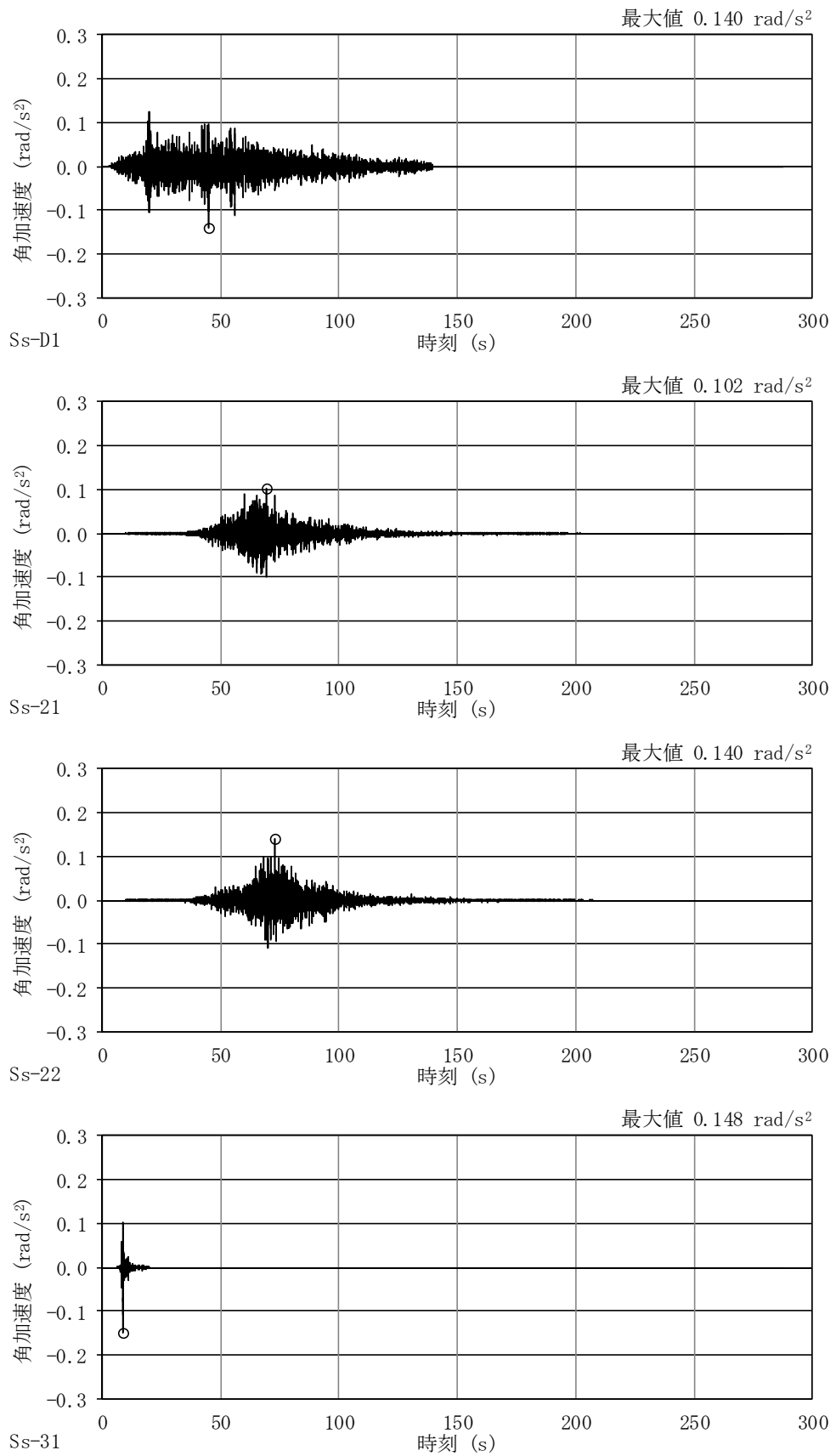
図 4-62 加速度時刻歴波形
