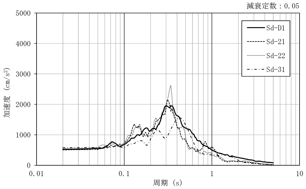
図 4-15 加速度応答スペクトル (弾性設計用地震動 S_a , NS 方向並進成分, 地盤物性のばらつきを考慮 (+ \sigma ))
