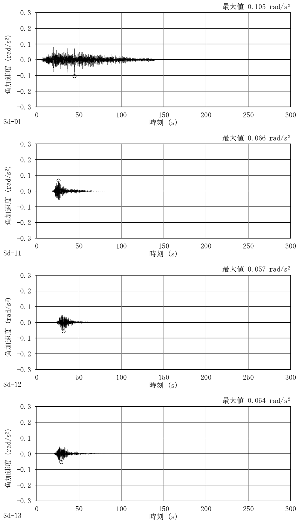
図 4-12 (1/2) 加速度時刻歴波形 (弾性設計用地震動 S_d , EW 方向回転成分, 基本ケース)
