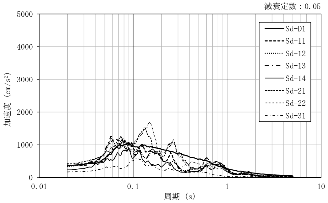
図 4-13 加速度応答スペクトル (弾性設計用地震動 S_d , UD 方向, 基本ケース)
