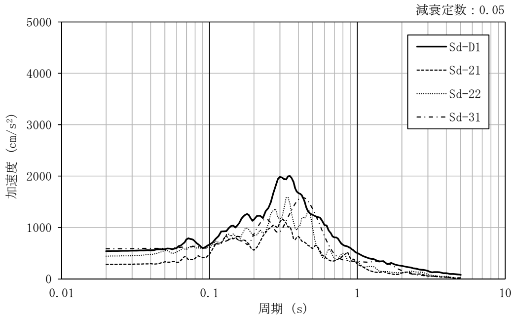
図 4-19 加速度応答スペクトル (弾性設計用地震動 S_a , EW 方向並進成分, 地盤物性のばらつきを考慮 (+ \sigma ))
