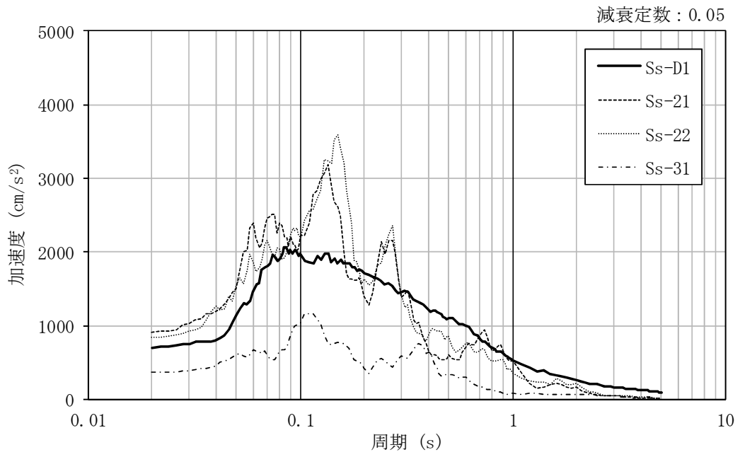
図 4-53 加速度応答スペクトル (基準地震動 S_s , UD 方向, 地盤物性のばらつきを考慮 (+ \sigma ))
