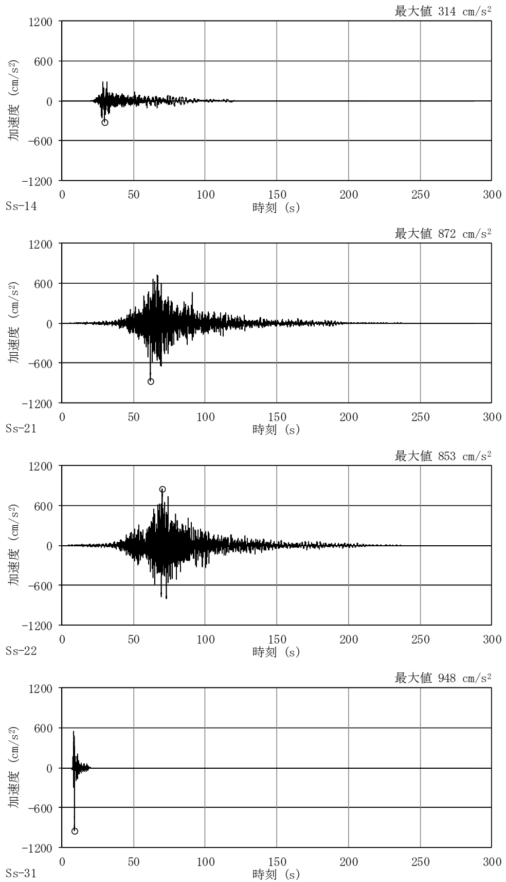
図 4-36 (2/2) 加速度時刻歴波形 (基準地震動 S_s , NS 方向並進成分, 基本ケース)
