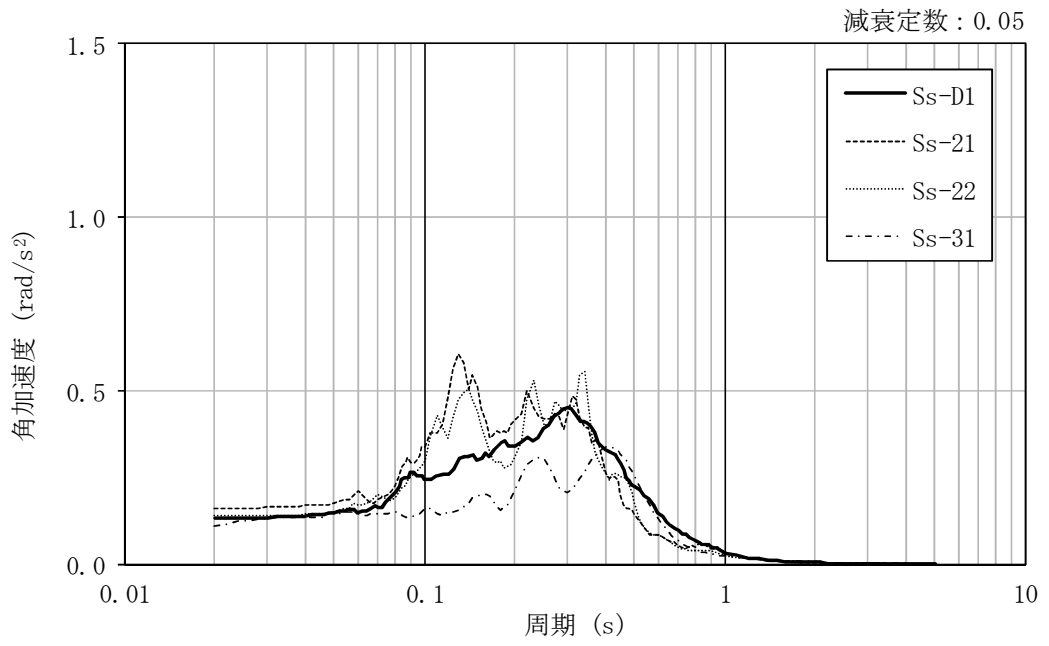
図 4-57 加速度応答スペクトル (基準地震動 S_s , NS 方向回転成分, 地盤物性のばらつきを考慮 ( -\sigma ))
