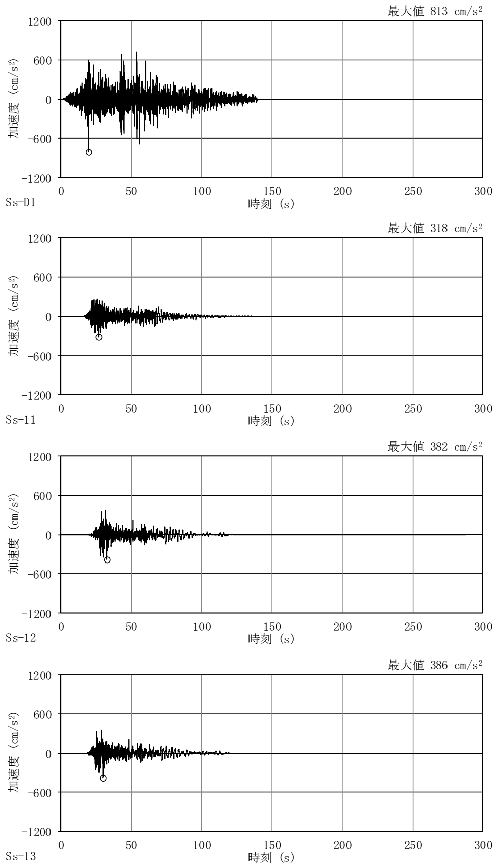
図 4-36 (1/2) 加速度時刻歴波形 (基準地震動 S_s , NS 方向並進成分, 基本ケース)
