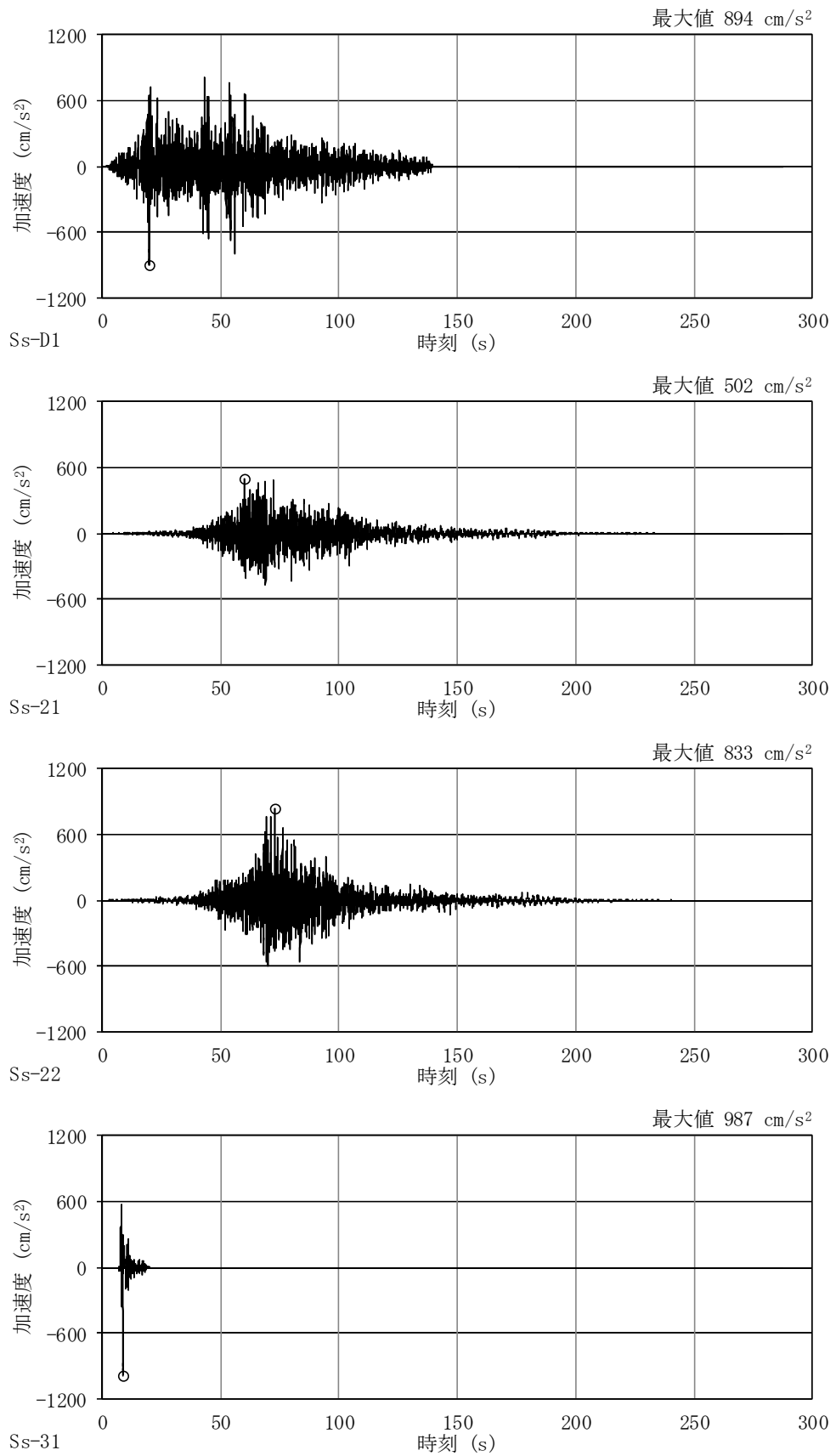
図 4-50 加速度時刻歴波形
