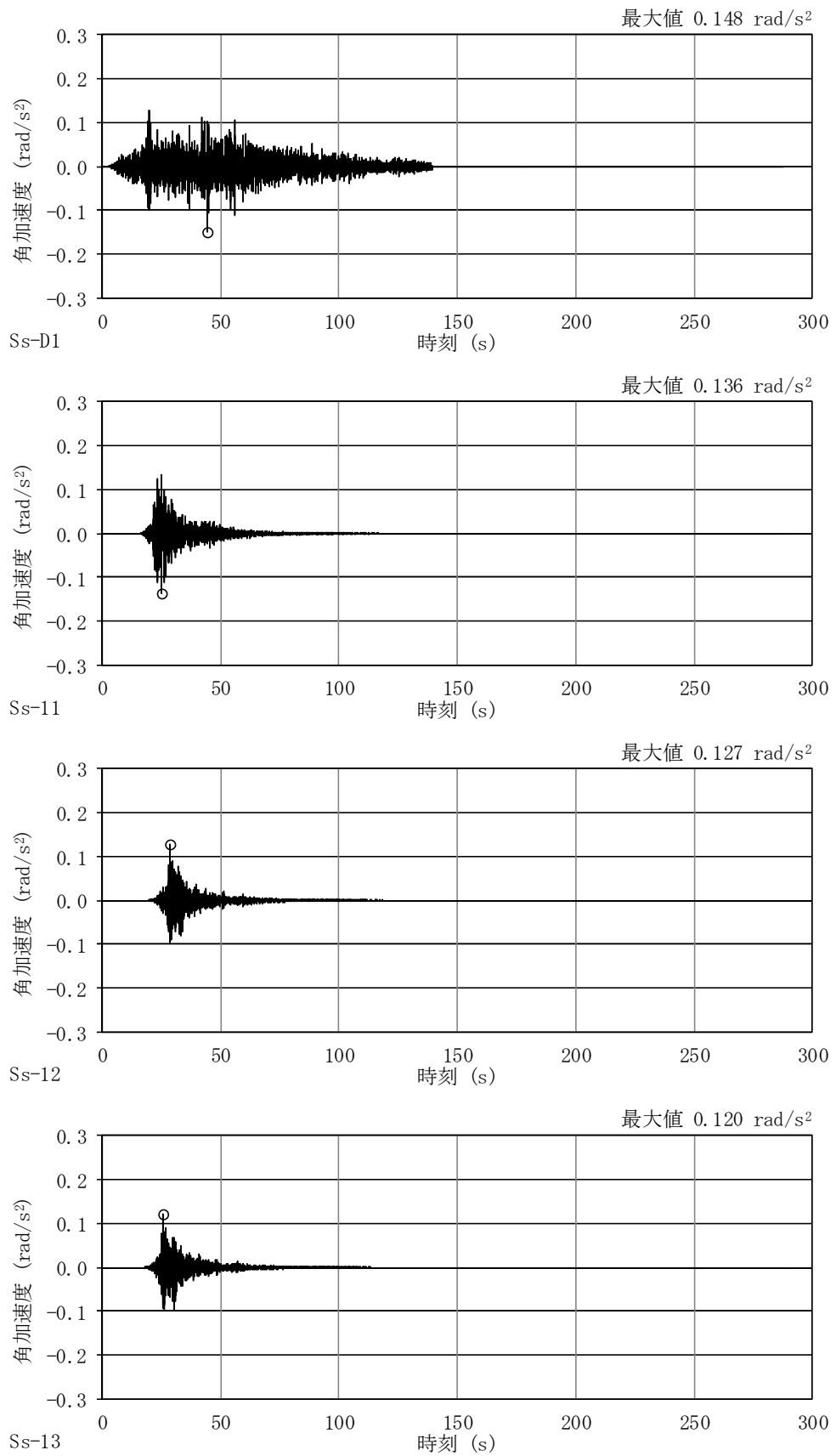
図 4-38 (1/2) 加速度時刻歴波形 (基準地震動 S_s , NS 方向回転成分, 基本ケース)
