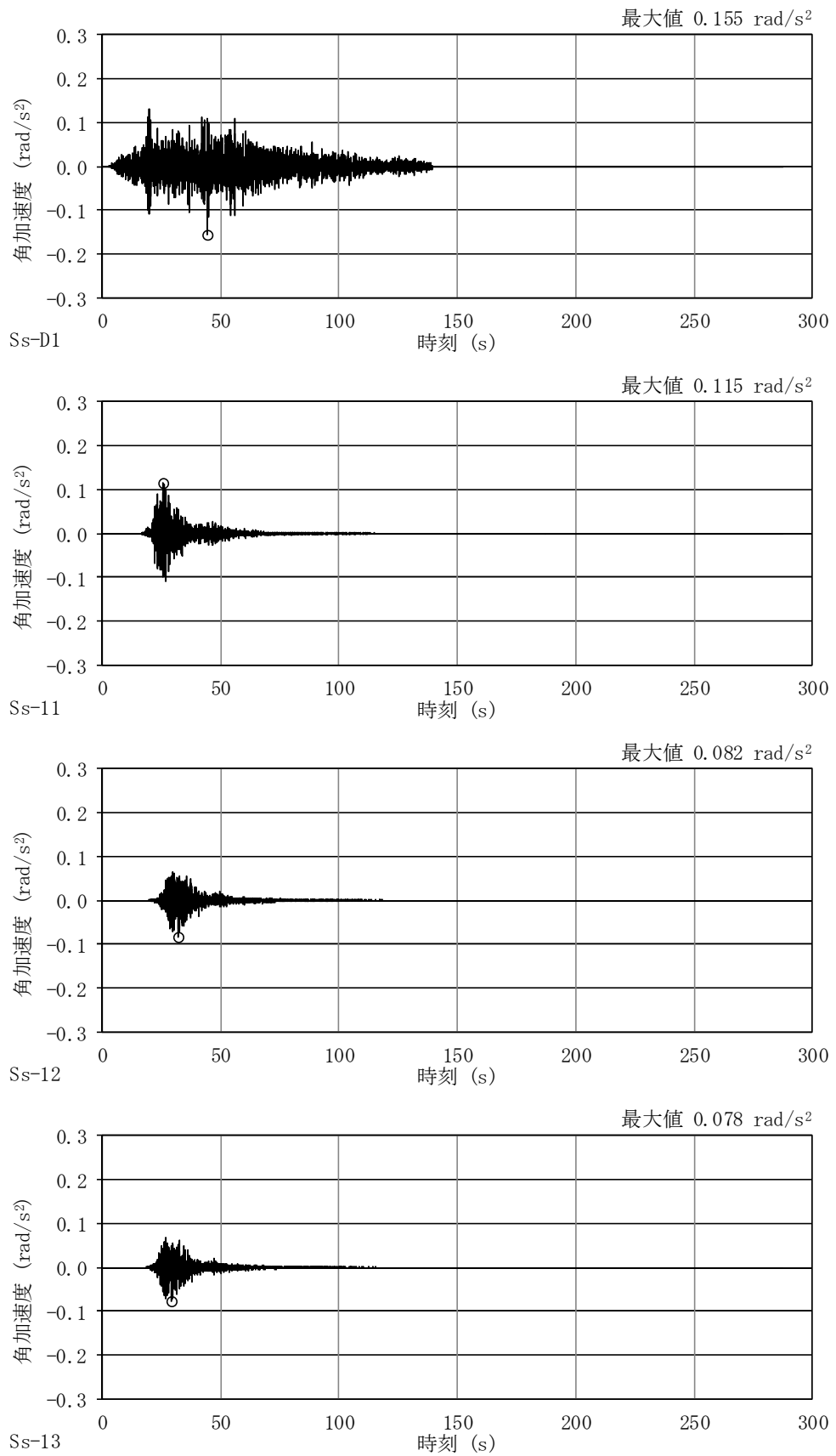
図 4-42 (1/2) 加速度時刻歴波形 (基準地震動 S s , EW 方向回転成分, 基本ケース)
