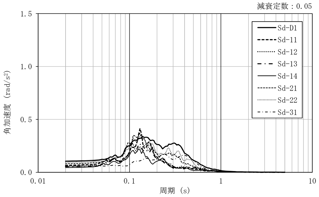
図 4-11 加速度応答スペクトル (弾性設計用地震動 S_d , EW 方向回転成分, 基本ケース)
