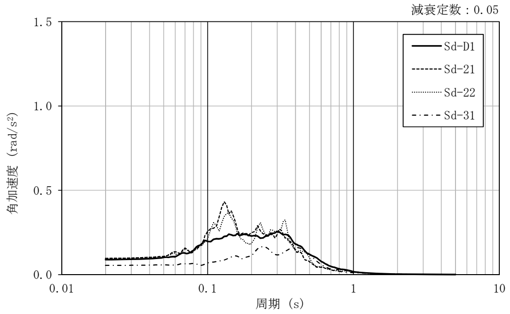
図 4-27 加速度応答スペクトル (弾性設計用地震動 S_a , NS 方向回転成分, 地盤物性のばらつきを考慮 ( -\sigma ))
