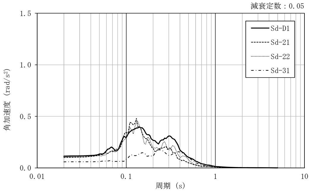
図 4-21 加速度応答スペクトル (弾性設計用地震動 S_a , EW 方向回転成分, 地盤物性のばらつきを考慮 (+ \sigma ))
