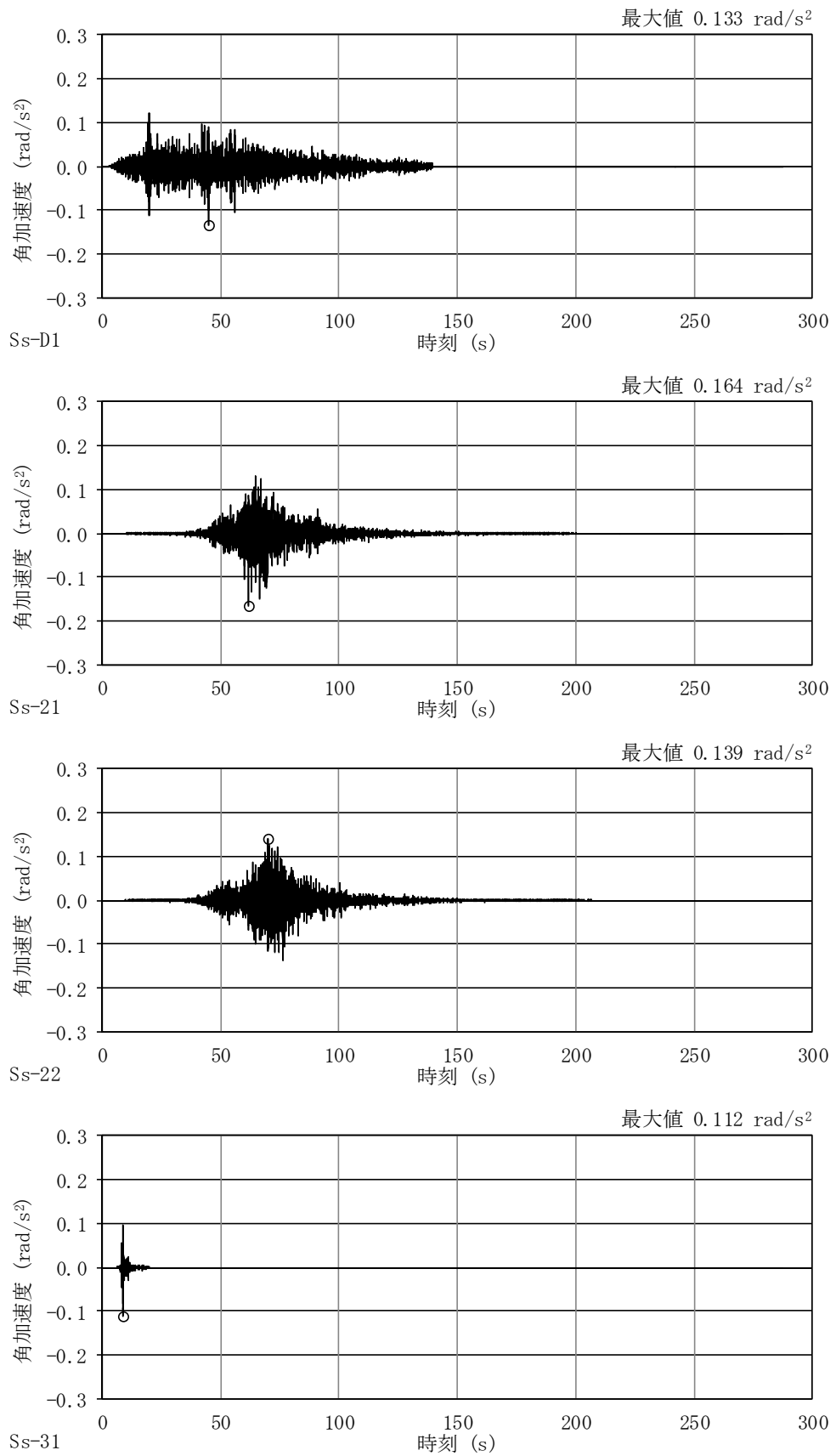
図 4-58 加速度時刻歴波形
