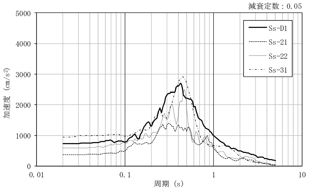
図 4-59 加速度応答スペクトル (基準地震動 S_s , EW 方向並進成分, 地盤物性のばらつきを考慮 ( -\sigma ))
