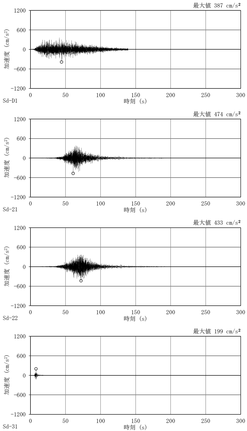
図 4-24 加速度時刻歴波形 (弾性設計用地震動 S d , UD 方向, 地盤物性のばらつきを考慮 (+σ))
