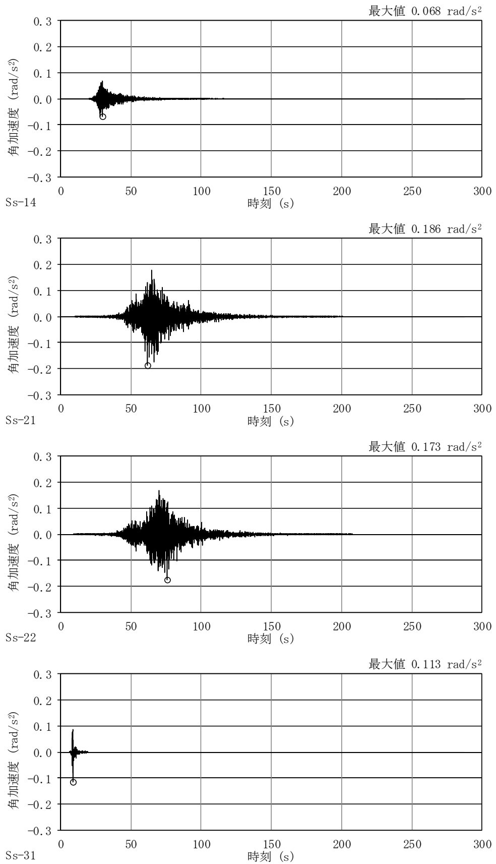
図 4-38 (2/2) 加速度時刻歴波形 (基準地震動 S_s , NS 方向回転成分, 基本ケース)
