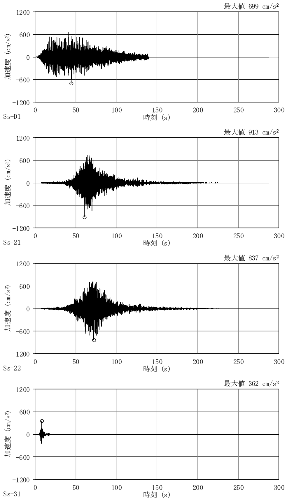
図 4-54 加速度時刻歴波形 (基準地震動 S_s , UD 方向, 地盤物性のばらつきを考慮 (+ \sigma ))
