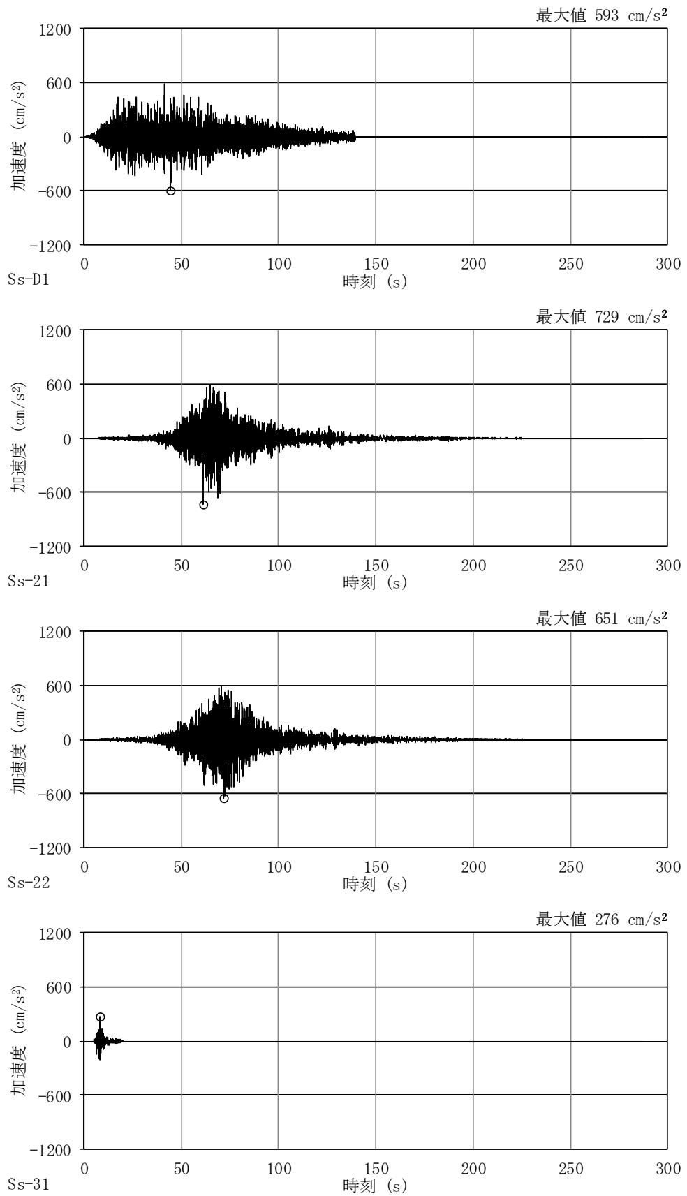
図 4-64 加速度時刻歴波形 (基準地震動 S_s , UD 方向, 地盤物性のばらつきを考慮 ( -\sigma ))
