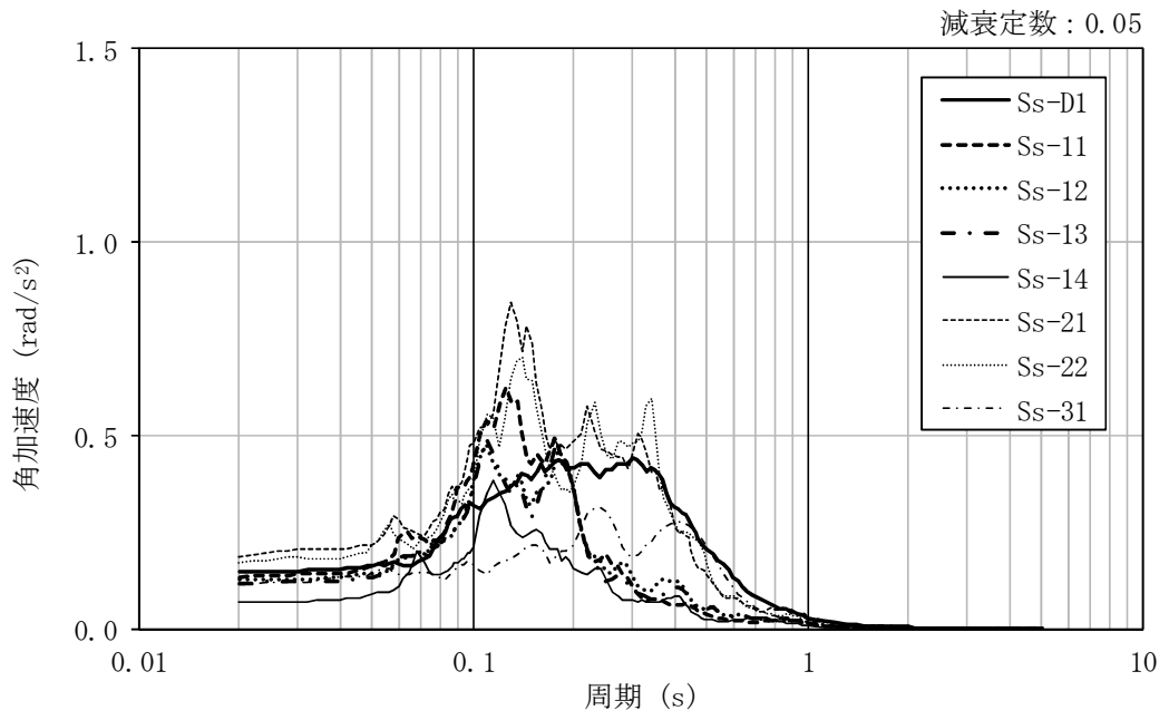
図 4-37 加速度応答スペクトル (基準地震動 S_s , NS 方向回転成分, 基本ケース)
