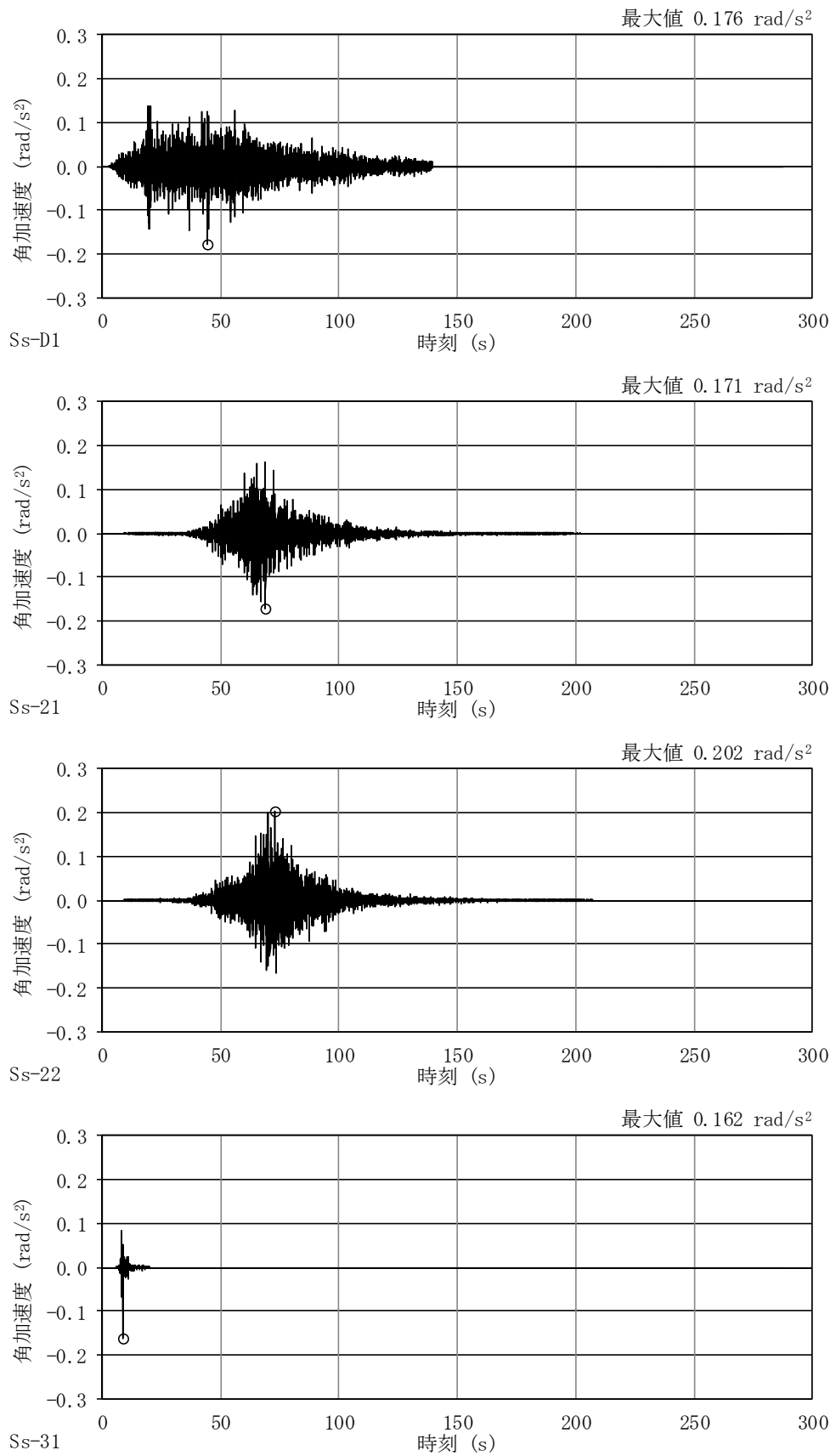
図 4-52 加速度時刻歴波形
