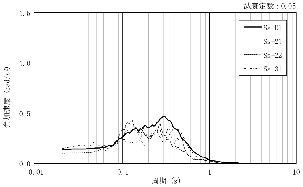
図 4-61 加速度応答スペクトル (基準地震動 S_s , EW 方向回転成分, 地盤物性のばらつきを考慮 ( -\sigma ))
