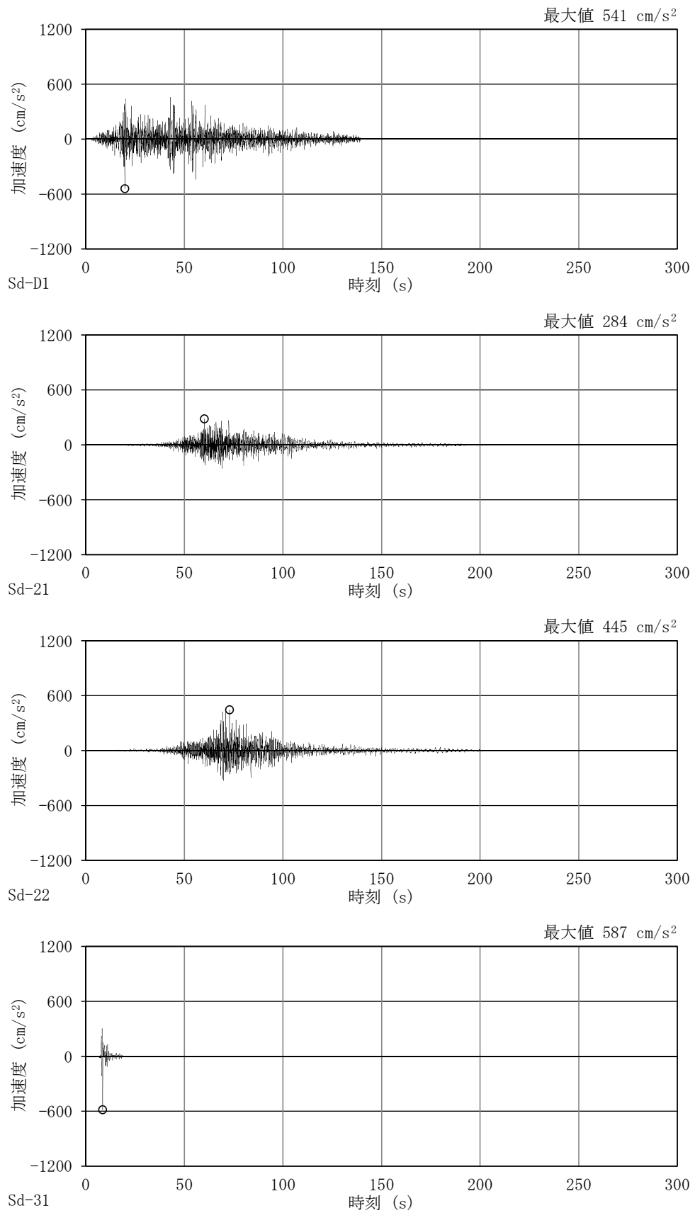
図 4-20 加速度時刻歴波形
