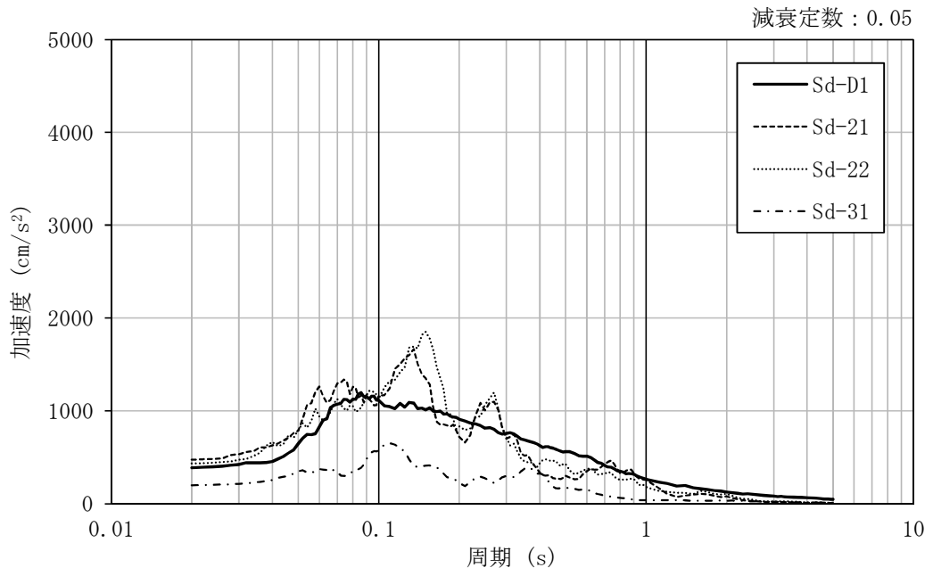
図 4-23 加速度応答スペクトル (弾性設計用地震動 S_a , UD 方向, 地盤物性のばらつきを考慮 (+ \sigma ))
