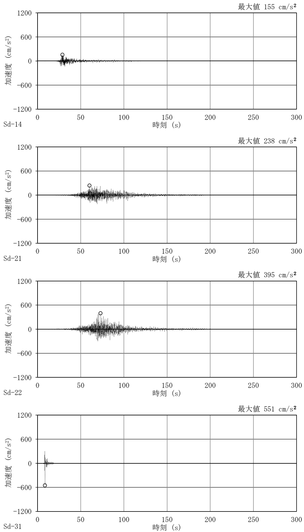
図 4-10 (2/2) 加速度時刻歴波形 (弾性設計用地震動 S_d , EW 方向並進成分, 基本ケース)
