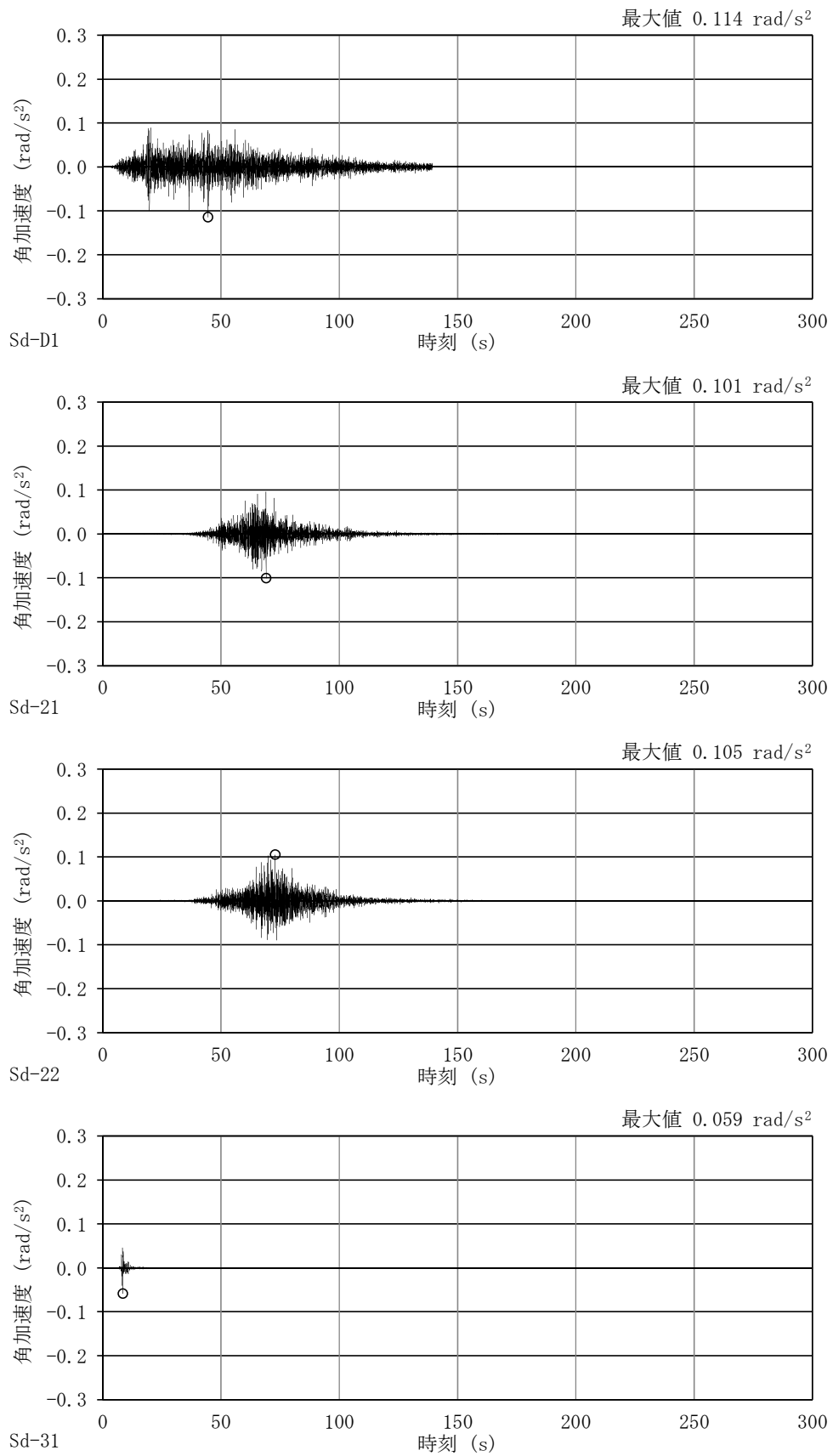
図 4-22 加速度時刻歴波形
