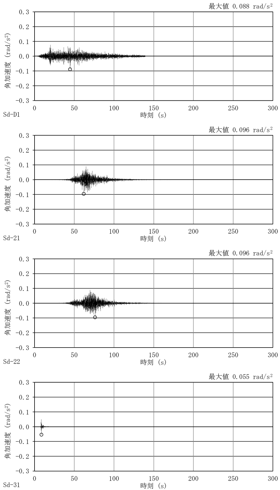
図 4-28 加速度時刻歴波形
