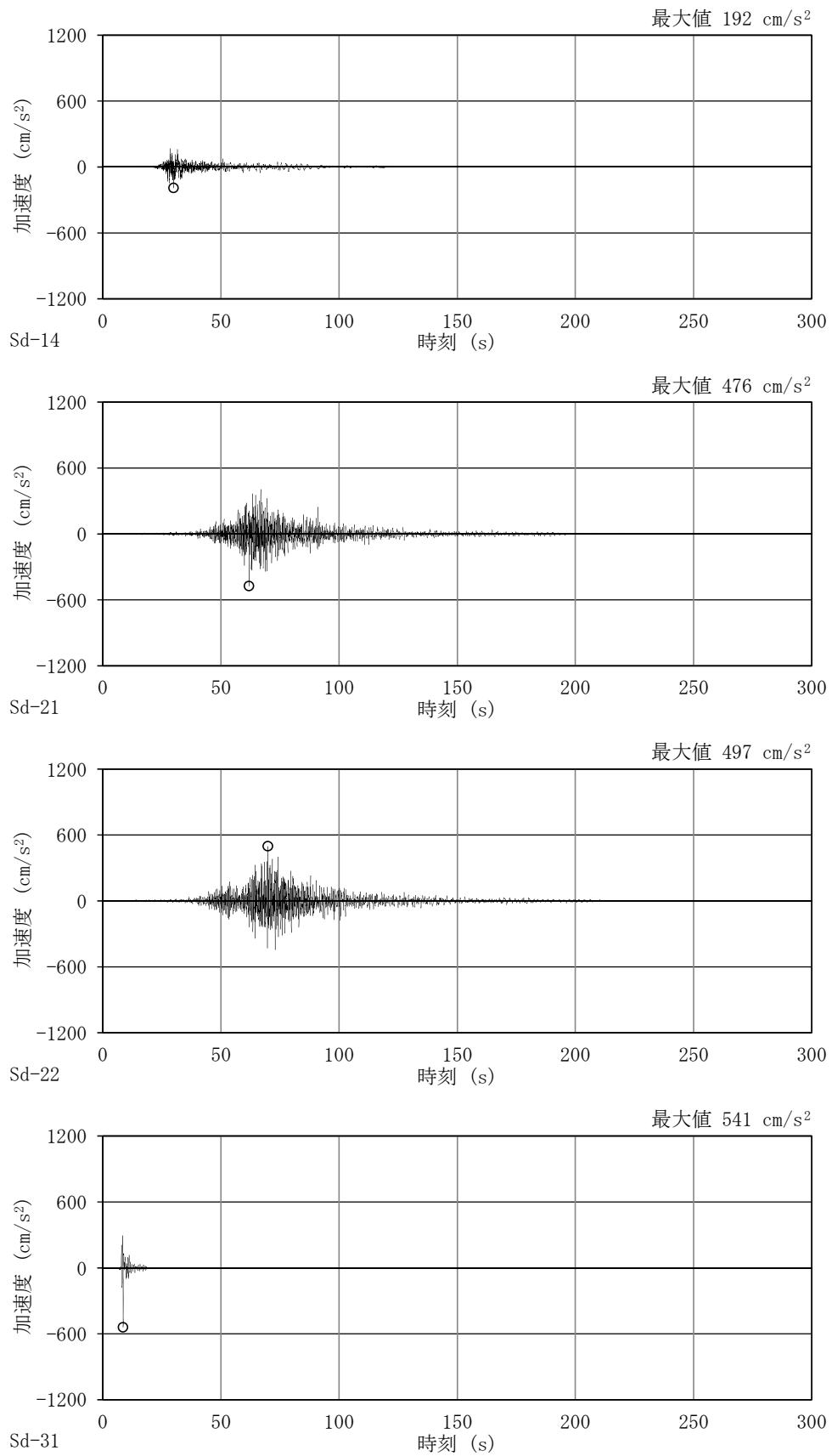
図 4-6 (2/2) 加速度時刻歴波形 (弾性設計用地震動 S_d , NS 方向並進成分, 基本ケース)
