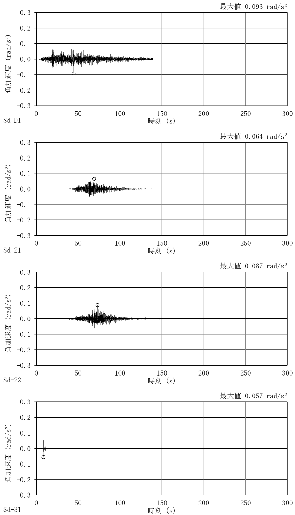
図 4-32 加速度時刻歴波形
