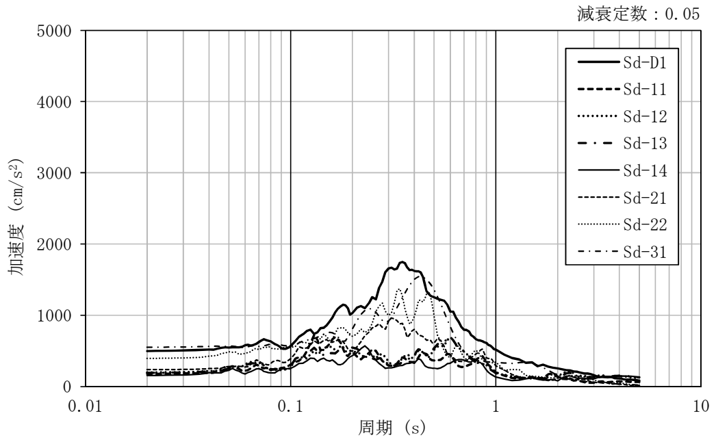
図 4-9 加速度応答スペクトル (弾性設計用地震動 S_d , EW 方向並進成分, 基本ケース)
