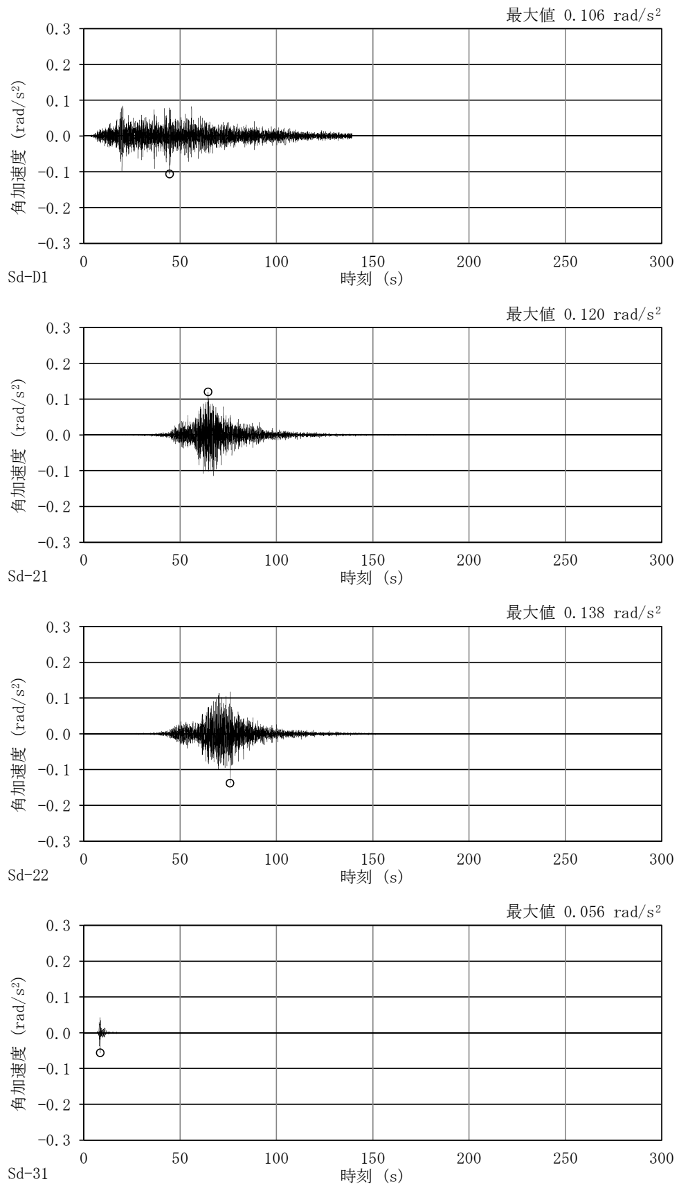
図 4-18 加速度時刻歴波形
