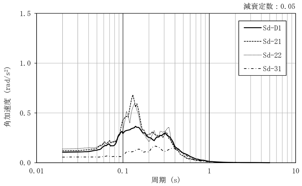
図 4-17 加速度応答スペクトル (弾性設計用地震動 S_a , NS 方向回転成分, 地盤物性のばらつきを考慮 (+ \sigma ))
