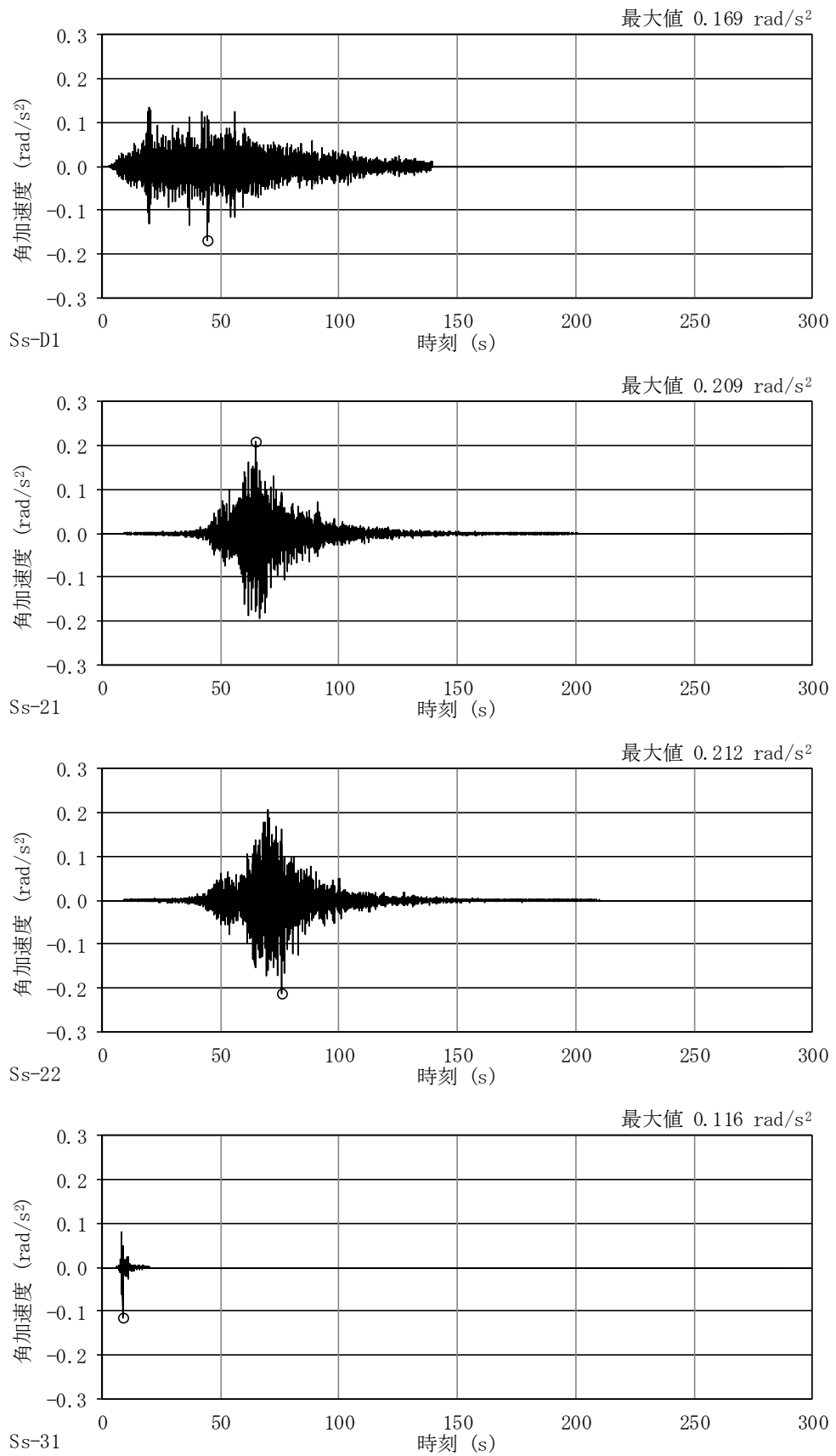
図 4-48 加速度時刻歴波形
