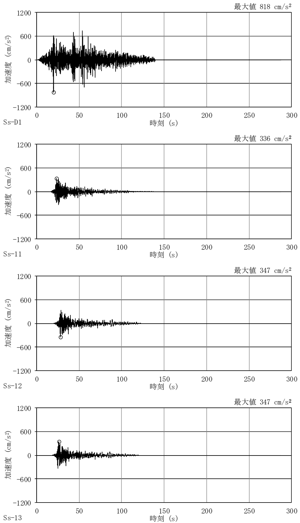
図 4-40 (1/2) 加速度時刻歴波形 (基準地震動 S s , EW 方向並進成分, 基本ケース)
