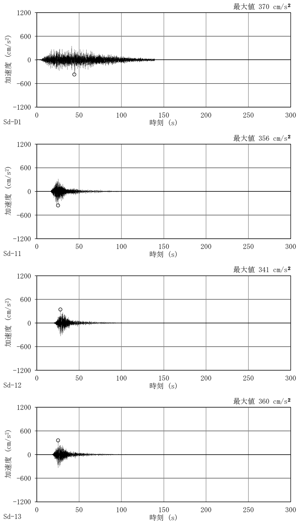
図 4-14 (1/2) 加速度時刻歴波形 (弾性設計用地震動 S_a , UD 方向, 基本ケース)
