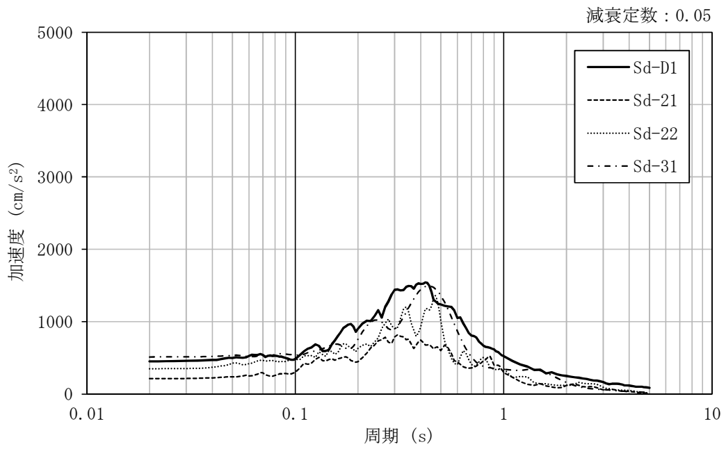
図 4-29 加速度応答スペクトル (弾性設計用地震動 S_a , EW 方向並進成分, 地盤物性のばらつきを考慮 ( -\sigma ))
