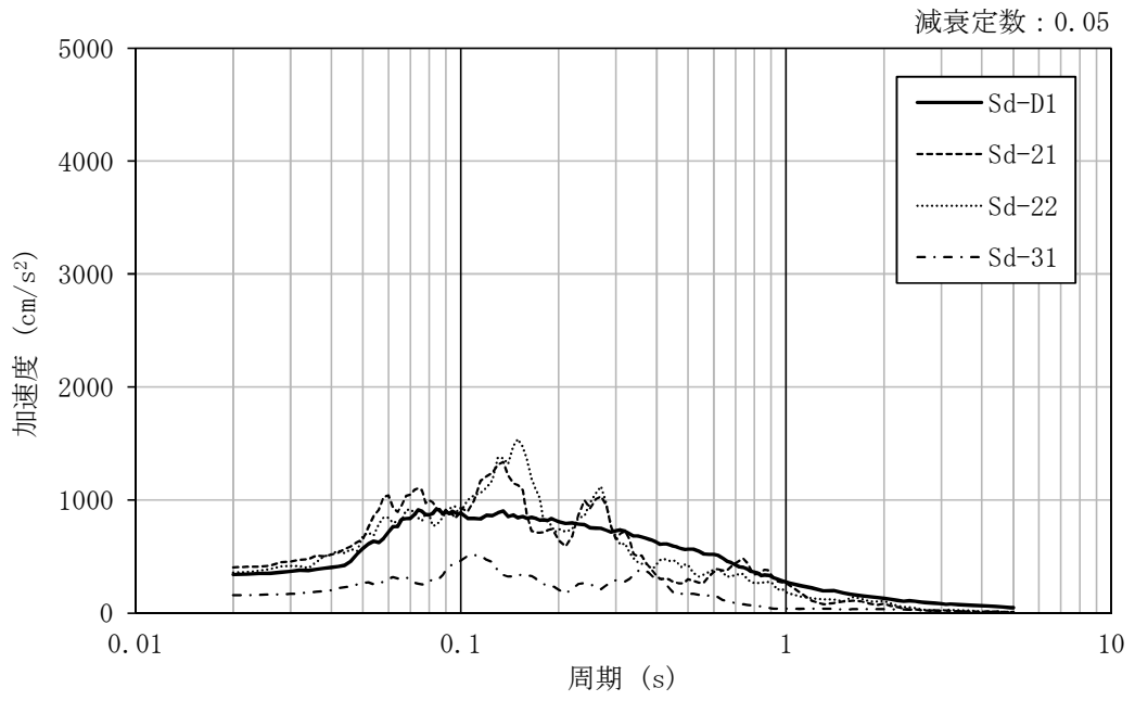
図 4-33 加速度応答スペクトル (弾性設計用地震動 S_a , UD 方向, 地盤物性のばらつきを考慮 ( -\sigma ))
