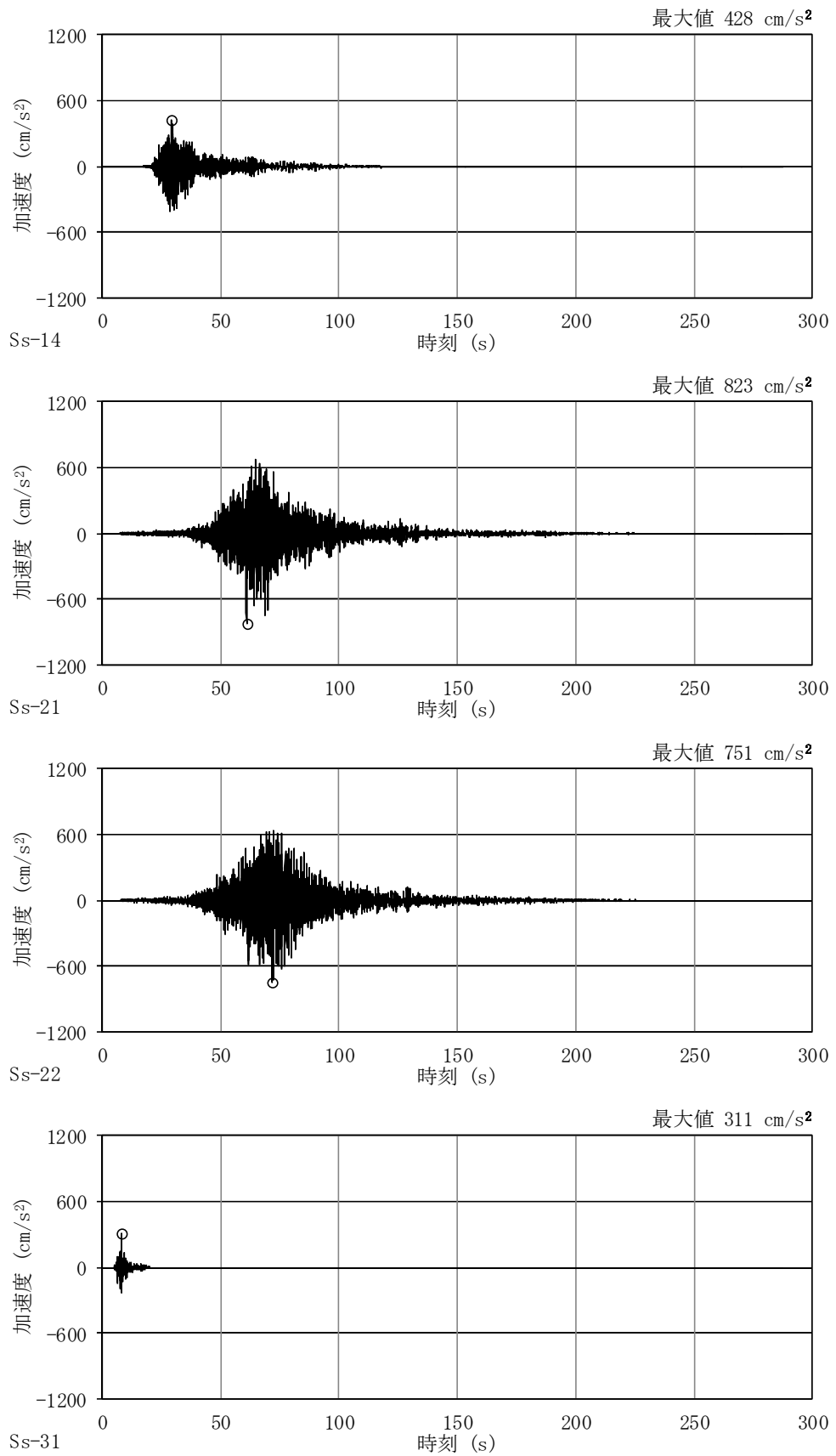
図 4-44 (2/2) 加速度時刻歴波形 (基準地震動 S s , UD 方向, 基本ケース)
