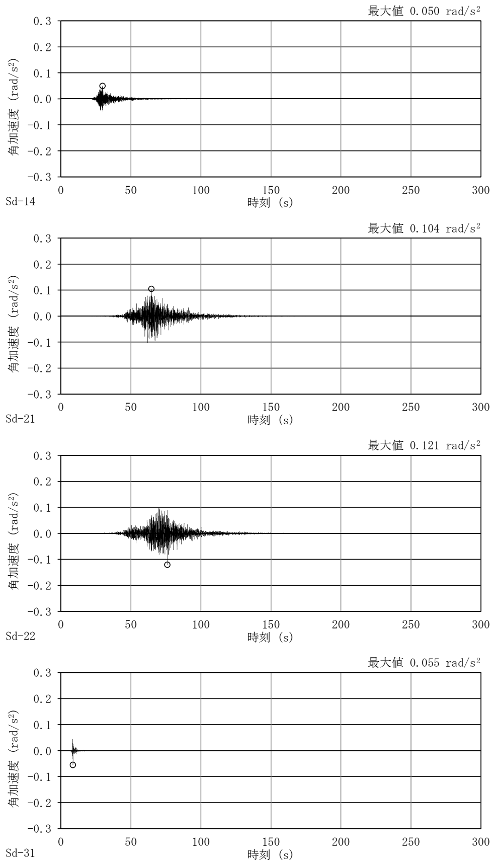
図 4-8 (2/2) 加速度時刻歴波形 (弾性設計用地震動 S_d , NS 方向回転成分, 基本ケース)
