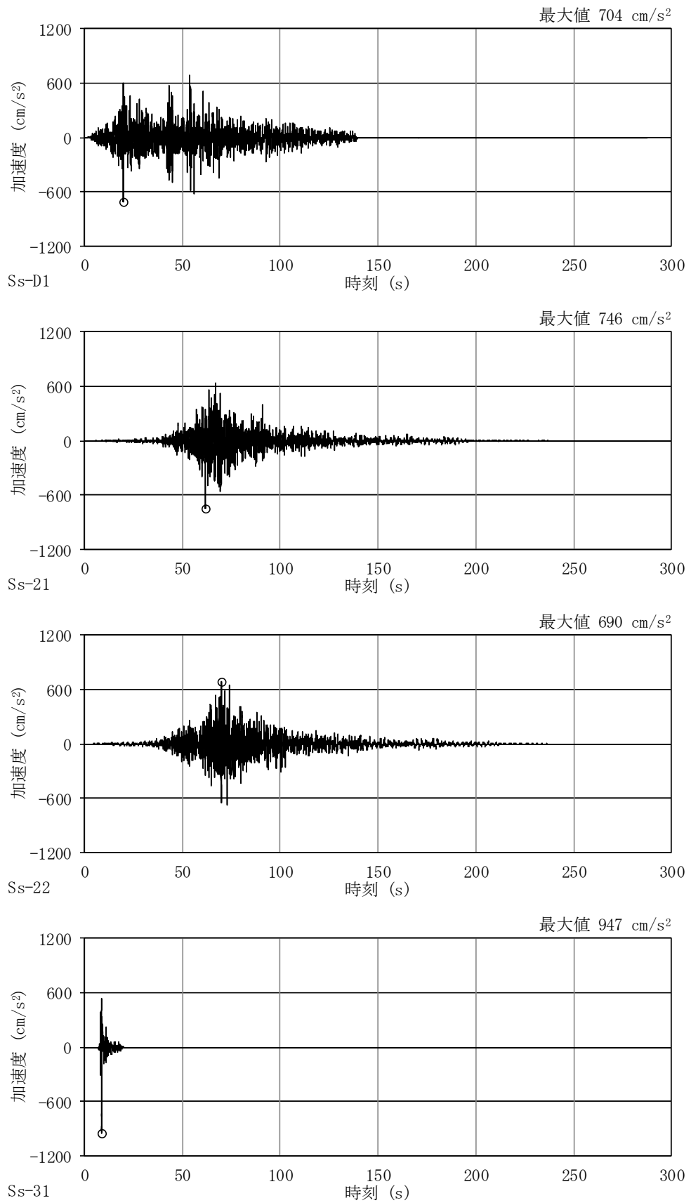
図 4-56 加速度時刻歴波形
