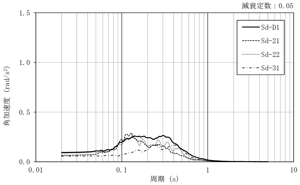
図 4-31 加速度応答スペクトル (弾性設計用地震動 S_a , EW 方向回転成分, 地盤物性のばらつきを考慮 ( -\sigma ))
