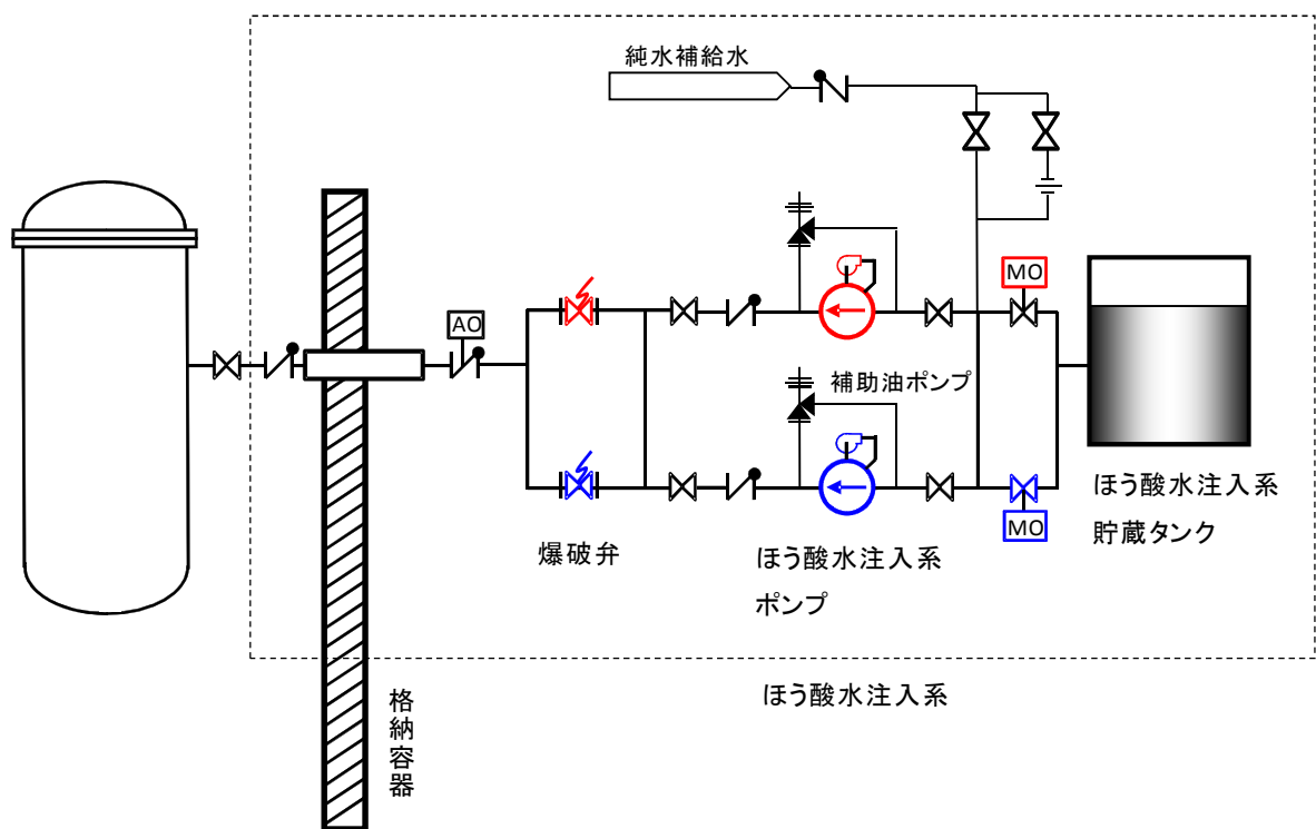
第1図 ほう酸水注入系概略系統図
