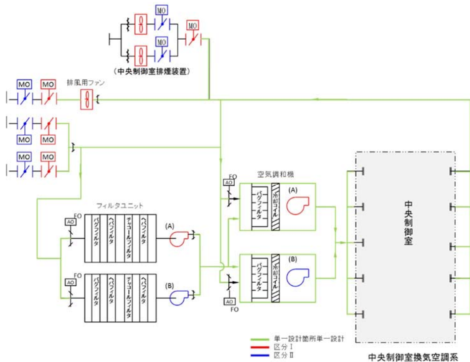
第20-1図 中央制御室換気系 系統概略図
