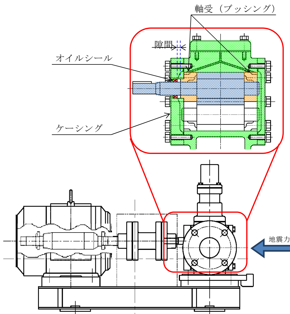
第 10 図 ギヤ式ポンプの標準的な構造概要図
