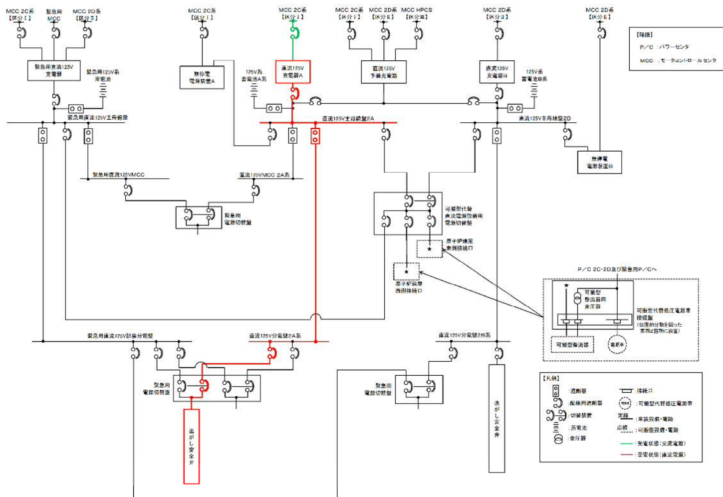
第5図 代替交流電源設備による復旧（可搬型代替交流電源設備を使用）（2／2）
