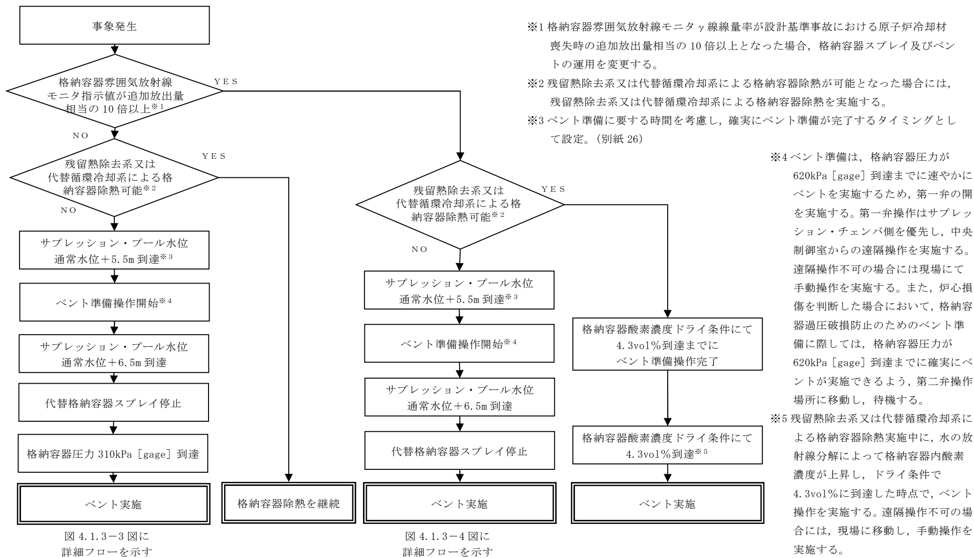
第 4.1.3-2 図 ベント実施の判断フロー
