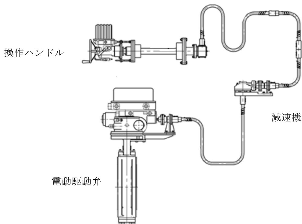
第 48-6-3 図 遠隔人力操作機構外形図
