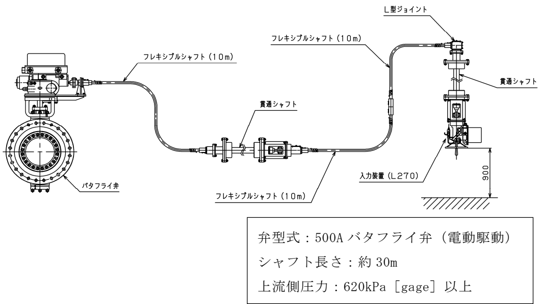
第 3 図 モックアップ試験の概要 (1/2)
