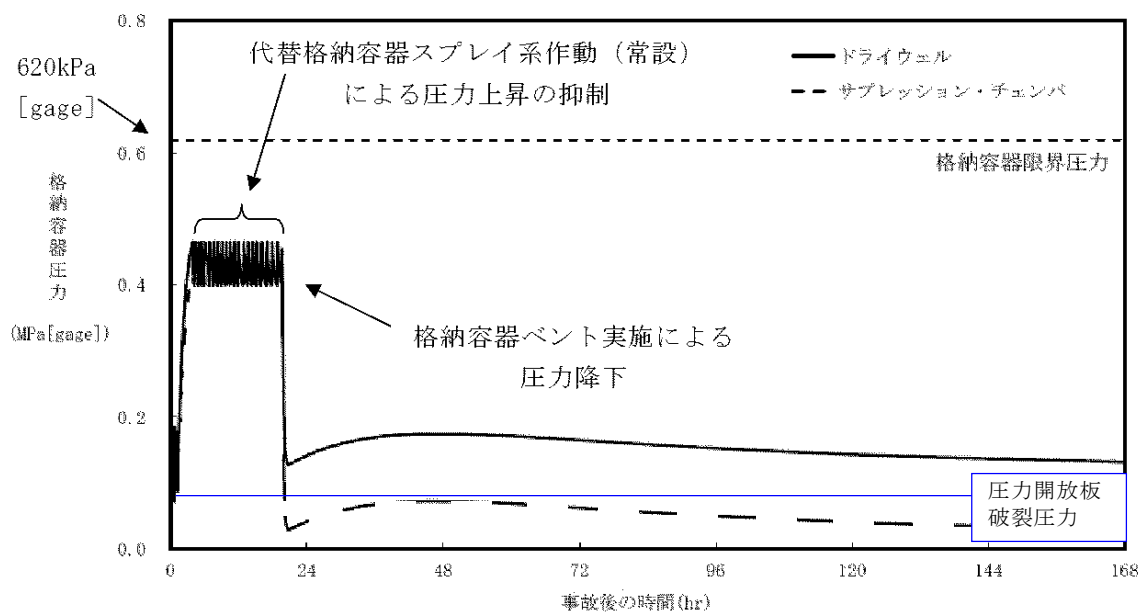
第 50－6－4 図 「雰囲気圧力・温度による静的負荷（格納容器過圧・過温破損）（代替循環冷却を使用しない場合）」における格納容器圧力の推移と圧力開放板破裂圧力の関係
