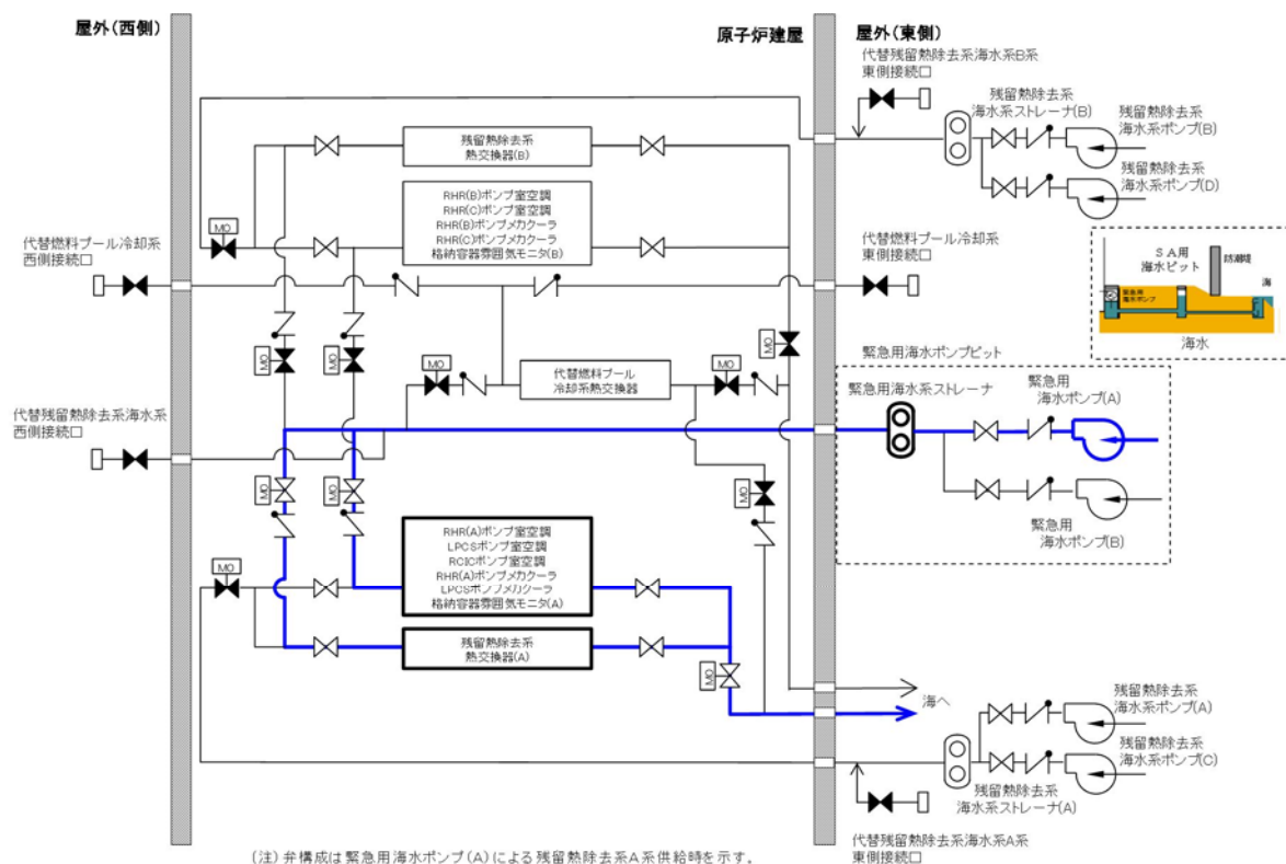
第 48-6-4 図 緊急用海水系運転性能検査系統図
