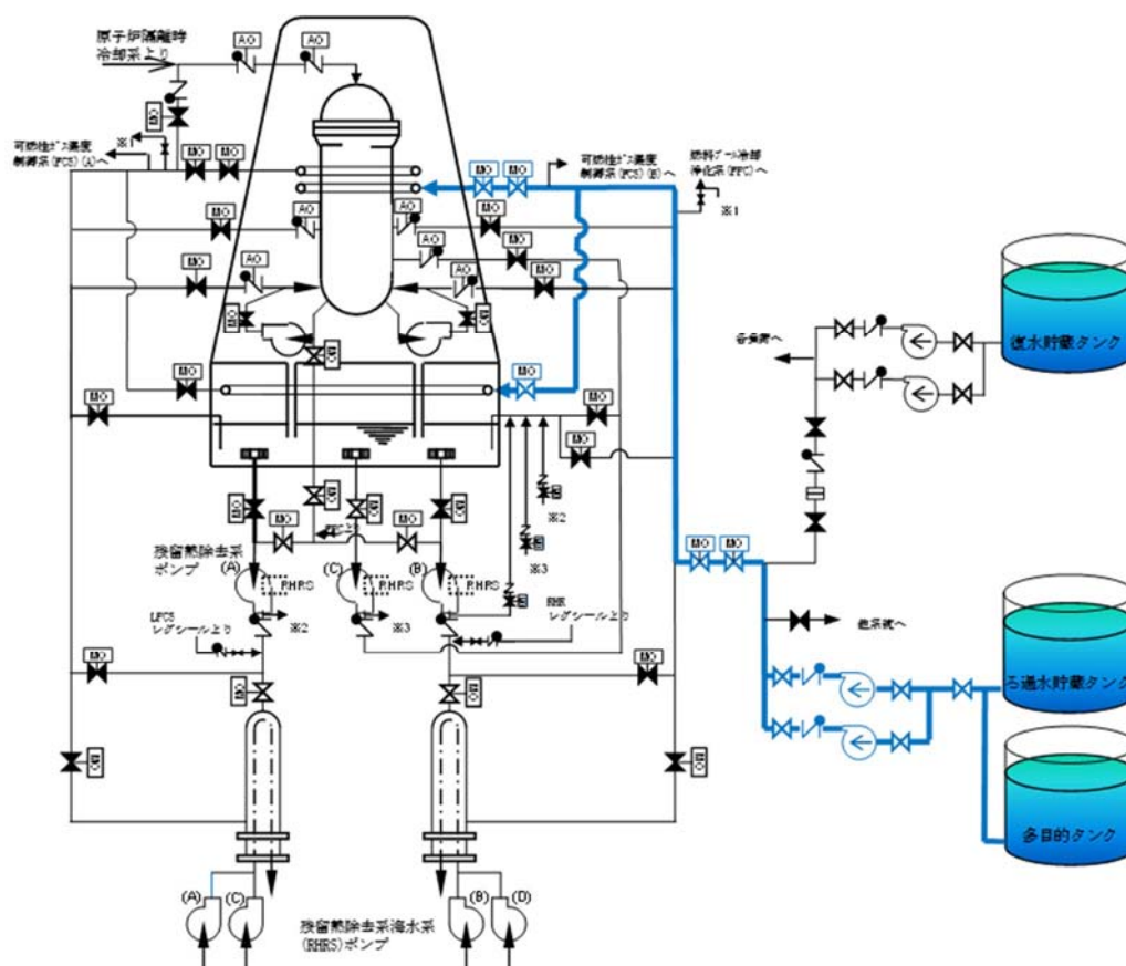
第49-10-1図 消火系による原子炉格納容器スプレー手順の概要図
