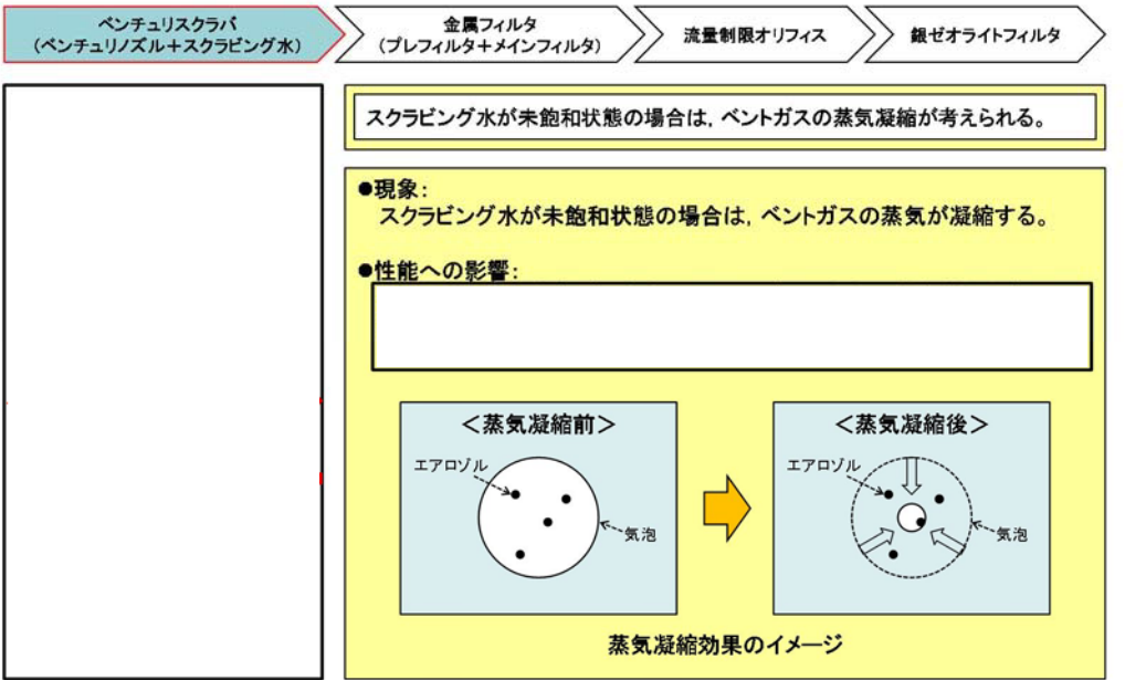
フィルタ装置機能模式図
