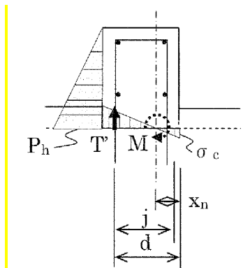
第 5-15 図 堰に生じる圧縮力の概念図
