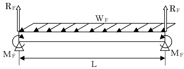
第5-10-2図 梁材及び柱材に生じる力の模式図 (2/2)
