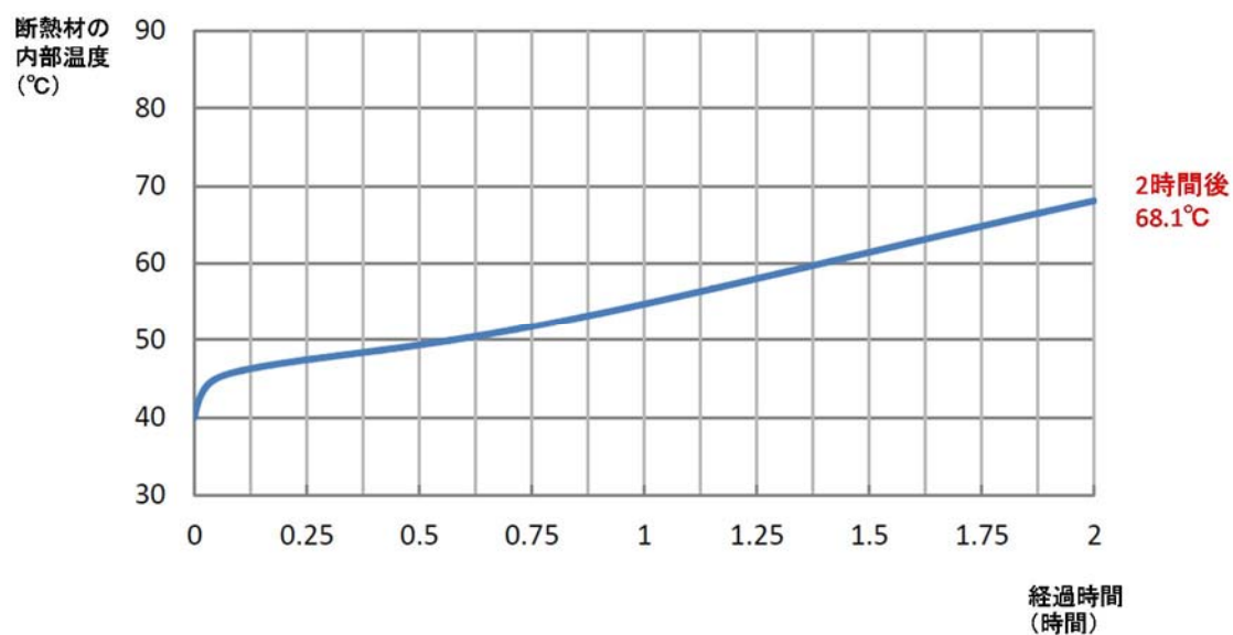
第 4 図 格納容器内水素濃度 (S A) 及び格納容器内酸素濃度 (S A) の断熱材厚さの評価結果 (断熱材外側 : 100°C ・ 2 時間, 断熱材厚さ 80mm の場合)
