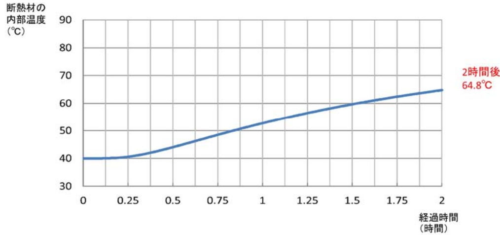
第2図 非常用窒素供給系高圧窒素ポンベ及び非常用逃がし安全弁駆動系高圧窒素ポンベの断熱材厚さの評価結果（断熱材外側： 100^{\circ}\text{C} \cdot 2 時間，断熱材厚さ 50\text{mm} の場合）
