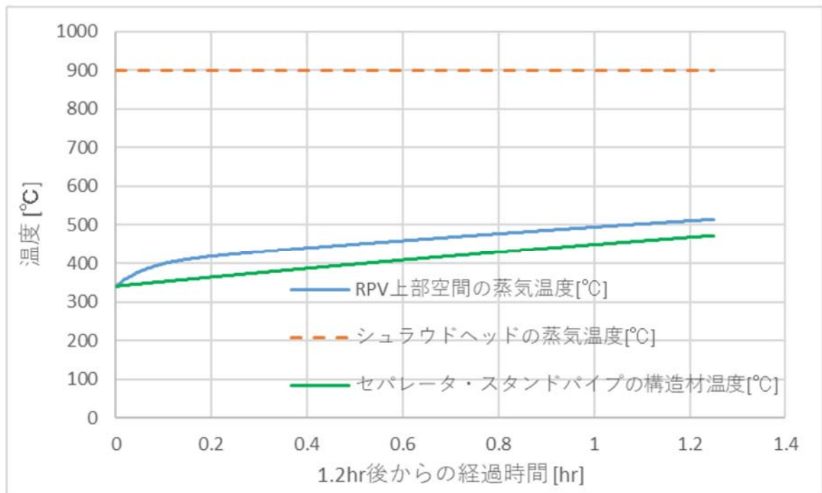
図3 簡易評価による原子炉圧力容器の上部ヘッ드의気相温度及びスタンドパイプ／セパレータの構造材温度
