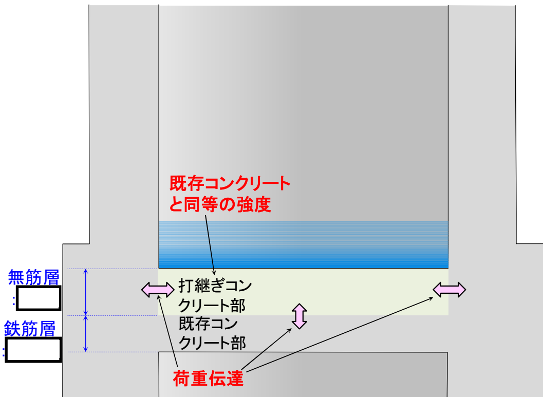
第2図 強度維持のために必要な事項について
