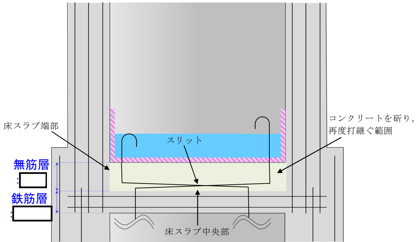
第1図 対策後のペDESTAL概要図
