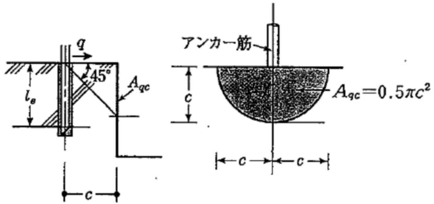
第 4 図 側面の有効投影面積
