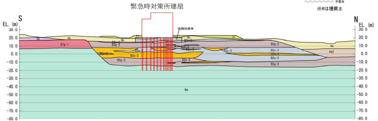
(3) 緊急時対策所周辺断面 (C-C 断面)
