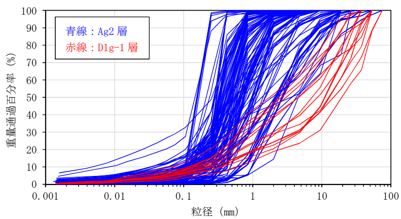
図8 D1g-1層とAg2層の粒度分布の比較
