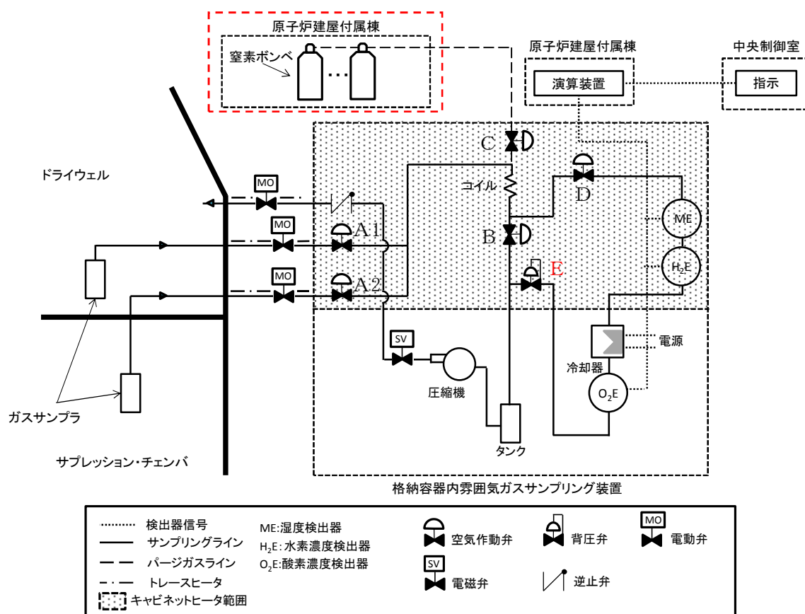
図 1-3-1 格納容器内雰囲気ガスサンプリング装置の構成 (通常待機状態)
