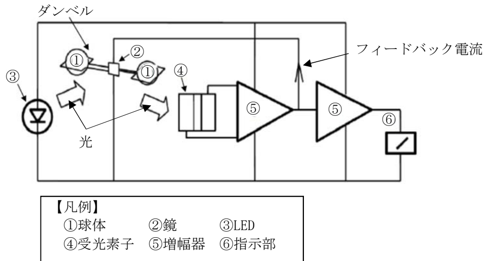
図 1-2-2-2 格納容器内酸素濃度（S A）検出回路図
