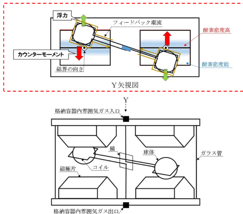
図 1-2-2-1 格納容器内酸素濃度（S A）の概要図
