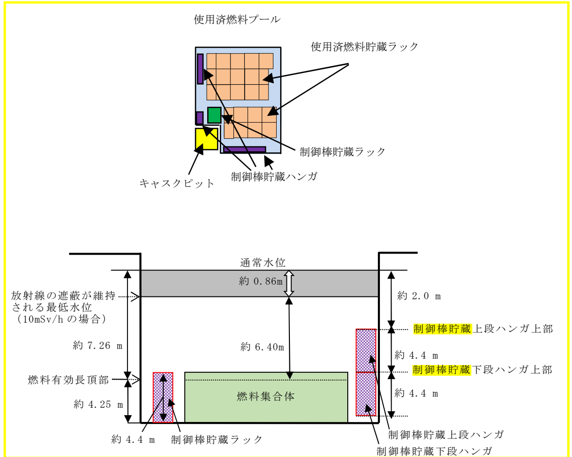
第 3-1 図 使用済燃料プール概要図
