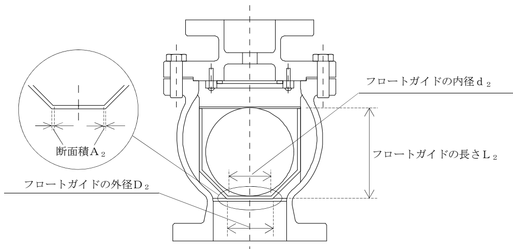
図 5-2 フロートガイドの応力評価に用いる長さ、外径、内径及び断面積
