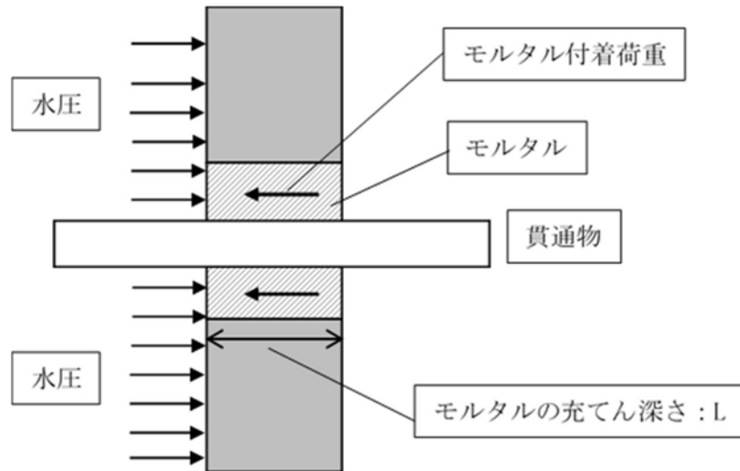
第5-19図 荷重模式図
