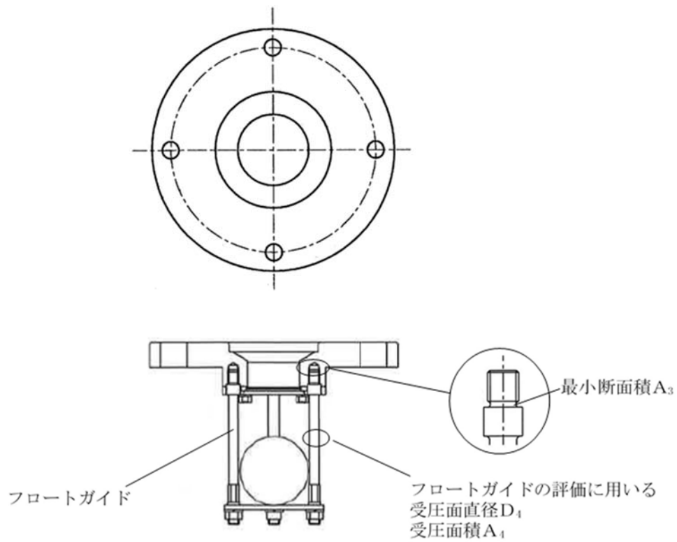
第5-17図 フロートガイドの強度評価に用いる受圧面直径及び断面積
