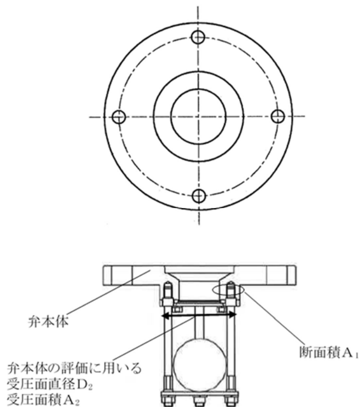
第 5-16 図 弁本体の強度評価に用いる受圧面直径及び断面積
