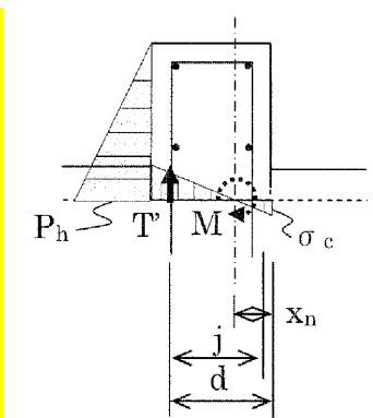
第 5-15 図 堰に生じる圧縮力の概念図
