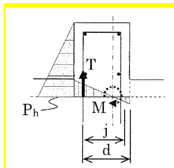
第 5-14 図 堰に生じる引張力の概念図
