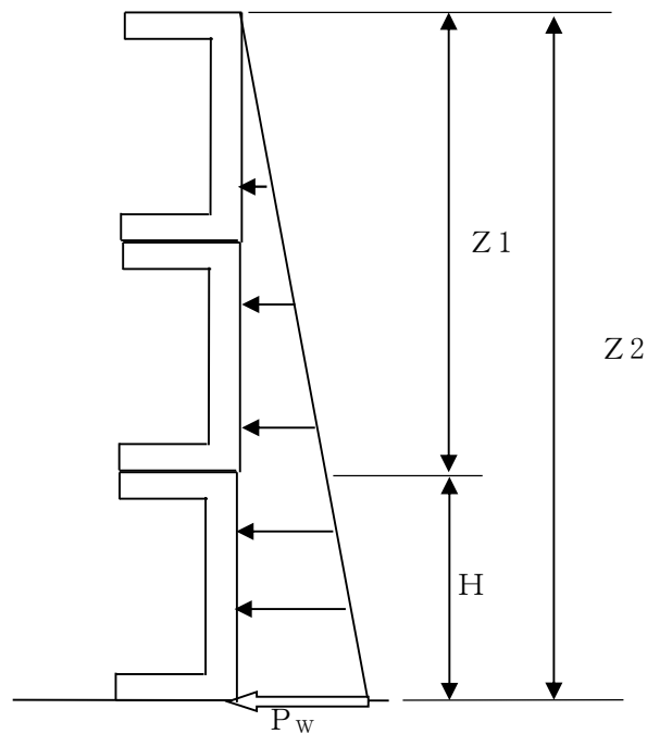
第5-10-1図 梁材及び柱材に生じる力の模式図 (1/2)
