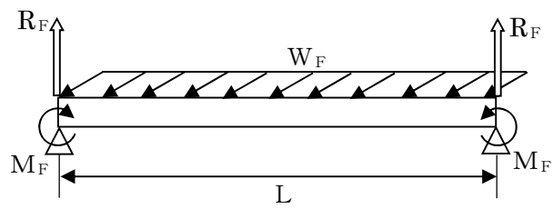
第5-10-2図 梁材及び柱材に生じる力の模式図 (2/2)
