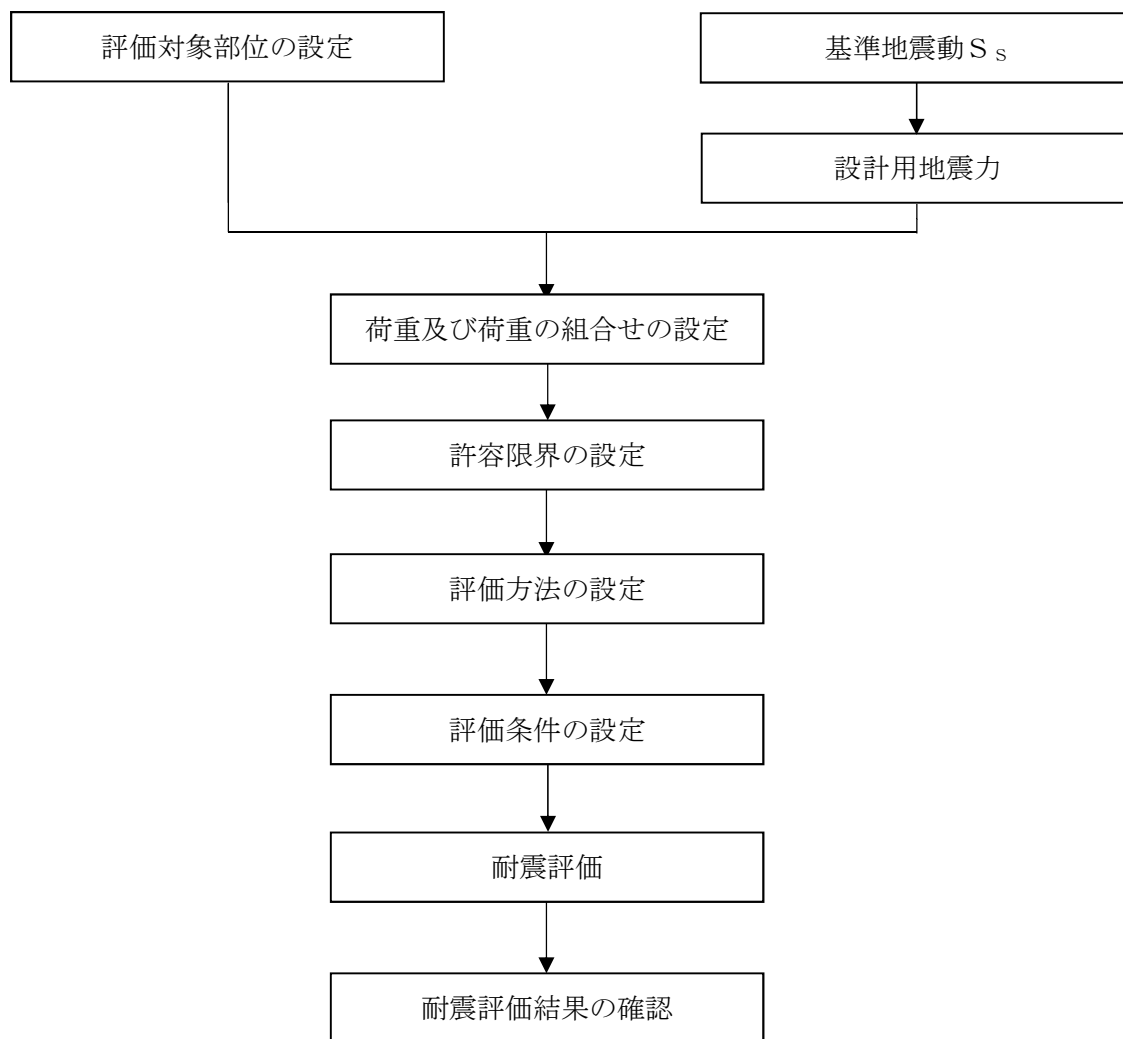
第2-16図 堰の耐震評価フロー
