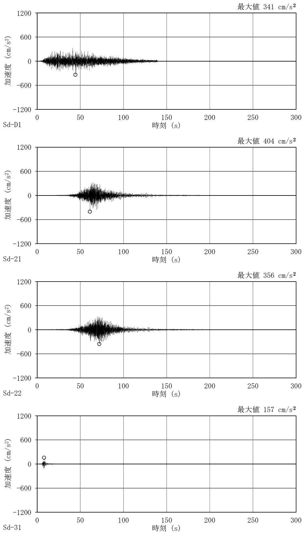
図 4-35 加速度時刻歴波形
