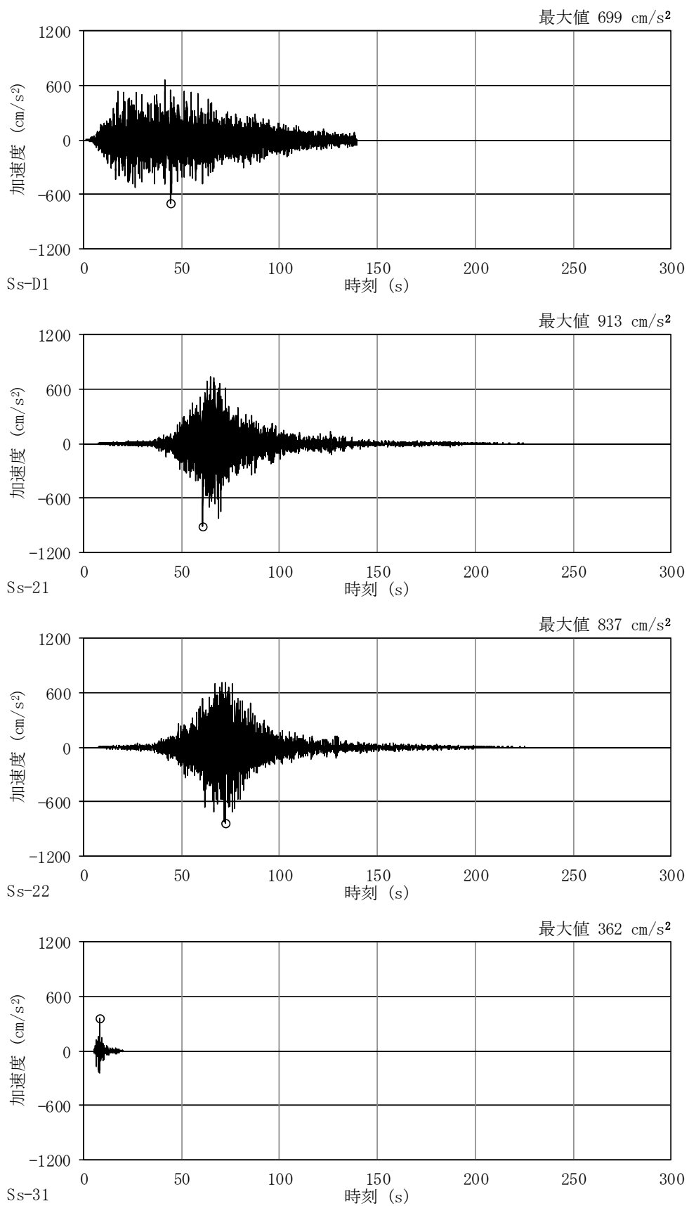
図 4-55 加速度時刻歴波形 (基準地震動 S s , UD 方向, 地盤物性のばらつきを考慮 (+σ))
