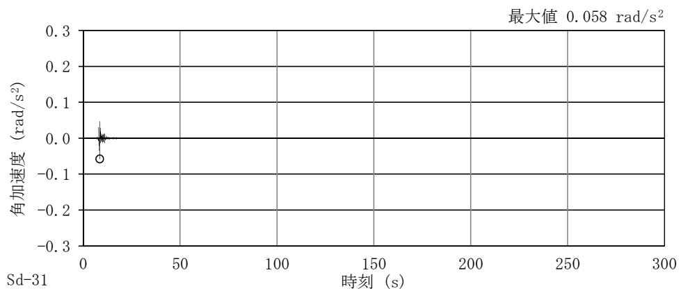
図 4-13 (2/2) 加速度時刻歴波形 (弾性設計用地震動 S d , EW 方向回転成分, 基本ケース)
