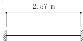
図4-6 解析モデル（屋根スラブ）
