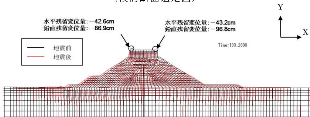
(残留変位図 (傾斜堤: ①-①断面))
