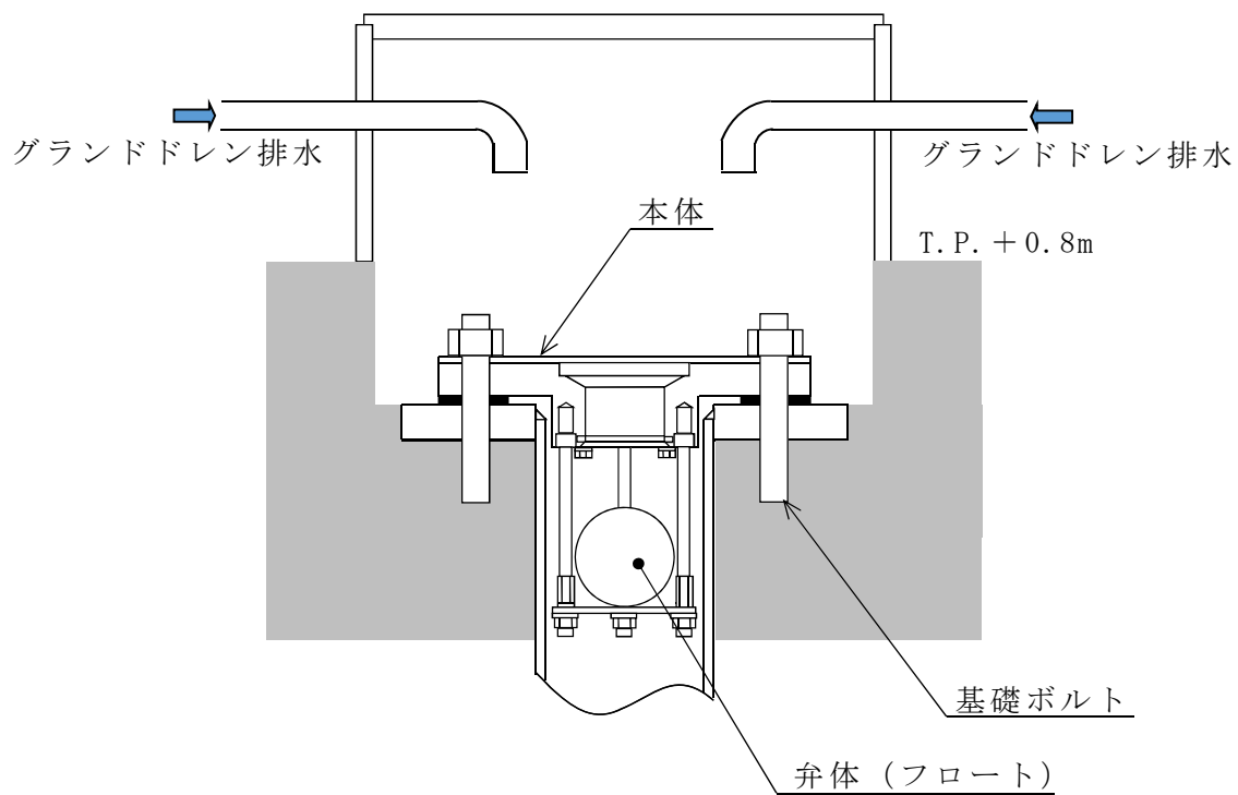
第 10.6-14 図 緊急用海水ポンプグラウンドドレン排出口逆止弁 概念図
