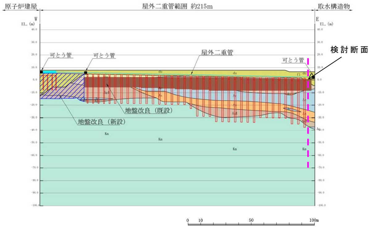
第 8 図 検討断面位置図
