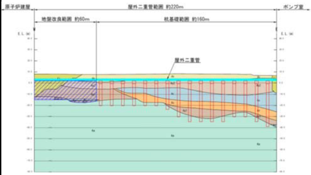
基礎縦断配置図
