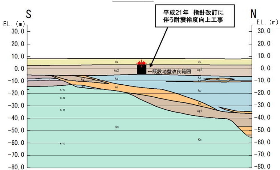
D-D 断面
