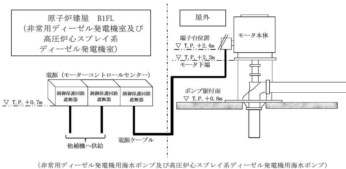
第 2.3-13 図 非常用海水ポンプの位置関係図
