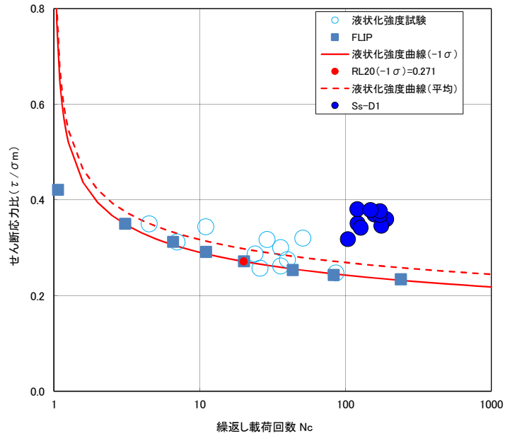
(a) 試験データの -1 \sigma 保守側の回帰曲線を再現対象とした FLIP の液状化強度特性
