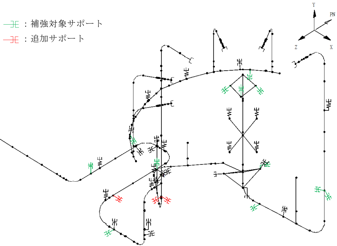
原子炉再循環系配管の耐震補強の例
