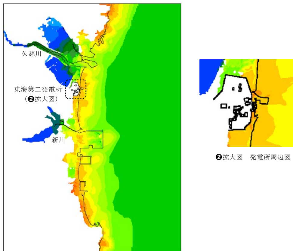
第 1.3-3 図 基準津波による発電所周辺の広域の最大水位上昇量分布図
