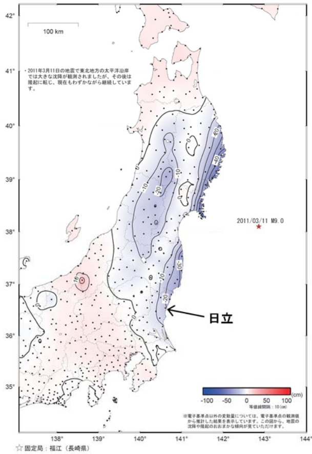
東北地方太平洋沖地震 (M9.0) 前後の地殻変動 (上下) 一本震前から6年間の累積
