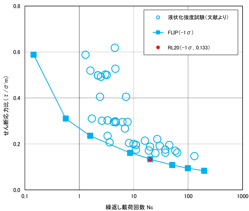
第 7.1.2 図 FLIPによる豊浦標準砂の 液状化強度特性 (-1 \sigma )
