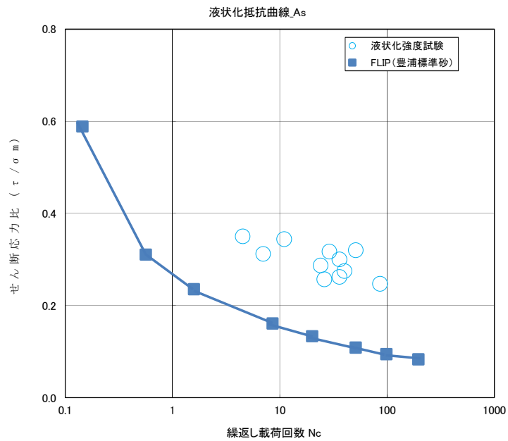
(b) 全ての試験データを包含する 豊浦標準砂の FLIP の液状化強度特性 第 4.4.5 図 累積損傷度理論に基づく評価結果 (取水口・海水ポンプ室, As 層)
