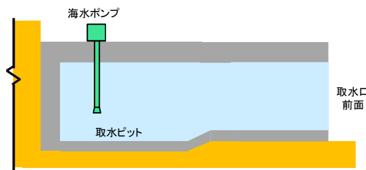
取水口概念図
