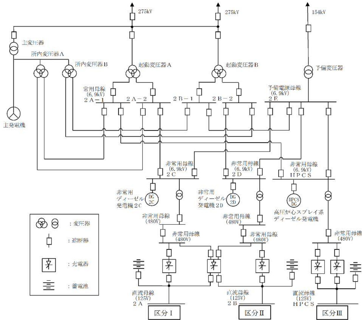
第 3.1.1.1-11 図 電源システムの概要図
