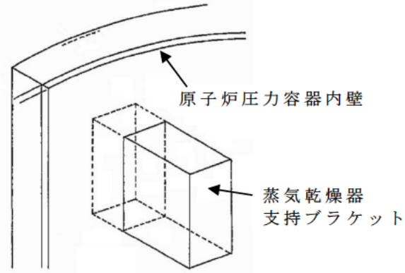
蒸気乾燥器支持ブラケット構造図
