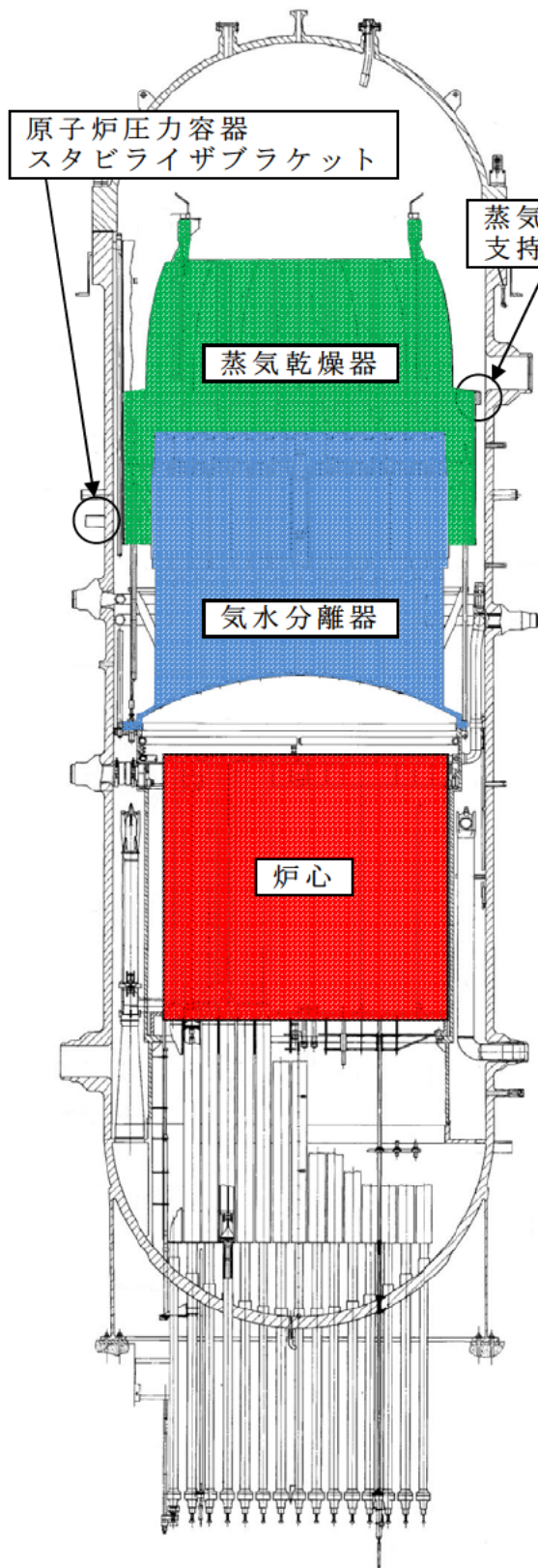
第2図 原子炉圧力容器（蒸気乾燥器支持ブラケット， 原子炉圧力容器スタビライザ）の概要図
