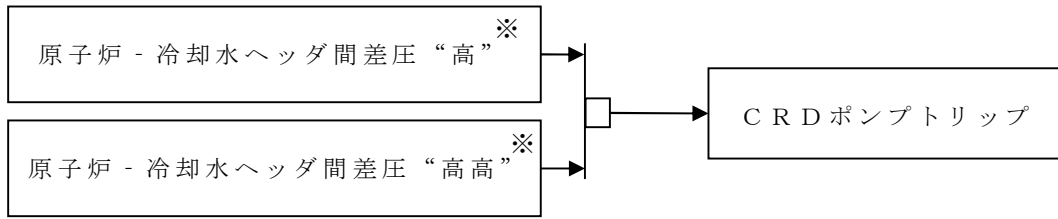
図 2 制御棒駆動水圧系ポンプの自動トリップインターロック
