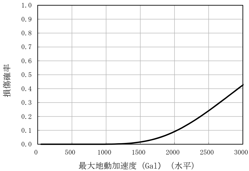
第 3.2.1.3-3-5 図 残留熱除去系熱交換器 (アンカボルト)
