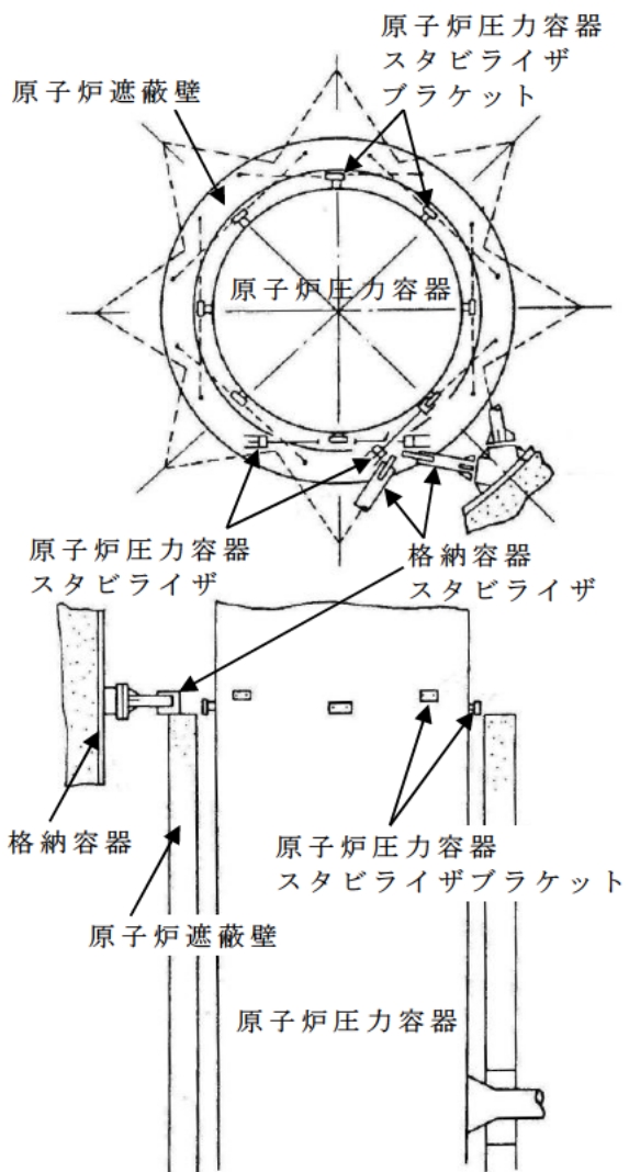
原子炉圧力容器スタビライザ構造図
