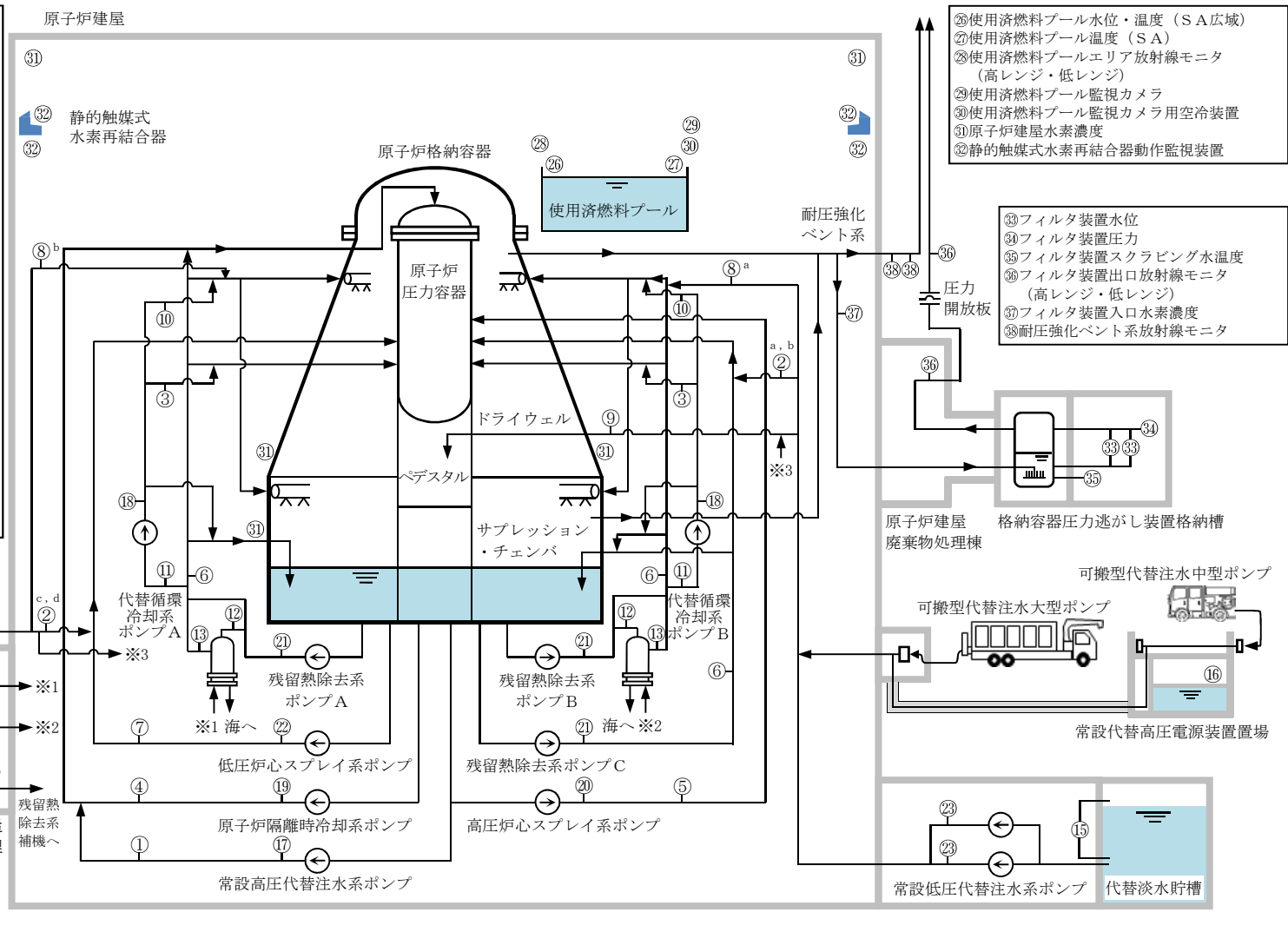
第 1.15-3 図 主要設備 系統概要図 (1/3)
