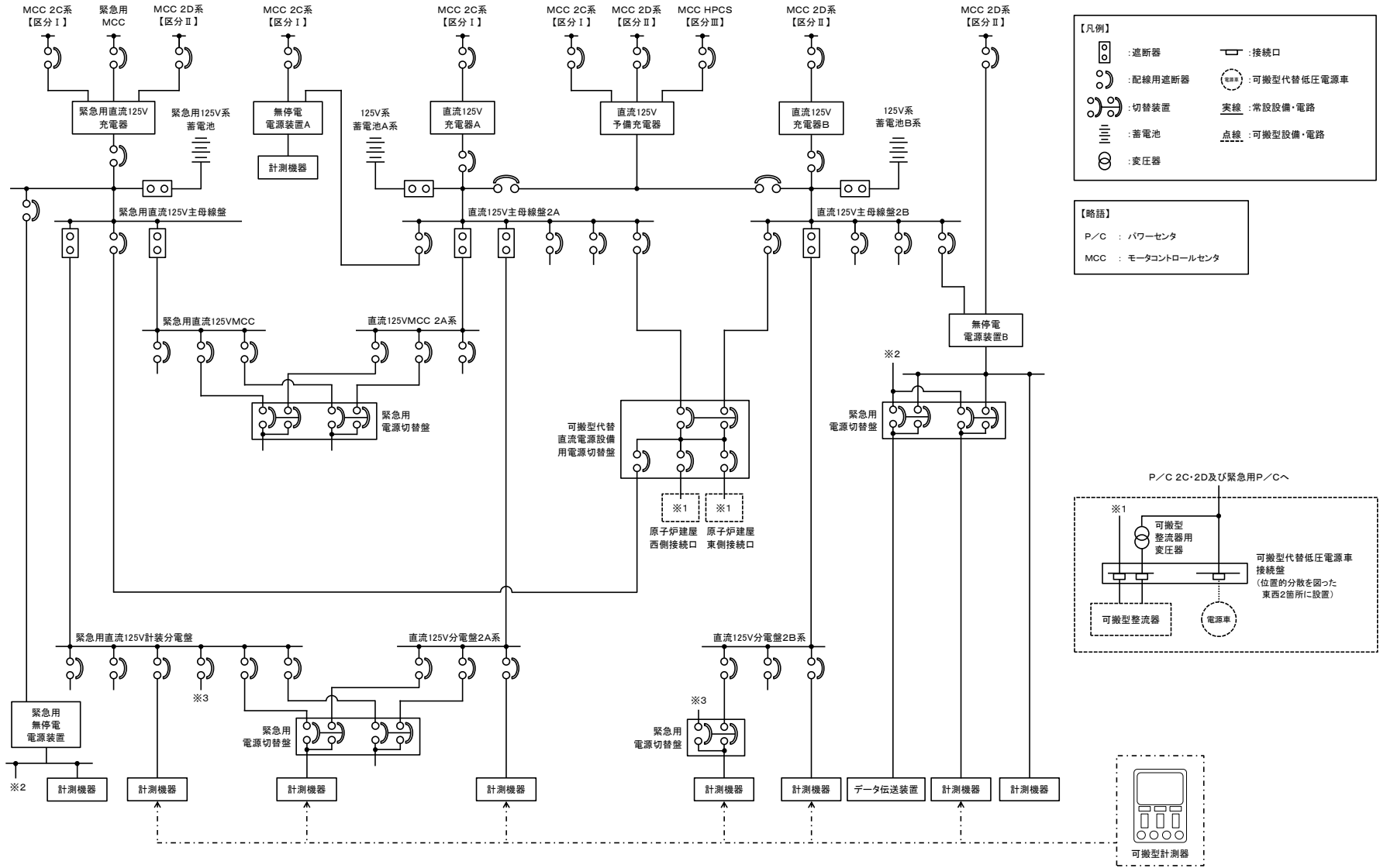
第 1.15-4 図 計器の電源構成図 (直流電源) (1/3)
