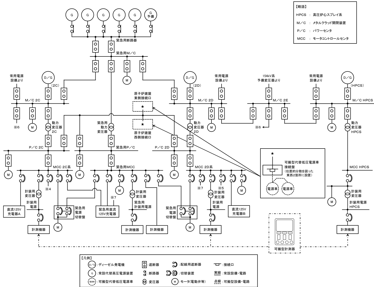
第 1.15-4 図 計器の電源構成図 (交流電源) (3/3)
