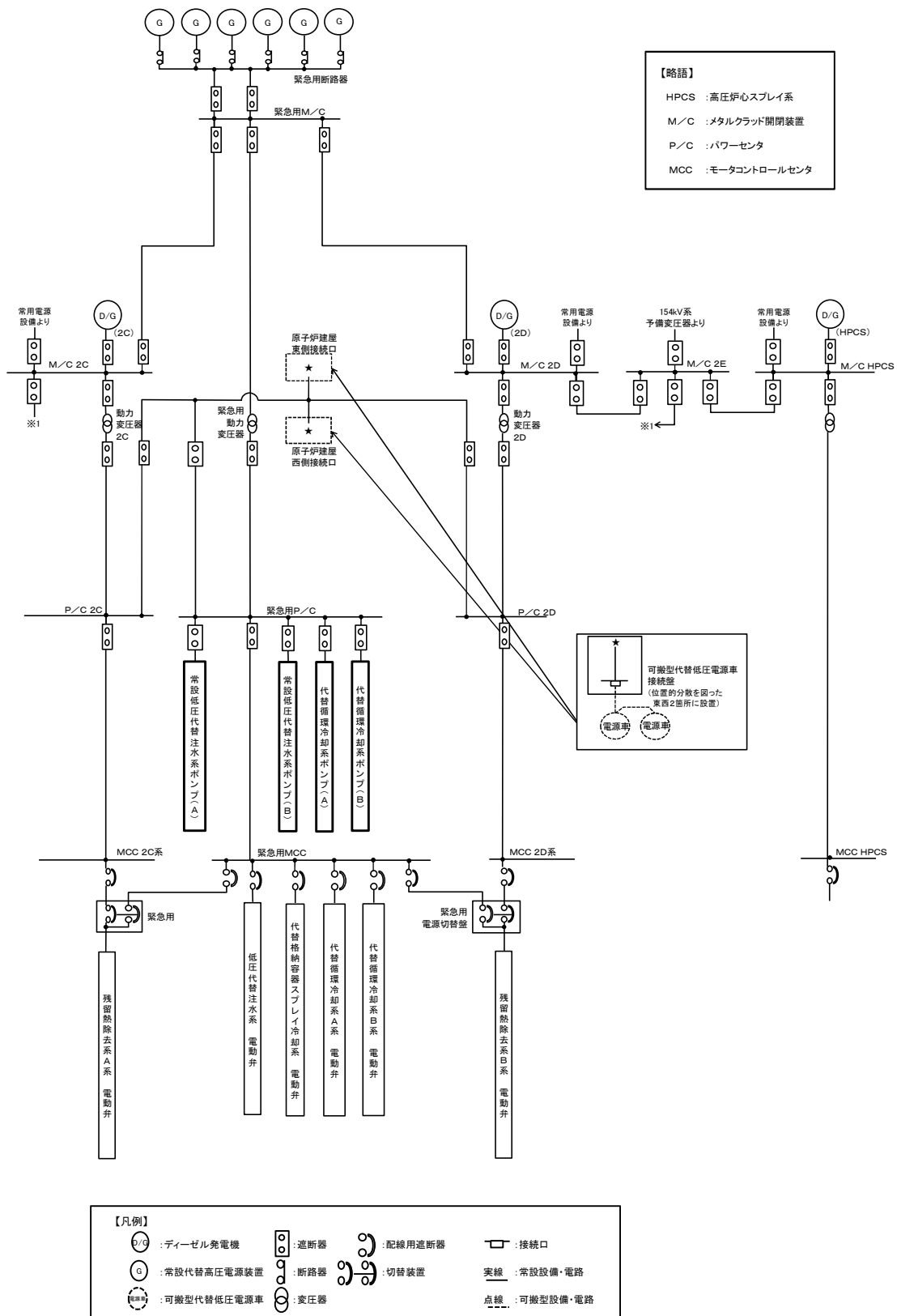
第 49-2-2 図 電源構成図 (交流電源) (2/2)
