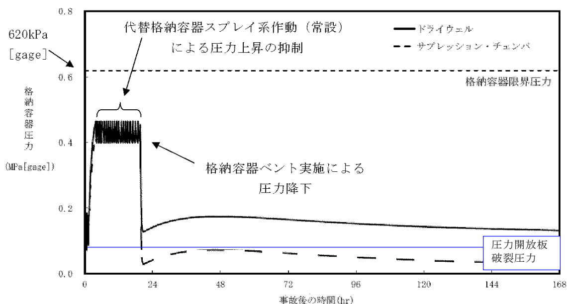
第 50-6-4 図 「雰囲気圧力・温度による静的負荷（格納容器過圧・過温破損）（代替循環冷却を使用しない場合）」における格納容器圧力の推移と圧力開放板破裂圧力との関係
