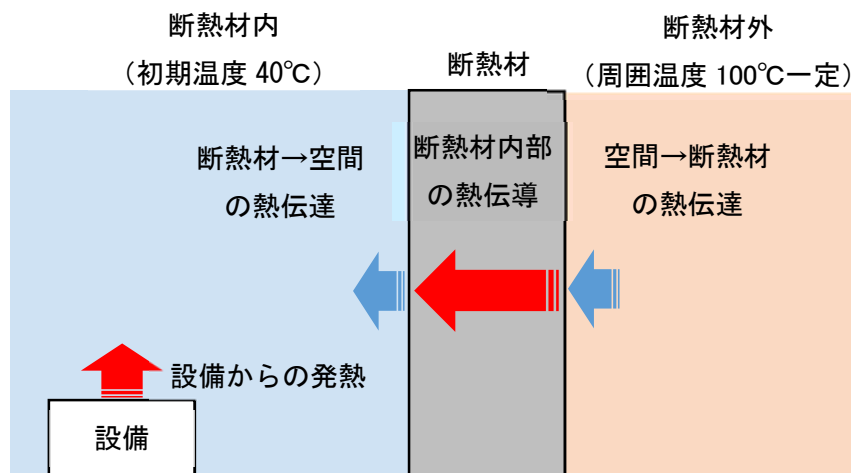
図1 断熱材厚さの評価モデルの概念図
