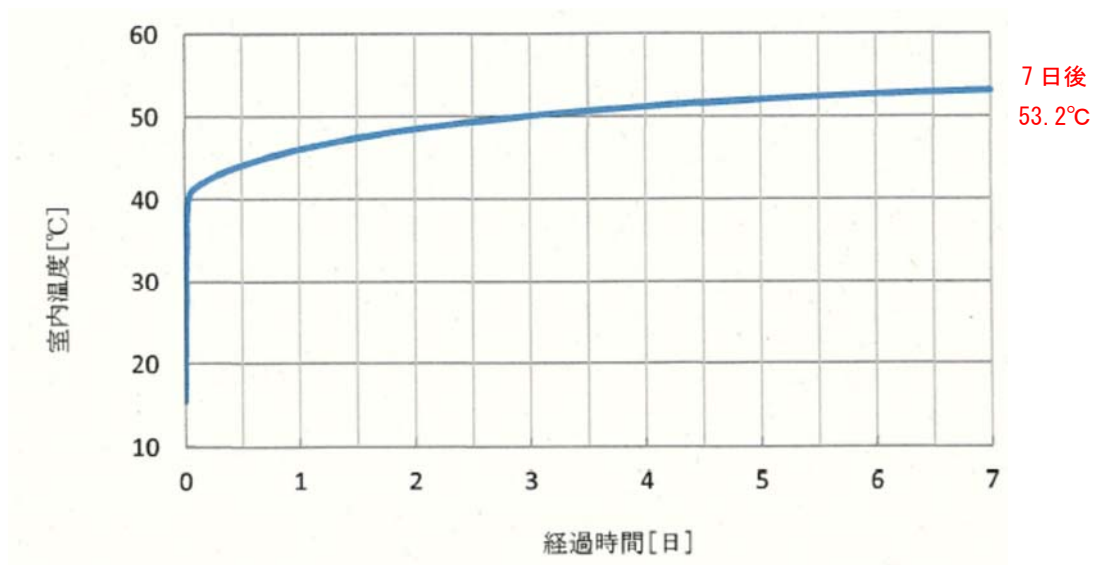
図3 格納容器圧力逃がし装置格納槽の室温評価結果
