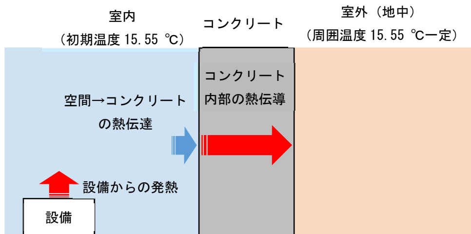
図2 室温評価の評価モデルの概念図
