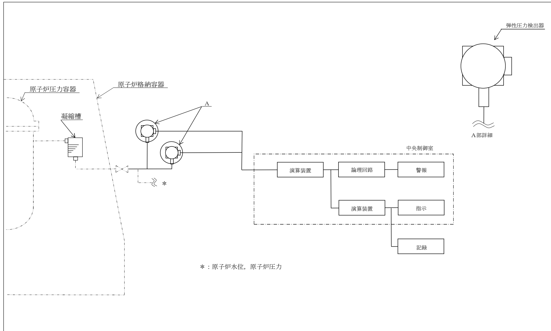
図 3-1-3-4 検出器の構造図 (原子炉压力 (S A))
