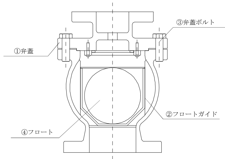
図 3-1 評価対象部位
