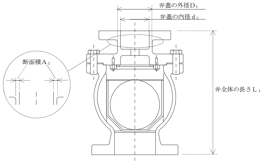
図 3-3 弁蓋の強度評価に用いる弁全体の長さ，弁蓋の外径及び内径
