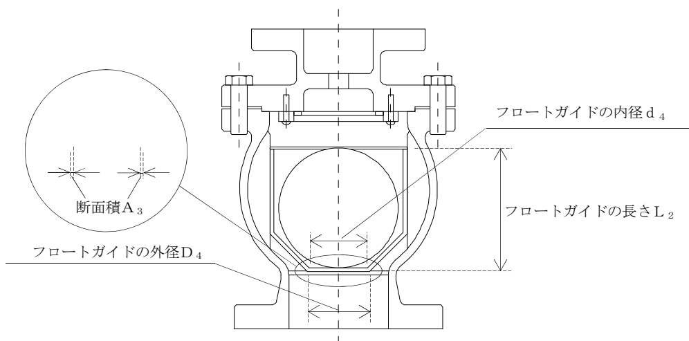
図 3-4 フロートガイドの強度評価に用いるフロートガイドの長さ、 フロートガイドの外径及び内径
