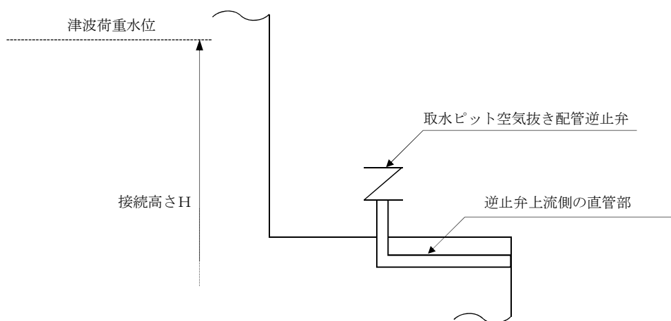
図 3-2 取水ピット空気抜き配管逆止弁の動水圧の算出に用いる H の設定
