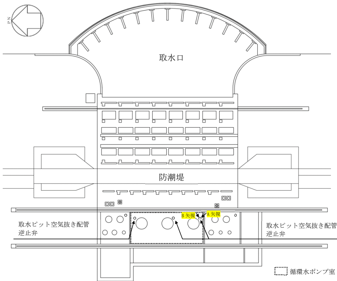
(平面図)
