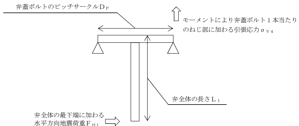
図 3-5 モーメントによる引張力の作用イメージ
