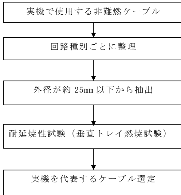
第 2-1 図 実機を代表するケーブル選定フロー
