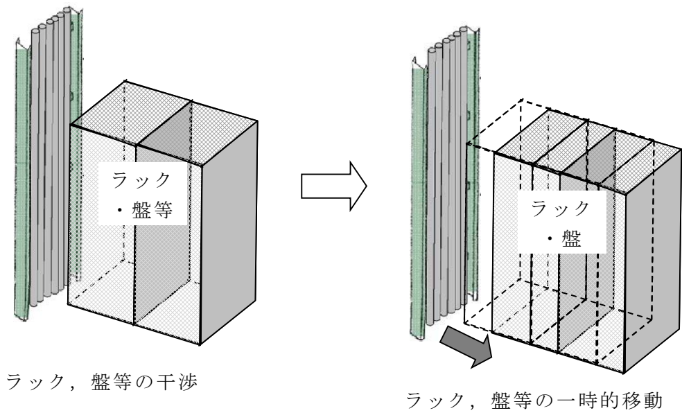
第 8.2-4 図 干渉物移動による作業
