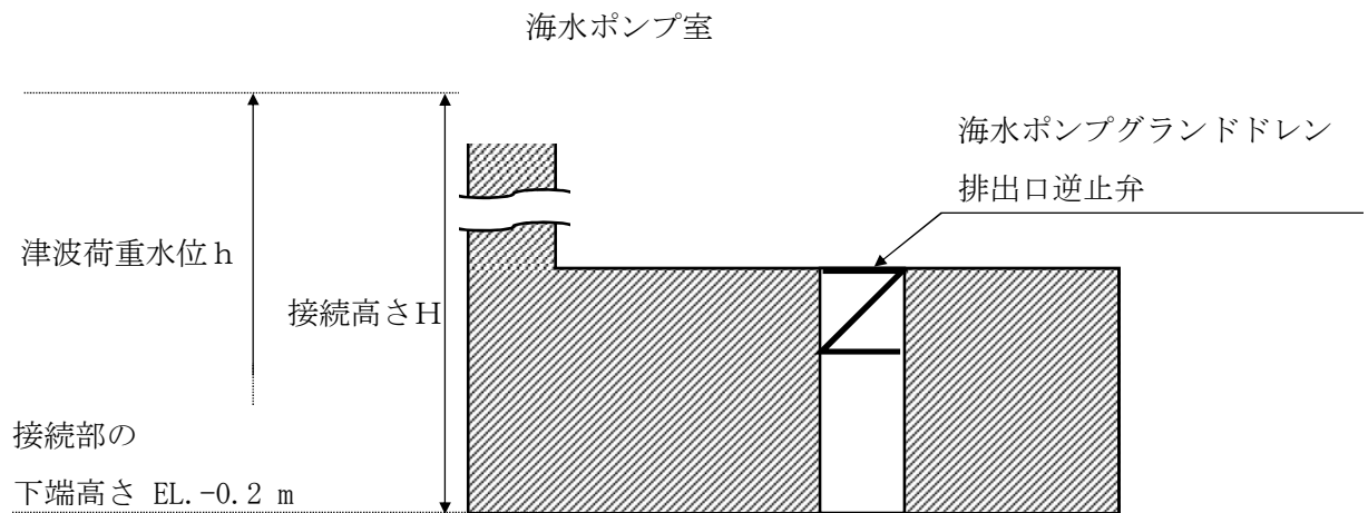
図 3-2 海水ポンプグラントドレン排出口逆止弁の動水圧の算出に用いる H の設定
