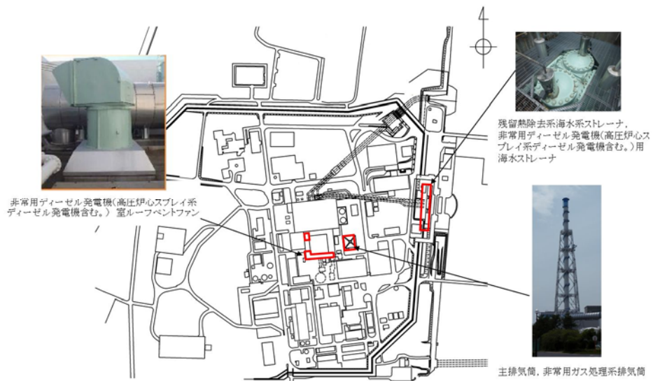
図 1-4 他の評価に包絡される対象の位置
