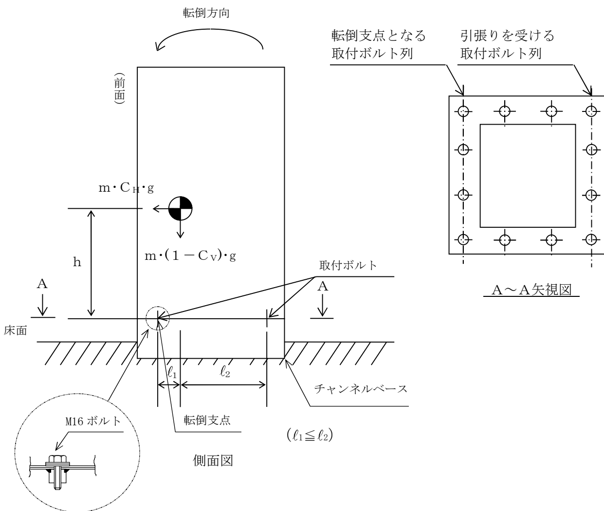
図2-1 計算モデル (垂直自立形 短辺方向転倒 (1 - C_V) \geq 0 の場合)
