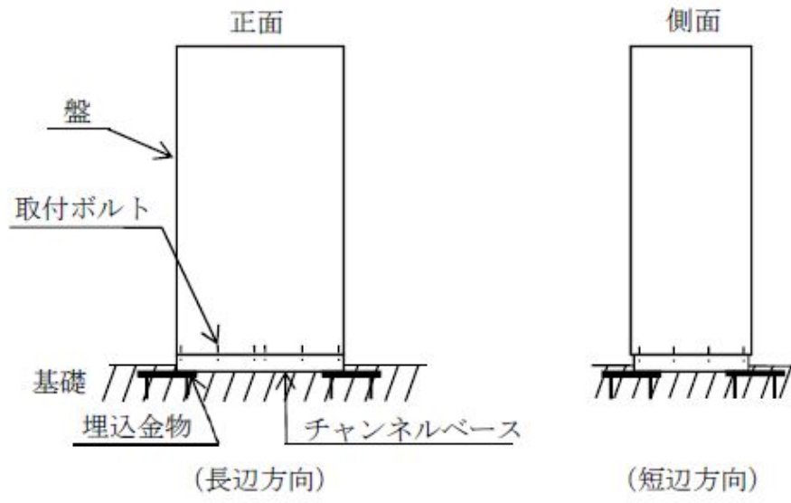
図1-2 概要図 (垂直自立形, 埋込金物)
