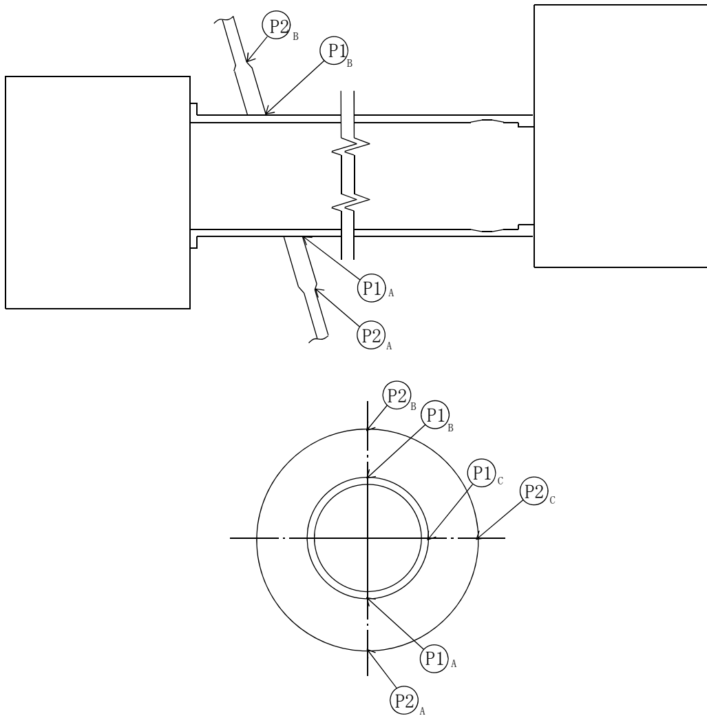
図 5-1 応力評価点
